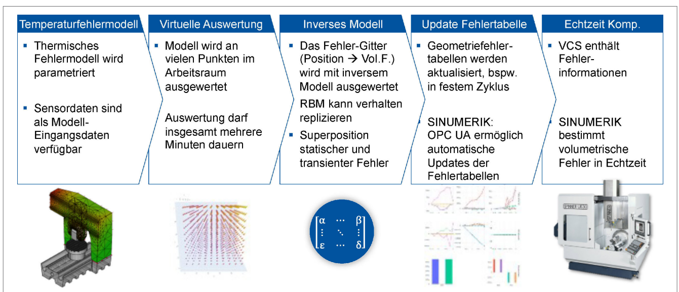
Bild 3 Arbeitsablauf: Überführung transients (thermischer) Fehler in ein Echtzeit-Starrkörpermodell (hier getestet mit: Siemens Sinumerik und VCS) auf einer Werkzeugmaschine. Grafik: WZL-IQS | RWTH Aachen
