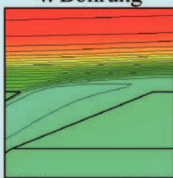
Bild 4b: Ergebnisse des Sonderforschungsbereichs 561 im Bereich Modellierung der aerothermomechanischen Phänomene.
