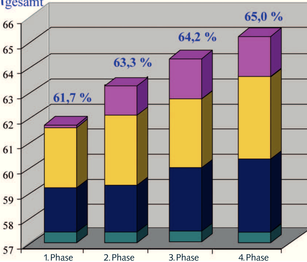
Bild 5: Beitrag der Technologien zur Entwicklung des Kraftwerk-Gesamtwirkungsgrades.
