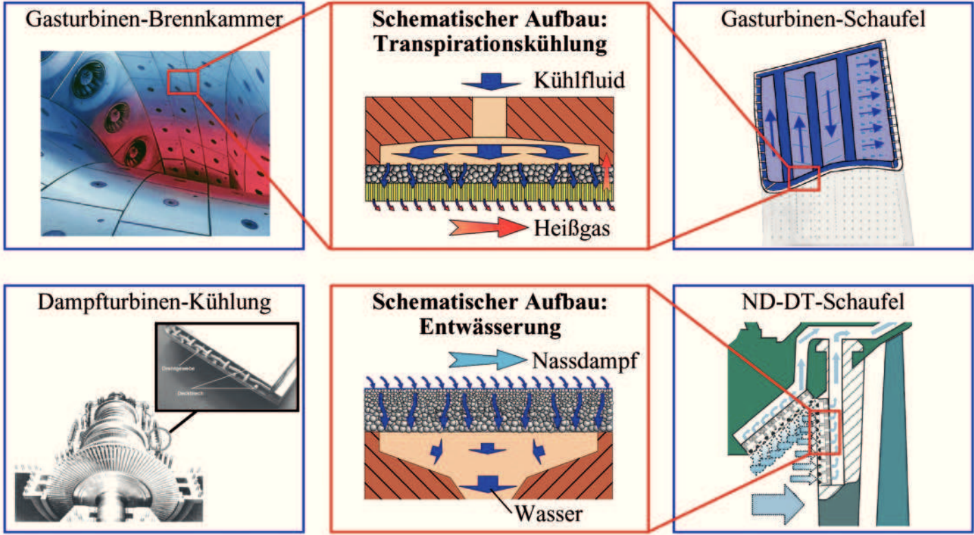
Bild 3: Wissenschaftliche Reduzierung der technologischen Herausforderungen auf Modelle.
