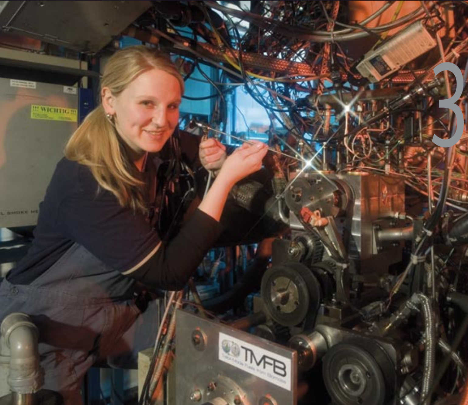
Versuchsstand des Exzellenzclusters „Maßgeschneiderte Kraftstoffe aus Biomasse“. Foto: Peter Winandy
