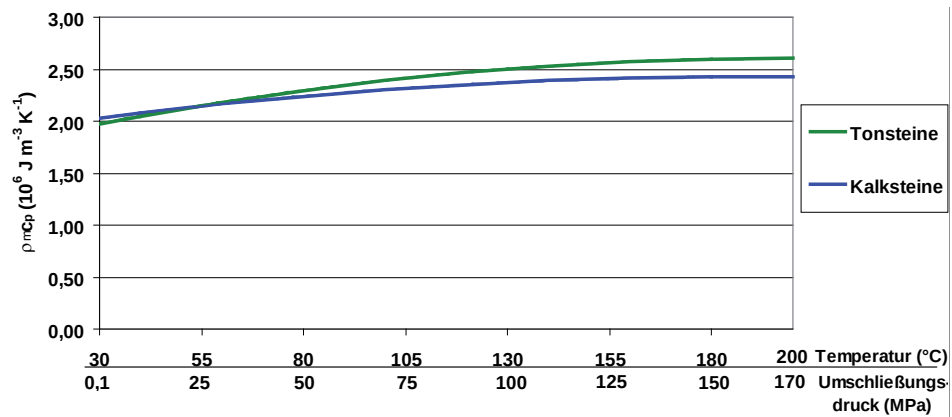
Abbildung 4.33: Mittlere Druck- und Temperaturabhängigkeit der volumetrische Wärmekapazität nach Gleichung 4.11 für die Hauptgesteinsarten.
