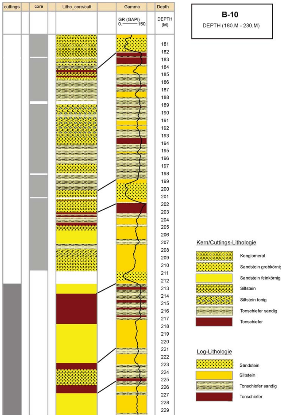
Abbildung 4.50: Lithologische Gliederung der Bohrung B-10 im Teufenintervall: 180 m bis 230 m. Bedeutung der Spalten von links nach rechts: 1. Bohrklingewinn; 2. Kerngewinn; 3. lithologische Unterteilung nach Kernbeschreibung und Bohrkleinanalyse; 3. Interpretation aus dem Gamma-Ray-Log, 4. Teufe. Insbesondere einzelne Sequenzen von Grobsand und Tonschiefer lassen sich zwischen den beiden Lithosäulen in Verbindung bringen.
