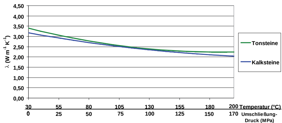
Abbildung 4.31: Mittlere Druck- und Temperaturabhängigkeit der Wärmeleitfähigkeit nach Gleichung 4.11 für die Hauptgesteinsarten.
