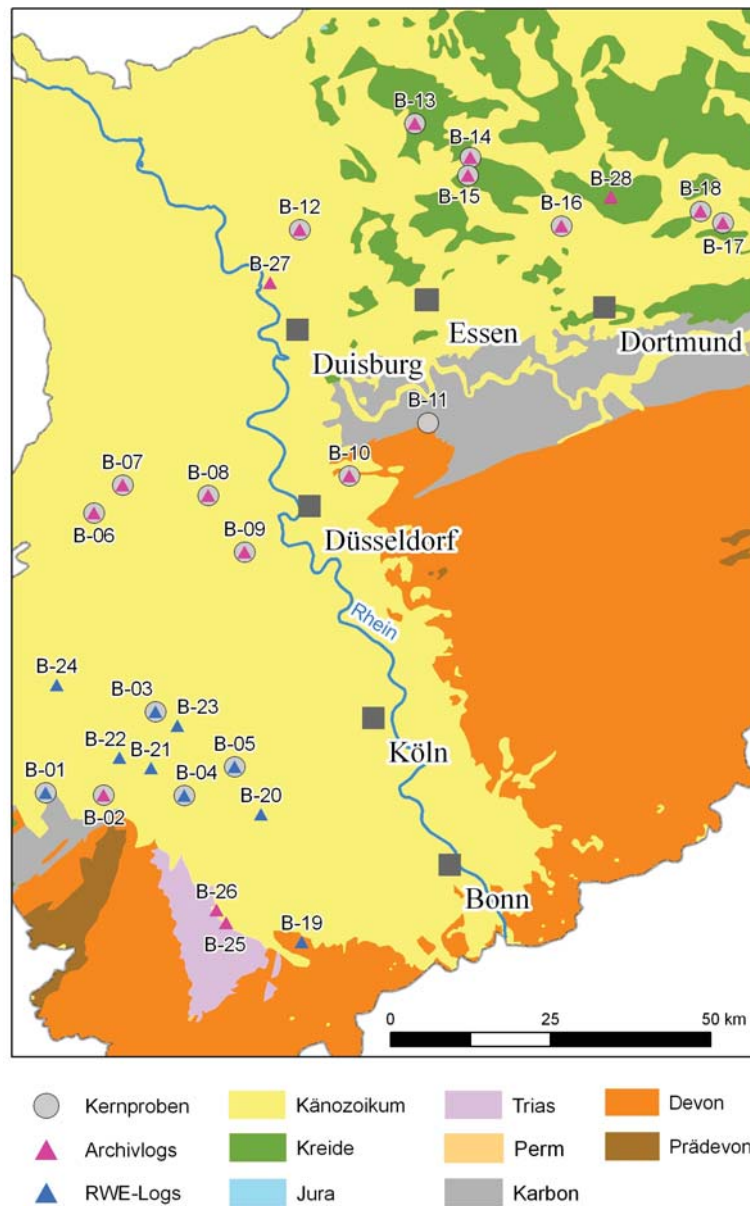
Abbildung 4.4: Übersicht der Bohrlochlokalitionen im westlichen Nordrhein-Westfalen, aus denen Kernproben und Bohrlochdaten zur Verfügung gestellt wurden.
