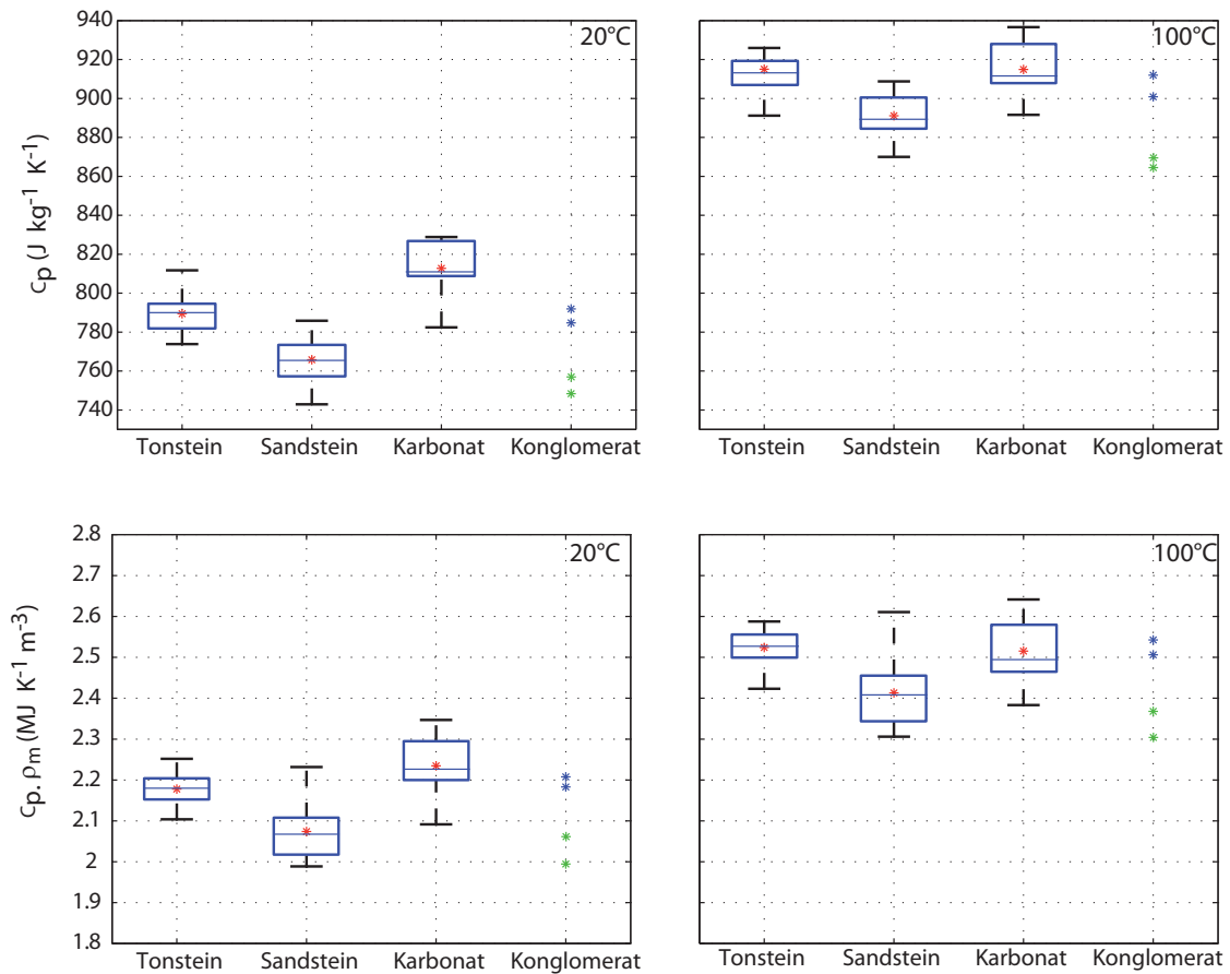
Abbildung 4.18: Häufigkeitsverteilung der spezifischen ( c_p ; oben) und volumetrischen Wärmekapazität ( \rho_m \cdot c_p ; unten) bei 20 °C (links) und bei 100 °C (rechts) für vier Hauptgesteinstypen und die dazugehörigen statistischen Maßzahlen in Form von Box-Whisker-Diagrammen (blaue Mittellinie: Medianwert; roter Stern: Mittelwert; blaue Box: 25%- und 75%-Quartil; schwarze Begrenzungsstriche: 5%- und 95 %-Perzentil). Bei den Konglomeraten sind jeweils zwei Einzelergebnisse phyllitreicher (blaue Sternchen) und quarzreicher Konglomerate (grüne Sternchen) markiert (vgl. Text). Die dargestellten Werte korrespondieren mit Tabelle 4.9.
