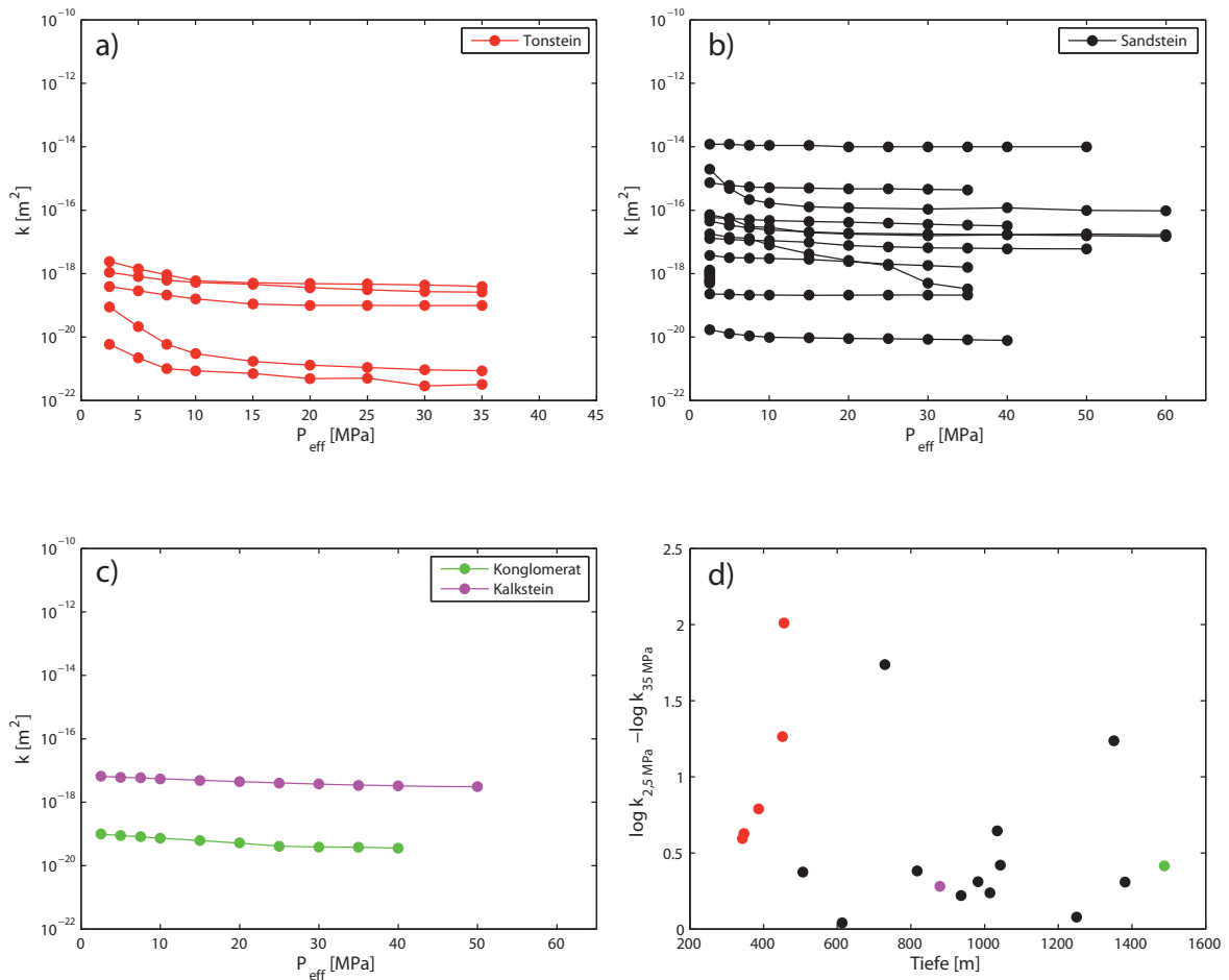
Abbildung 4.38: Permeabilität k ausgewählter Proben in Abhängigkeit des effektiven Drucks P_{eff} für verschiedene Gesteinstypen paläozoischer Gesteinsserien aus dem westlichen Nordrhein-Westfalen (a-c). d) Relative Abnahme der Permeabilität k (logarithmisch) als Differenz zwischen der logarithmischen Permeabilität bei P_{eff}=2,5 MPa und P_{eff}=35 MPa in Abhängigkeit der Tiefe, aus der die jeweiligen Proben ursprünglich stammen.
