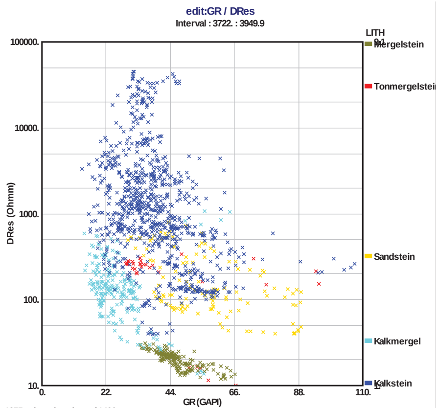
Abbildung 5.8: Streudiagramm des im Bohrloch gemessenen Widerstands ( DRes ) gegen die Gamma-Strahlung ( GR ). Dargestellt sind die Abfolgen des Kalksteins und des Gault-Sandsteins der Unterkreide sowie Schichten des Kalkmergelsteins, Mergelsteins und Tonmergelsteins aus dem Turon.
