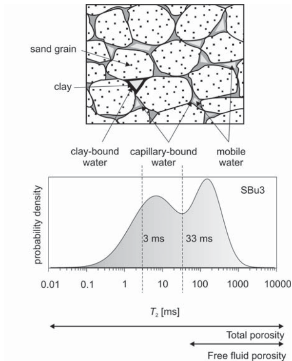
Abbildung 2.11: T_2 -Verteilung in einem wassergesättigten Sandstein zur Identifizierung von Fluidkomponenten (aus Arnold, 2007). Mobiles Wasser (hellgrau) verursacht größere T_2 -Werte, während die kleinere T_2 -Werte kapillar- und tongebundenes Wasser anzeigen (nach Allen et al., 2000).
