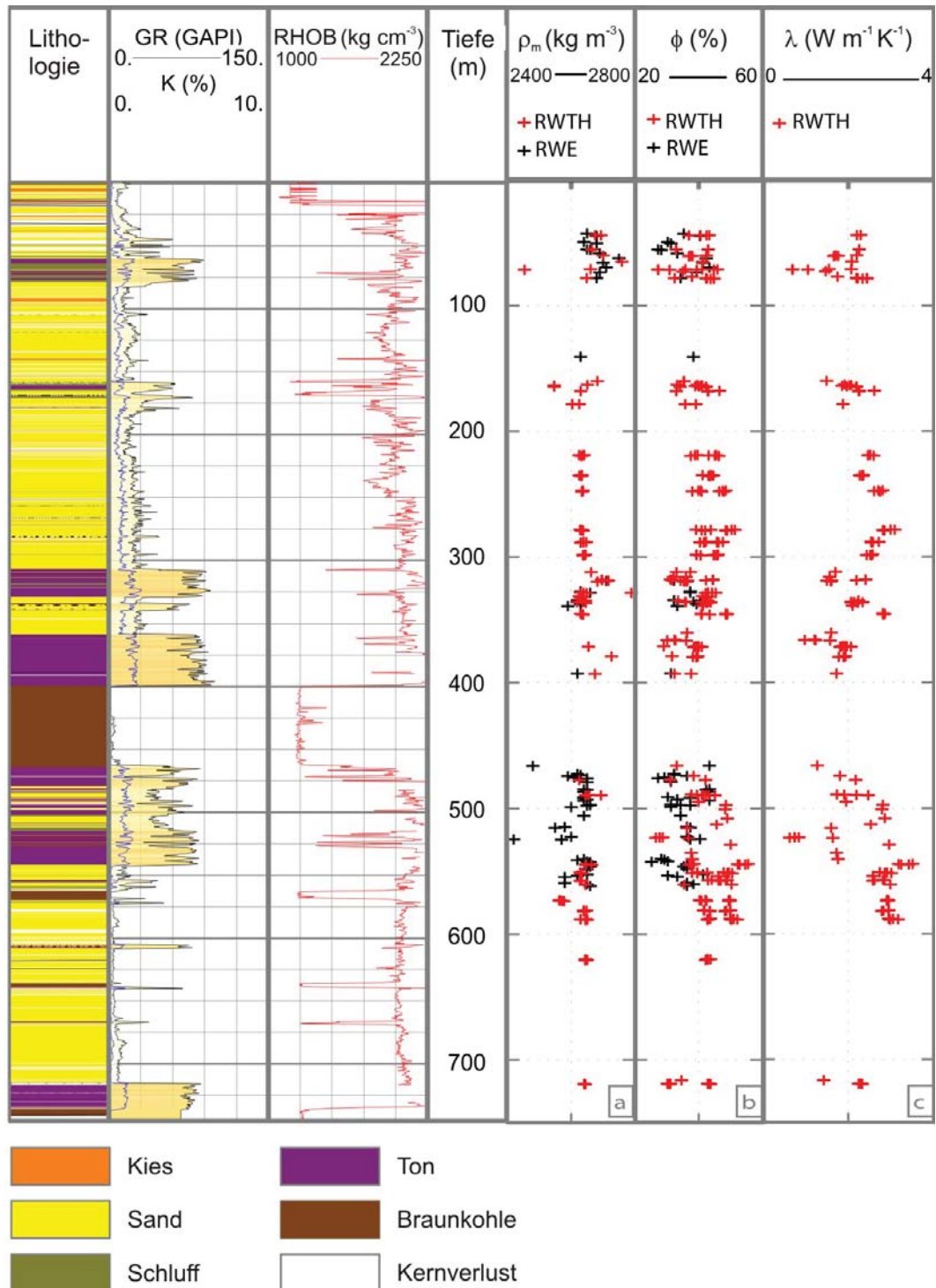
Abbildung 3.5: Lithologisches Profil, bohrlochphysikalische Messungen (GR: Gamma-Ray; RHOB: Dichte) und gesteinsphysikalische Laboruntersuchungen ( \rho_m : Reindichte; \phi : Porosität, \lambda_f : Wärmeleitfähigkeit im bergfeuchten Zustand). Reindichte und Porosität wurden mittels Stechzylinder bzw. einer Ausstechform in Anlehnung an DIN 18125-1 (1997) jeweils in den Laboren der RWTH Aachen (rot) und der RWE Power AG (schwarz) ermittelt.
