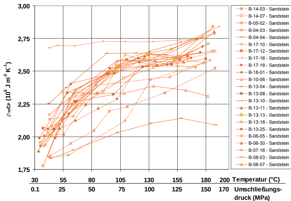
Abbildung 4.30: Ergebnisse der druck- und temperaturabhängigen Messungen der volumetrischen Wärmekapazität ( \rho_m c_p ) für die Sandsteine.
