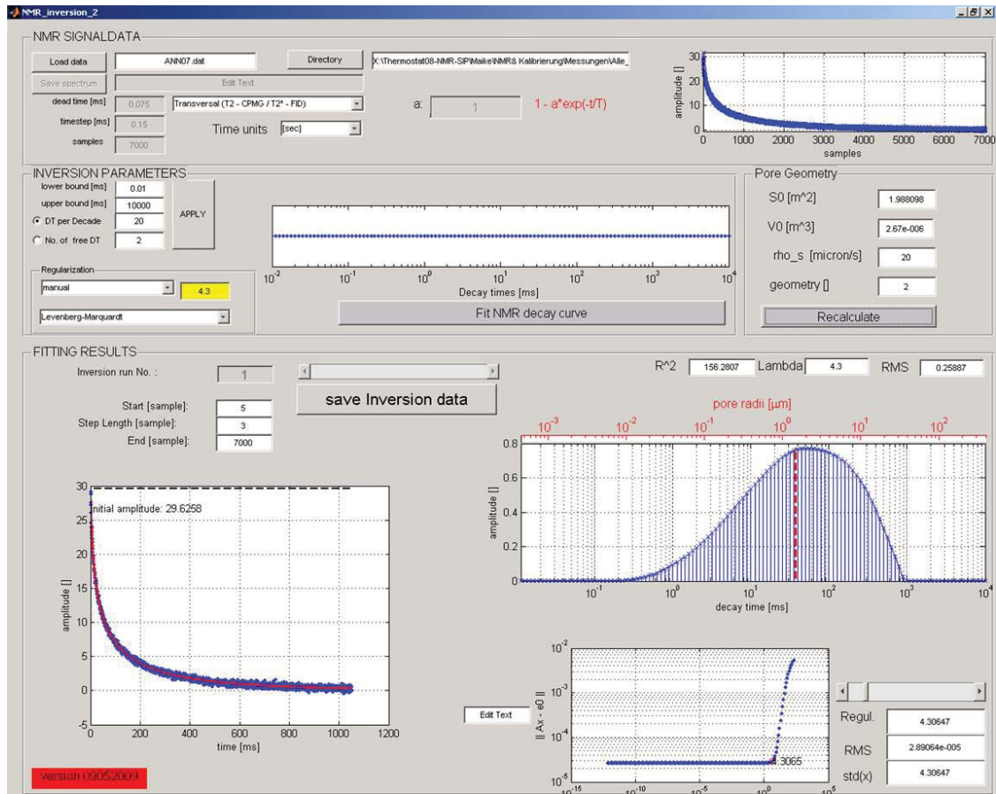
Abbildung 4.39: Benutzeroberfläche des MATLAB-Programms zur Auswertung von 1D- und 2D-NMR-Relaxometriedaten.
