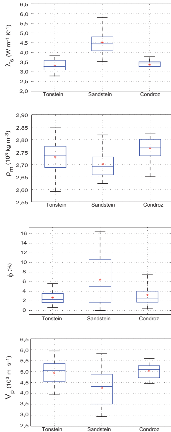
Abbildung 4.15: Darstellung der statistischen Maßzahlen petrophysikalischer Eigenschaften für drei modifizierte Gesteinsgruppen aus dem Paläozoikum des westlichen Nordrhein-Westfalens in Form von Box-Whisker-Diagrammen (blaue Mittellinie: Medianwert; roter Stern: Mittelwert; blaue Box: 25%- und 75%-Quartil; schwarze Begrenzungsstriche: 5%- und 95%-Perzentil): a) Wärmeleitfähigkeit gesättigter Proben \lambda_s , b) Reindichte \rho_m , c) Porosität \phi und d) Kompressionswellengeschwindigkeit V_p . Die dargestellten Werte korrespondieren mit Tabelle 4.7.
