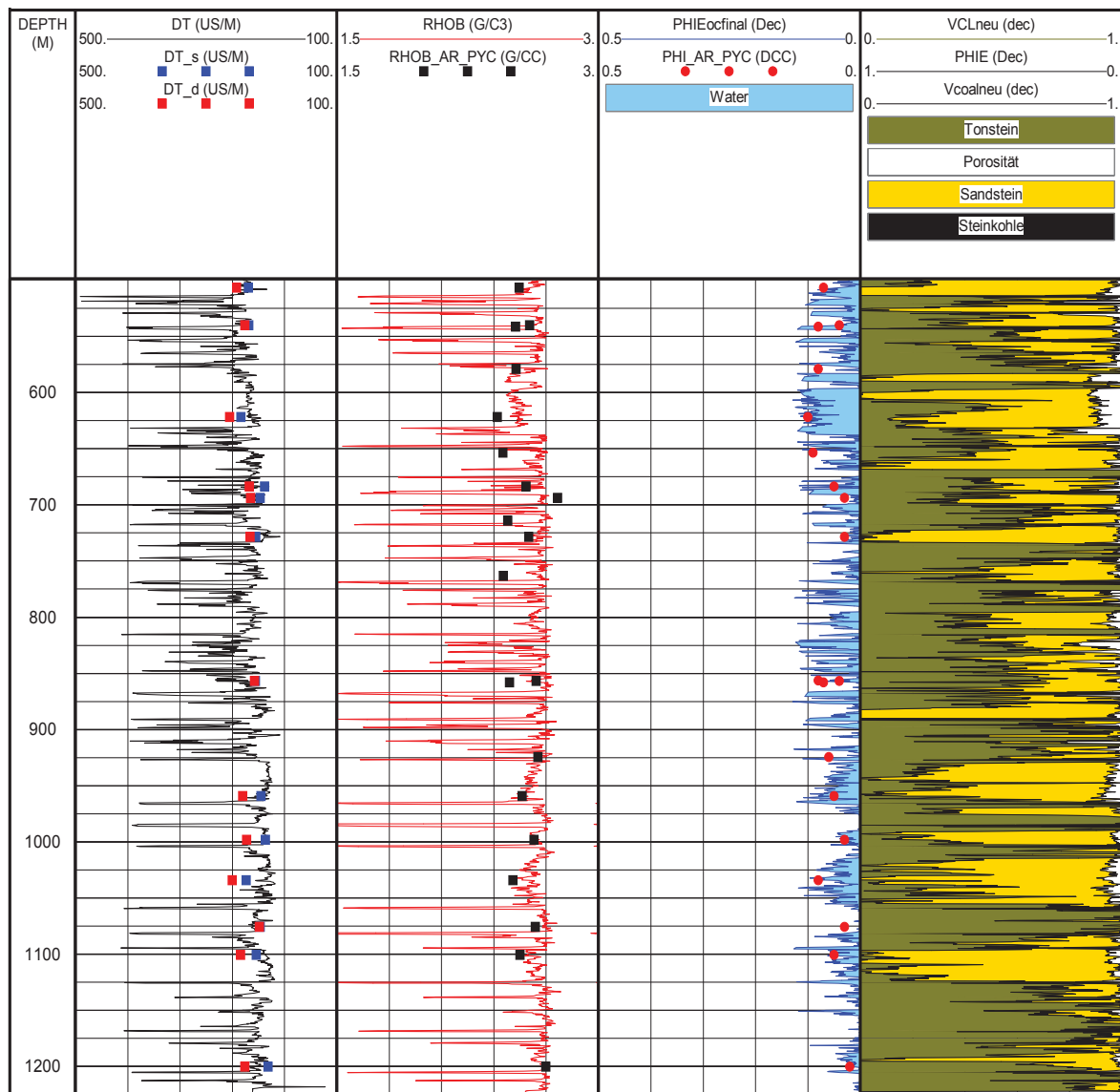
Abbildung 4.45: Vergleich der berechneten und am Kern gemessenen Porositätswerte für die Bohrung B-17 (PHIEocfinal, PHI_AR_PYC). Für die Berechnung der Porosität wurden Zonen, in denen Steinkohle auftritt, nicht berücksichtigt. Zusätzlich dargestellt sind die Logs der Dichte (RHOB) und P-Wellengeschwindigkeit (VP) mit den entsprechenden Kernmessungen: RHOB_AR_PYC, DT_s (saturiert), DT_d (trocken).
