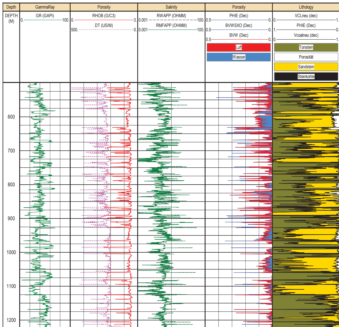
Abbildung 4.44: Ergebnis der petrophysikalischen Auswertung für die Bohrung B-17. GR: Gammaaktivität; RHOB: Gesamtdichte; DT: Laufzeit der Longitudinalwelle; RWAPP: scheinbarer Widerstand des Formationswassers; RMFAPP: scheinbarer Widerstand des Mud-Filtrats; PHIE: effektive Porosität; BVW: Gesamtwasservolumen; BVWSXO: Gesamtwasservolumen der saturierten Formation; VCLneu: Tonvolumen, berechnet aus GR; Vcoalneu: ausgewiesen durch Dichte-Cuttoff.
