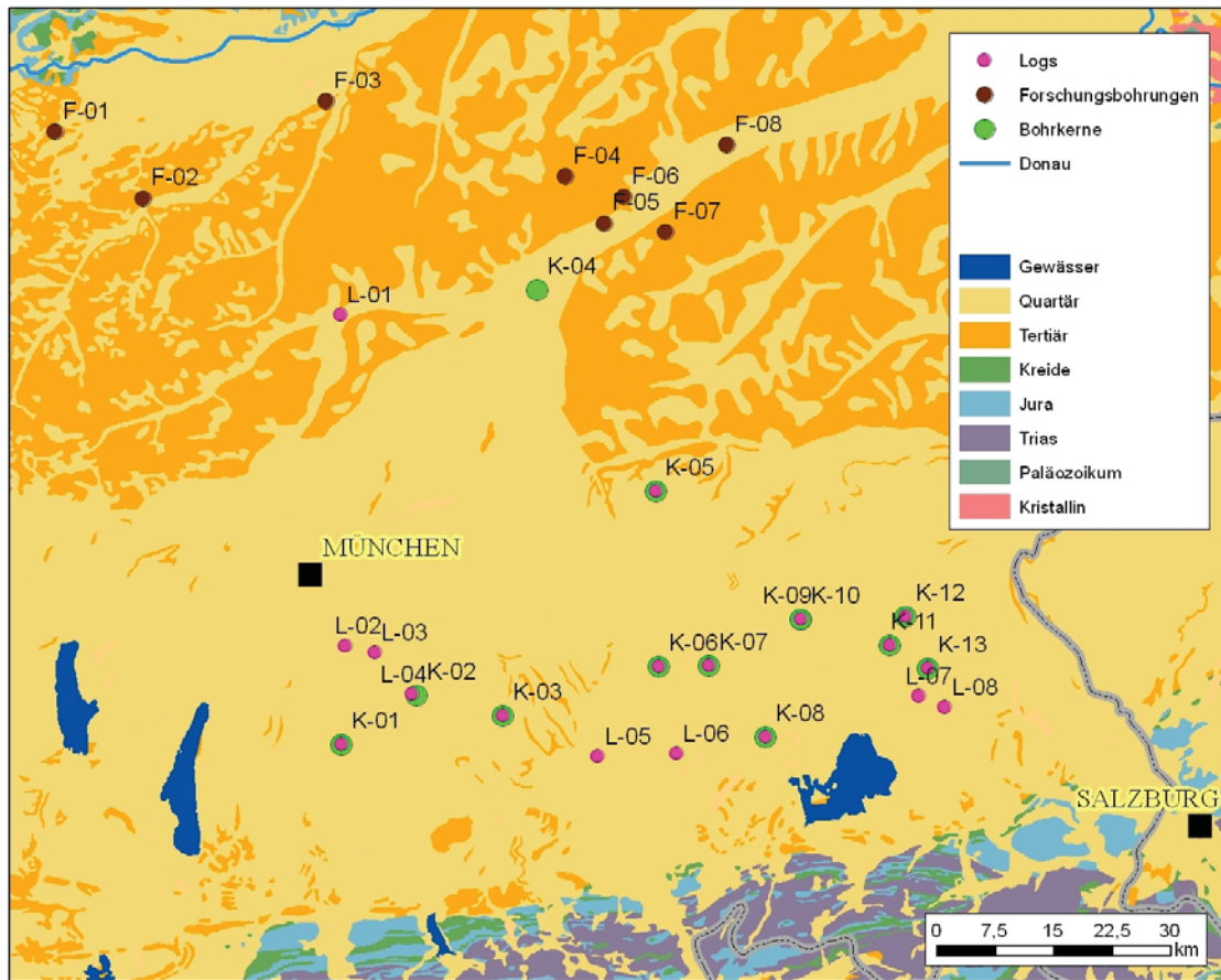
Abbildung 5.3: Übersicht der Bohrlochlokalitionen in der Ostmolasse, aus denen Kernproben (grüne Punkte; vgl. Tabelle 5.1) oder Logdaten (vgl. Tabelle 5.4) aus Forschungsbohrungen (braune Punkte) und Explorationsbohrungen der KW-Industrie (rosafarbene Punkte) dem Forschungsprojekt zur Verfügung gestellt wurden.
