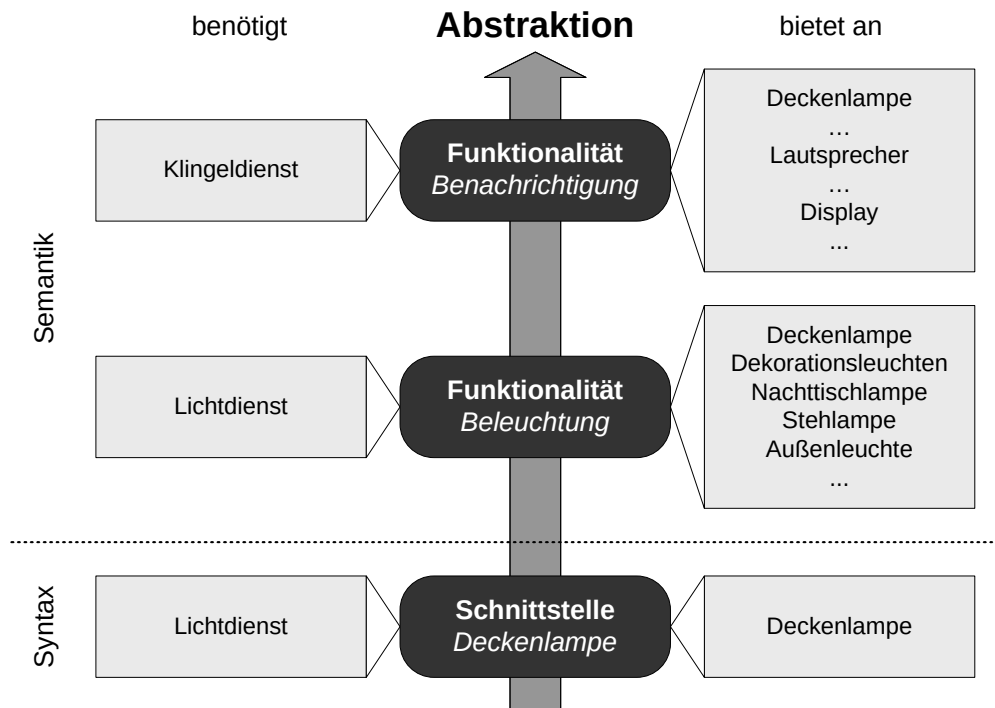
Abbildung 5.4: Abstraktionsebenen der semantischen Modellierung.
