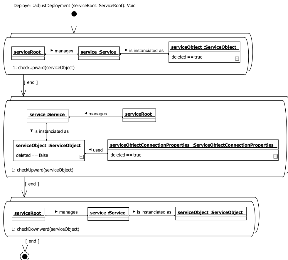
Abbildung 4.31: Anpassung des Deployments.
