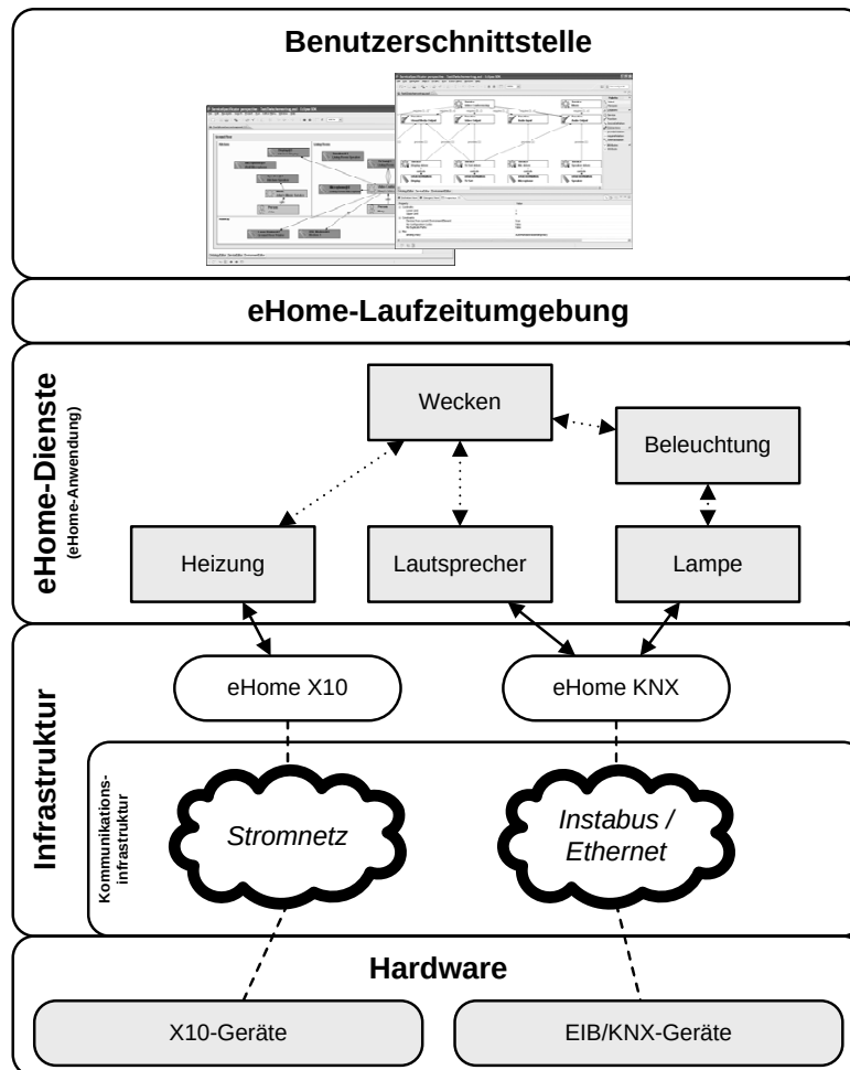
Abbildung 6.1: Übersicht des realisierten Systems.
