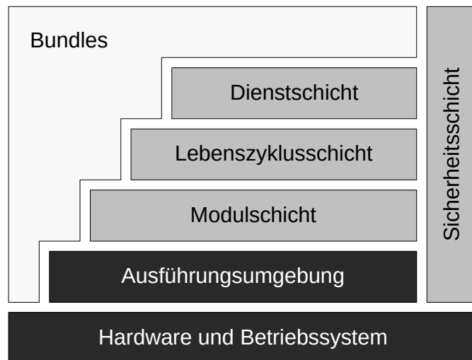
Abbildung 3.2: Aufbau der OSGi Service Plattform. (in Anlehnung an [OSG07b])
