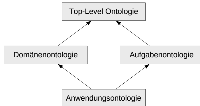
Abbildung 5.3: Arten von Ontologien nach ihrem Grad an Allgemeinheit. (in Anlehnung an [Gua98])
