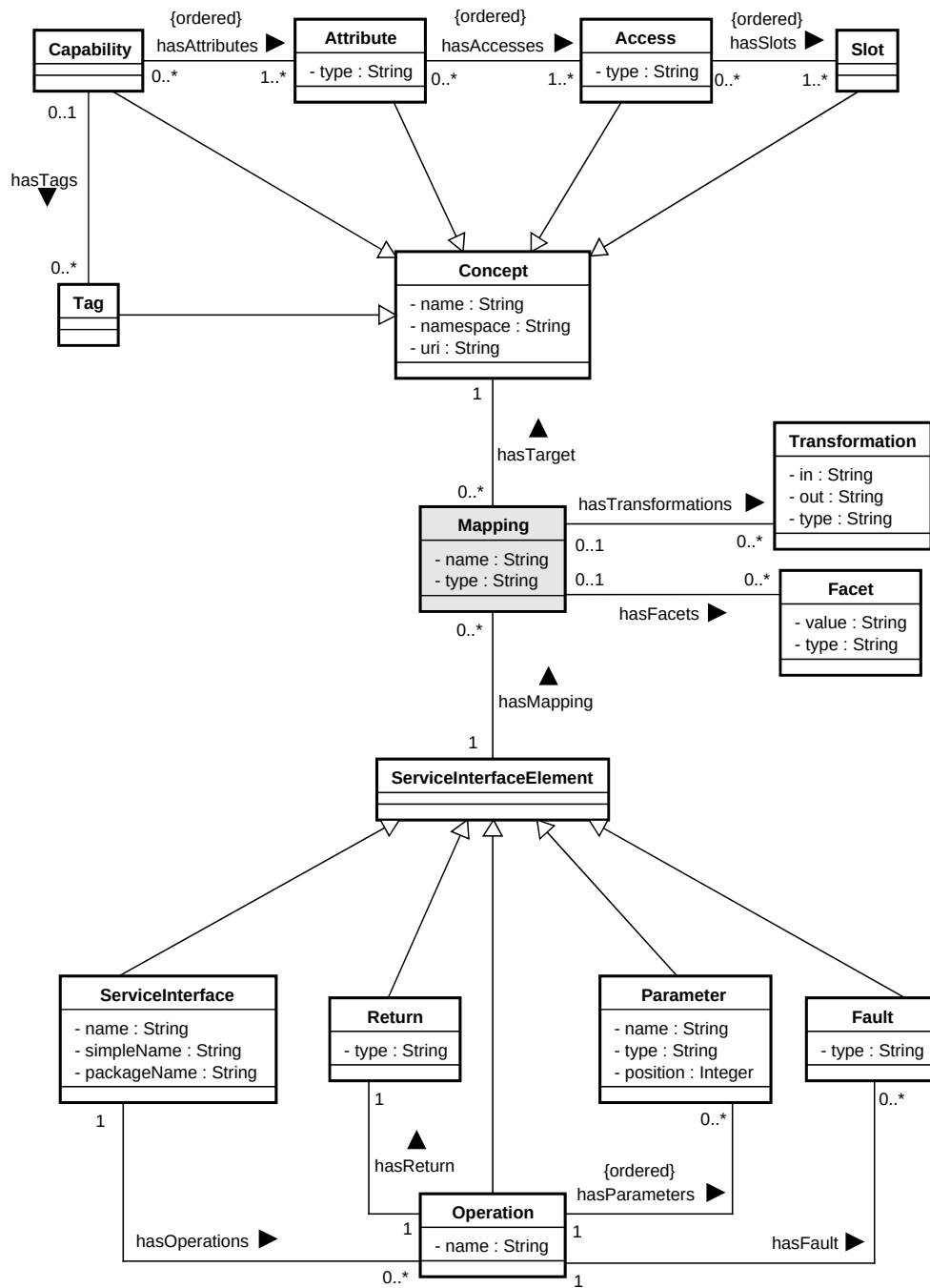
Abbildung 5.15: Modellierung der semantischen Abbildung.
