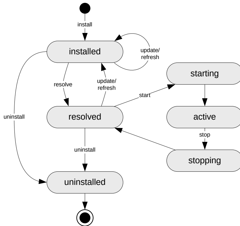
Abbildung 3.3: Lebenszyklus eines OSGi Bundles.
