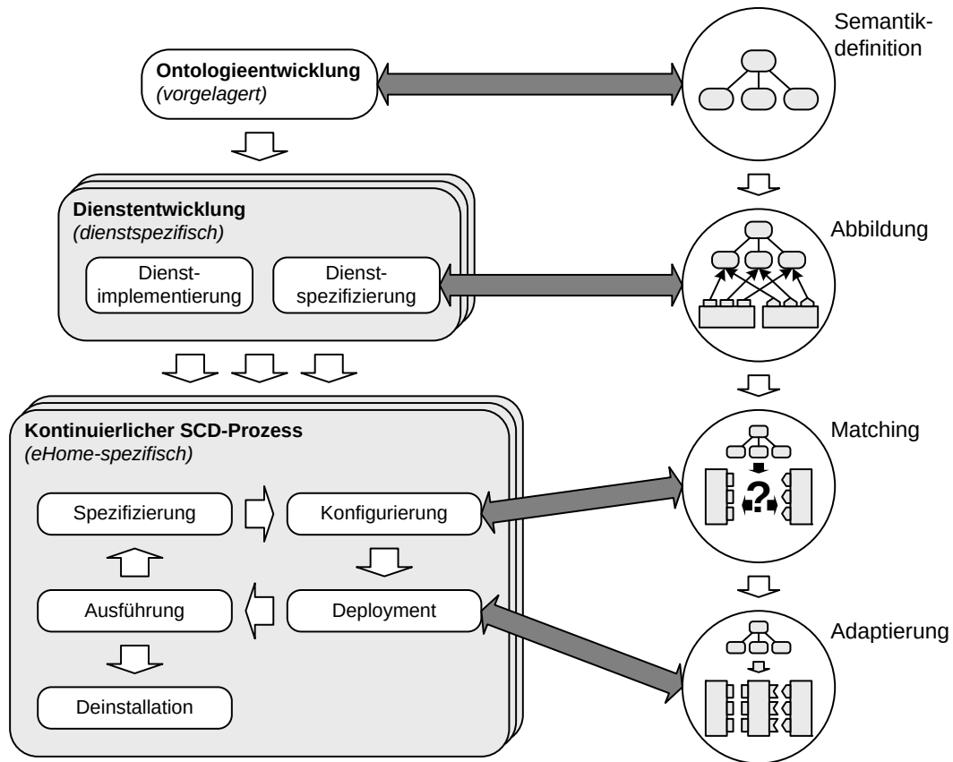
Abbildung 5.8: Einbettung des semantischen Teilprozesses in den Entwicklungsprozess für dynamische eHome-Systeme.
