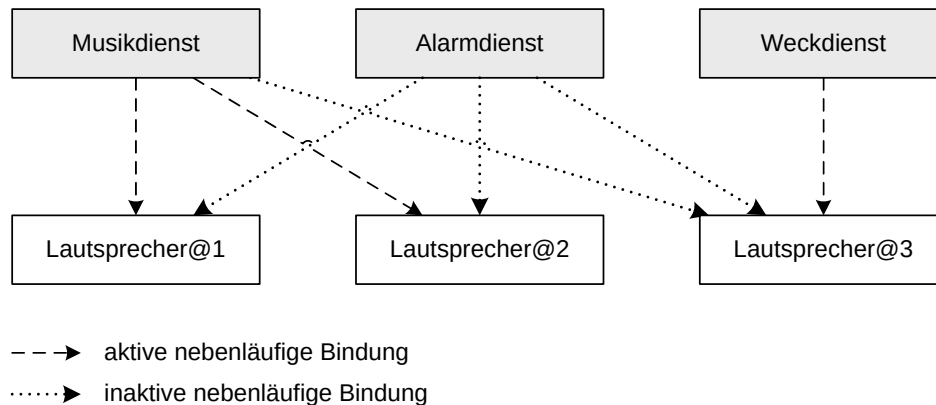
Abbildung 4.14: Beispielkonfiguration mit nebenläufigen Bindungen.
