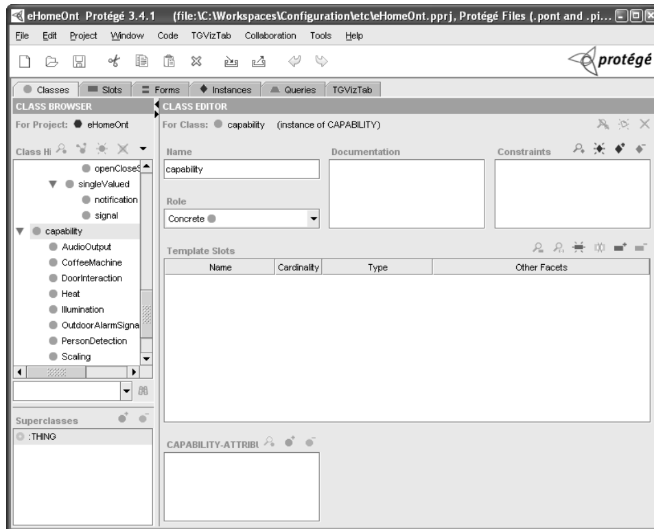
Abbildung 5.14: Protégé-Editor mit eHome-Ontologie.
