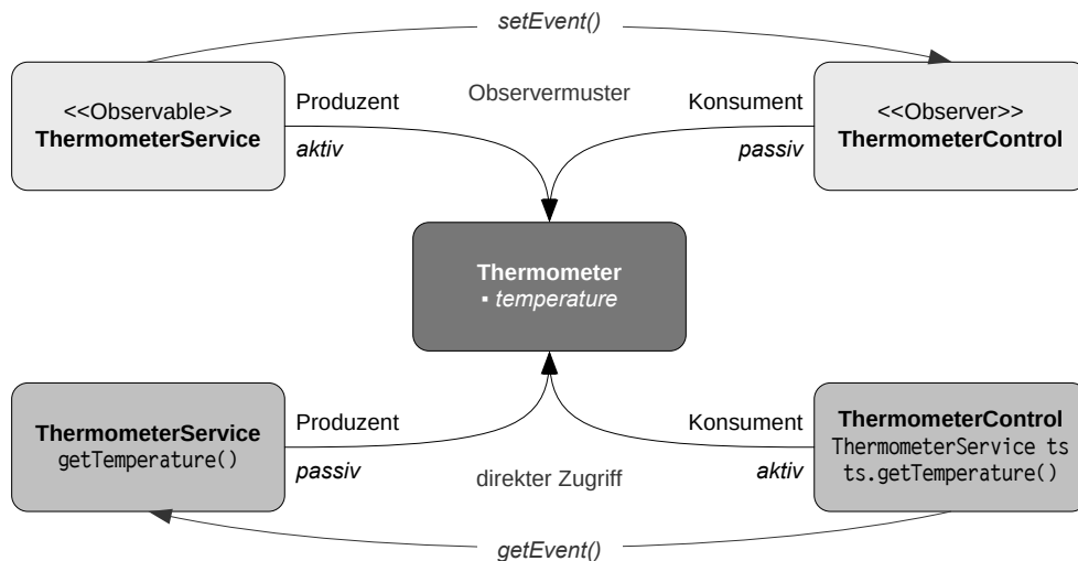
Abbildung 5.20: Adaption aktiver und passiver Komponenten.
