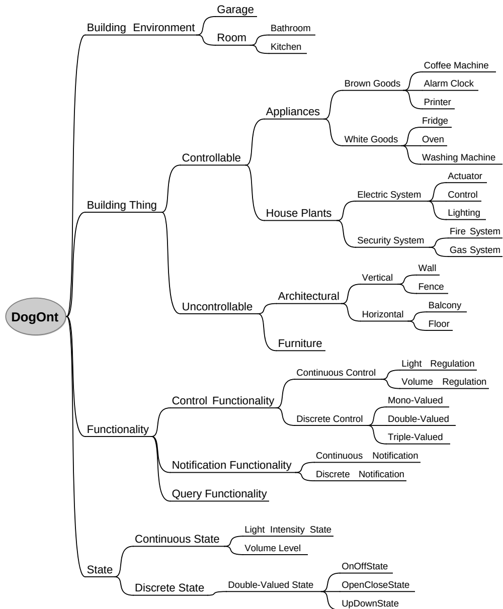
Abbildung 5.23: Ausschnitt der DogOnt-Ontologie. (in Anlehnung an [BC08])
