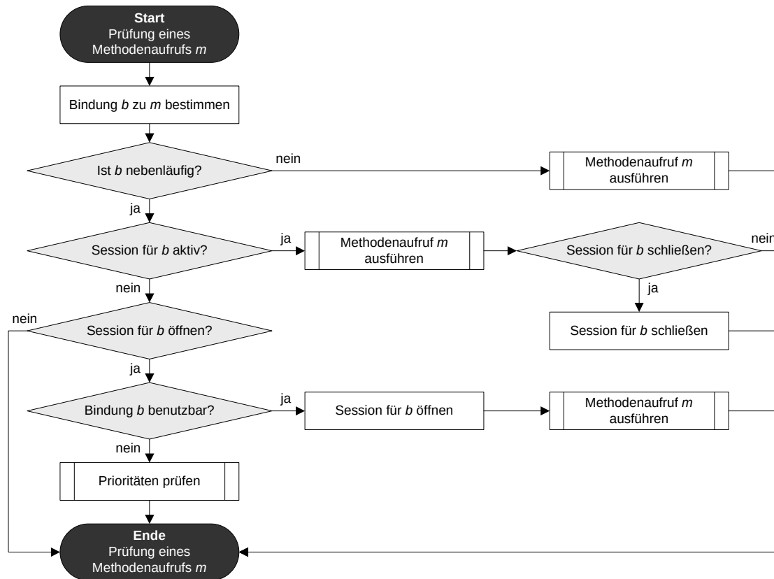
Abbildung 4.33: Algorithmus zur Prüfung eines Methodenaufrufs bei der Dienstkommunikation.
