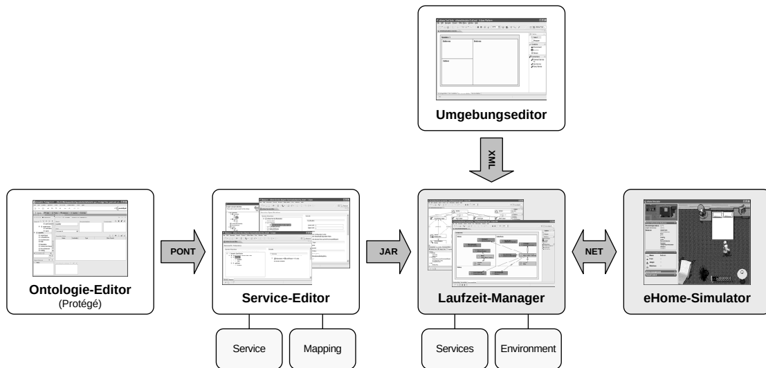
Abbildung 6.3: Zusammenspiel der entwickelten Werkzeuge.
