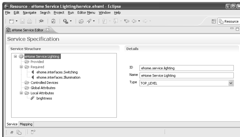
Abbildung 6.4: Bearbeiten einer Dienstspezifikation im Service-Editor.
