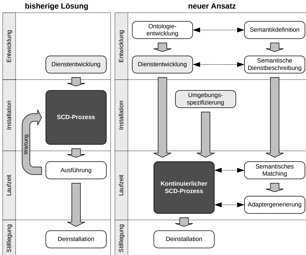
Abbildung 1.2: Übersicht des neuen Ansatzes.
