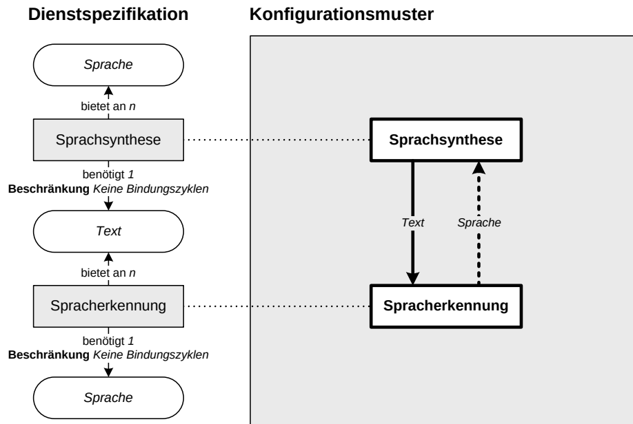
Abbildung 4.10: Beispiel einer Bindungsbeschränkung gegen Konfigurationszyklen.
