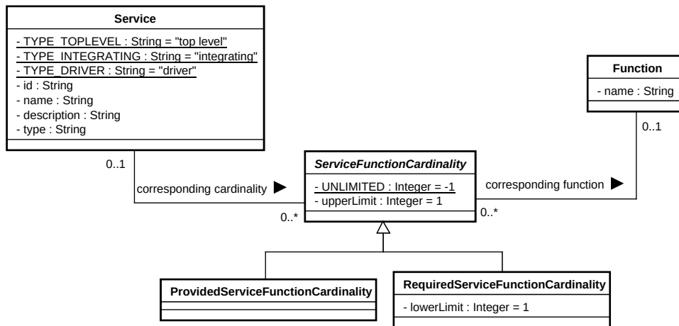
Abbildung 4.3: Modellierung der Dienstspezifikation.
