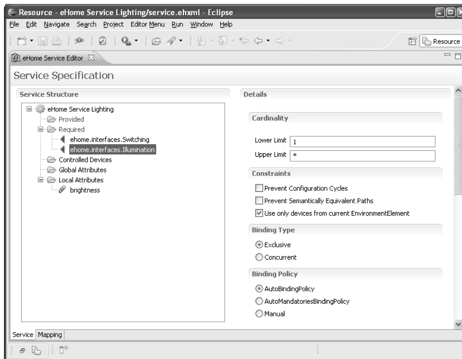
Abbildung 6.6: Spezifikation einer benötigten Funktionalität.
