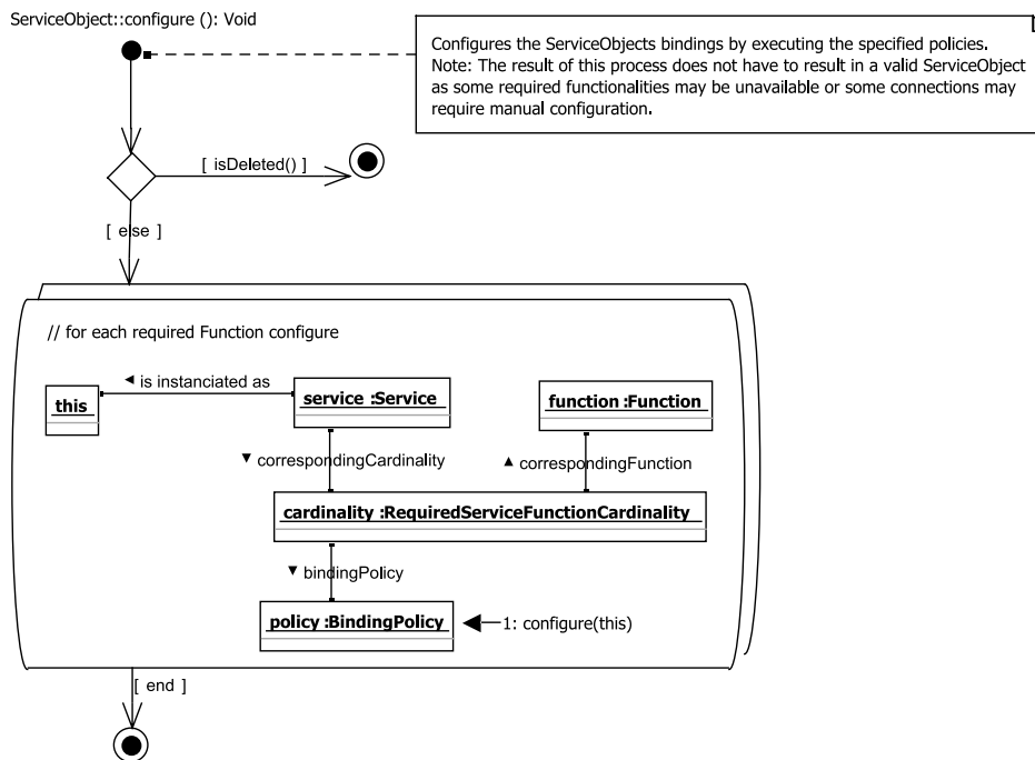
Abbildung 4.21: Konfigurierung eines ServiceObject.
