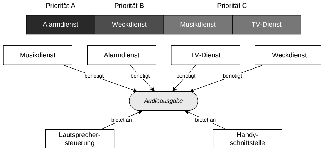
Abbildung 4.15: Beispiel der Priorisierung auf Basis von Funktionalitäten.
