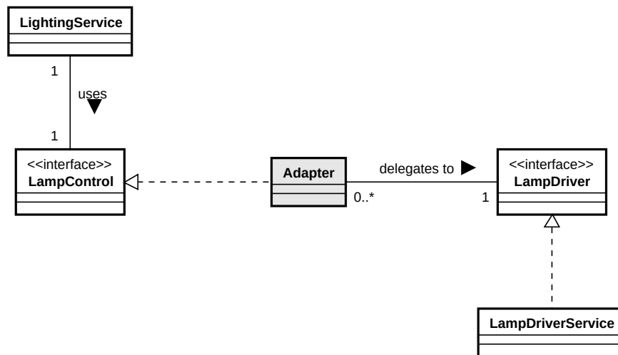
Abbildung 5.21: Struktur des Adaptermusters.
