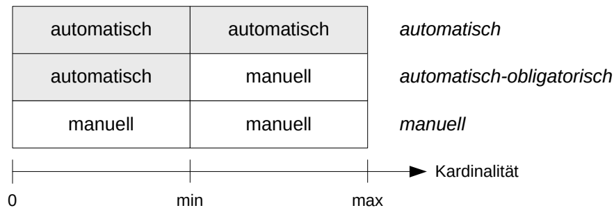
Abbildung 4.12: Festlegung des Bindungsverhaltens.
