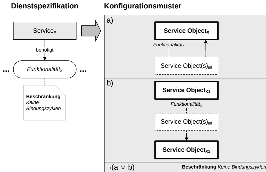
Abbildung 4.9: Bindungsbeschränkung zum Verhindern zyklischer Bindungen.
