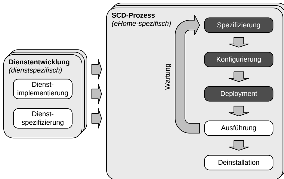
Abbildung 3.7: Entwicklungsprozess für eHome-Systeme nach NORBISRATH mit eingebettetem SCD-Prozess. (in Anlehnung an [Nor07])
