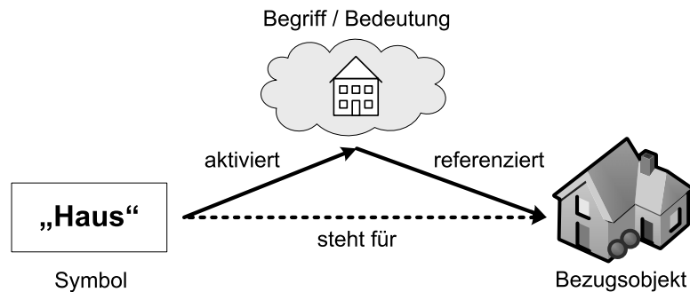
Abbildung 5.1: Semiotisches Dreieck.
