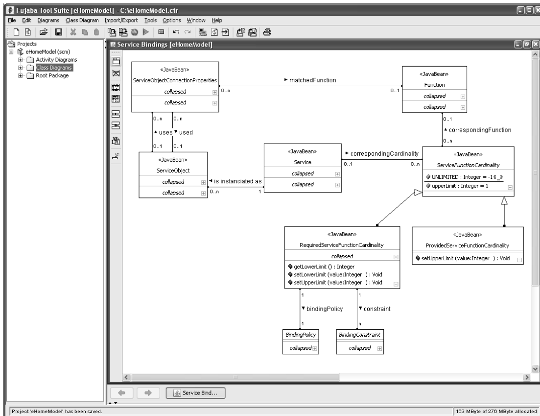
Abbildung 3.5: Die Fujaba-Entwicklungsumgebung.
