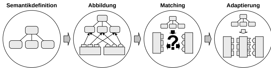
Abbildung 5.7: Semantischer Teilprozess.
