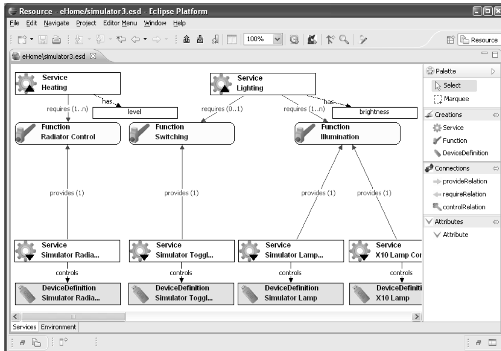
Abbildung 6.10: Dienstübersicht im Laufzeit-Manager.
