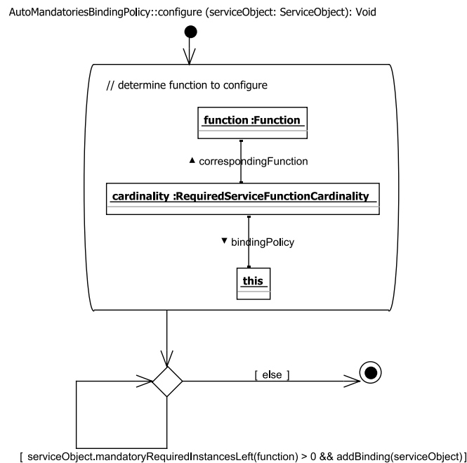
Abbildung 4.22: Konfigurierung mit automatisch-obligatorischer Bindungsstrategie.
