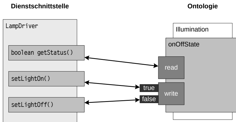
Abbildung 5.16: Beispiel einer Funktionalitätsabbildung.
