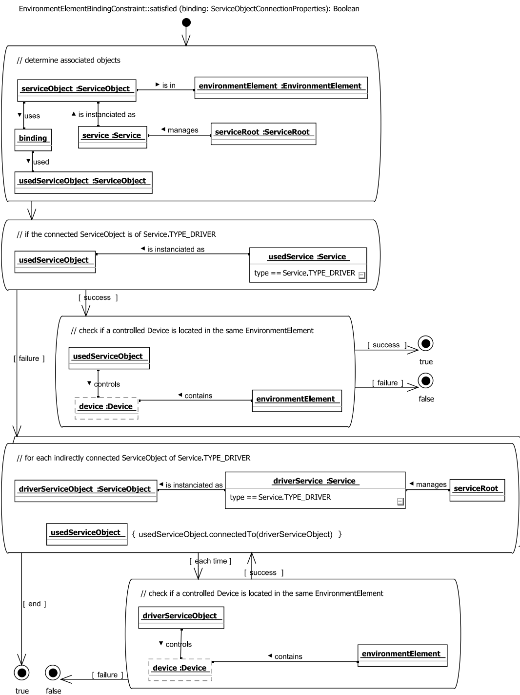
Abbildung 4.23: Überprüfung der Bindungsbeschränkung auf lokale Ressourcen.
