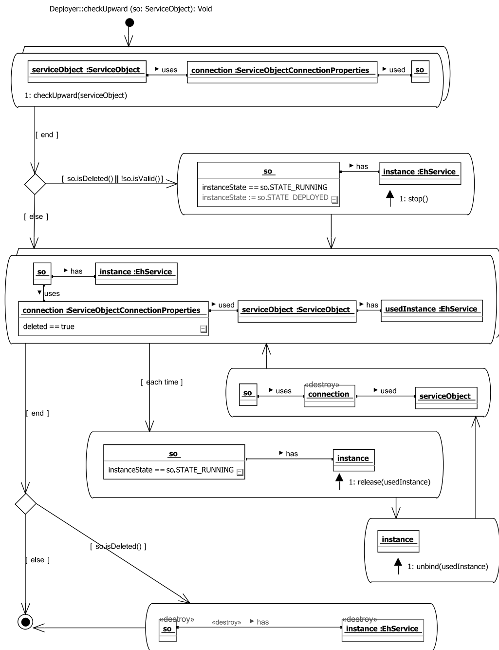
Abbildung 4.32: Realisierung der Aufwärtsprüfung.
