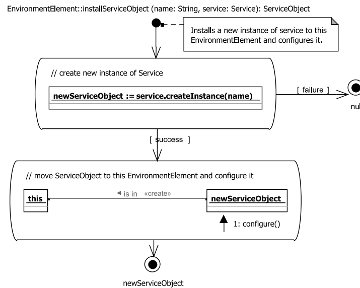
Abbildung 4.19: Erstellen eines ServiceObject.
