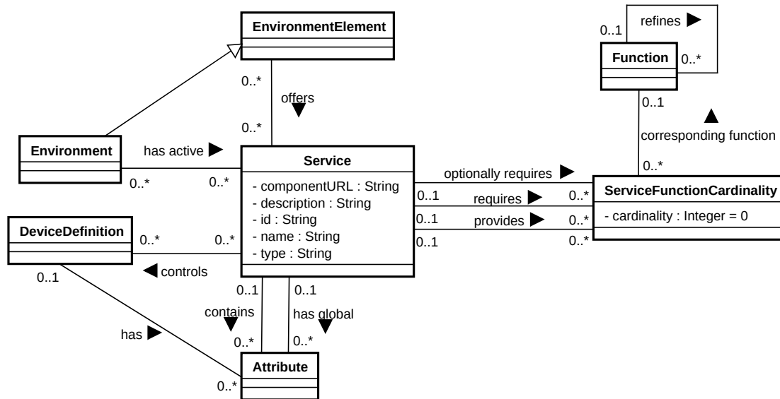
Abbildung 3.10: Ausschnitt des eHome-Modells nach NORBISRATH.
