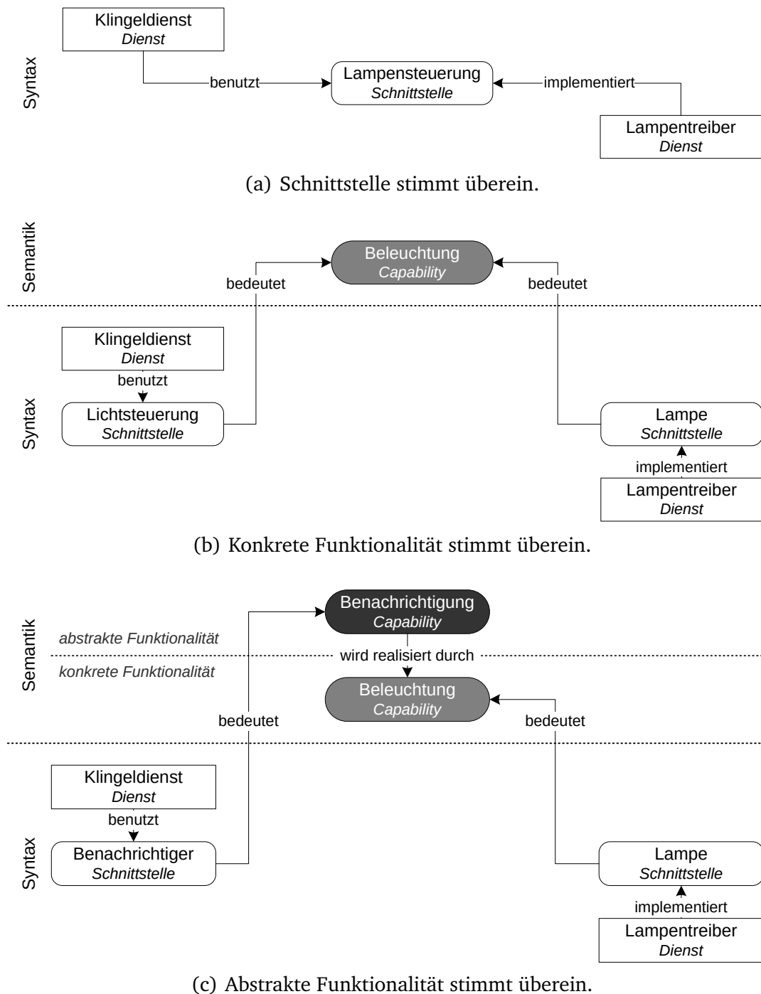
Abbildung 5.17: Verschiedene Ebenen des Matchings.
