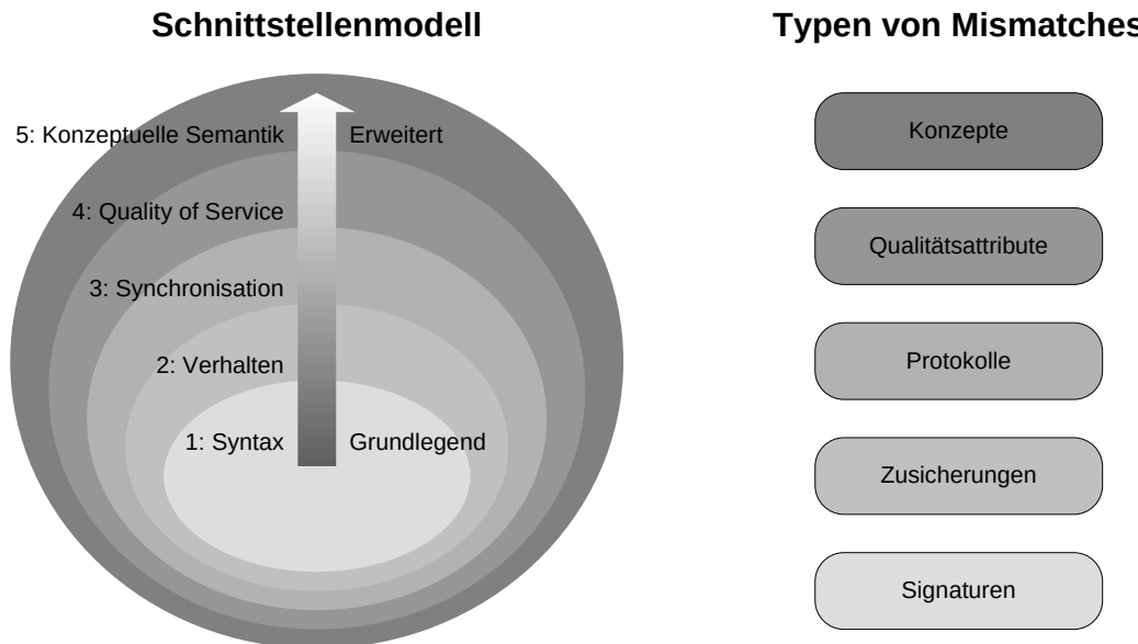
Abbildung 5.5: Verschiedene Typen von Mismatches. (in Anlehnung an [BBG + 06])
