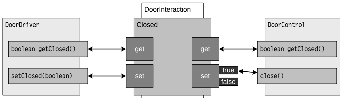
Abbildung 5.18: Funktionalitätsüberdeckung für ein semantisches Match.
