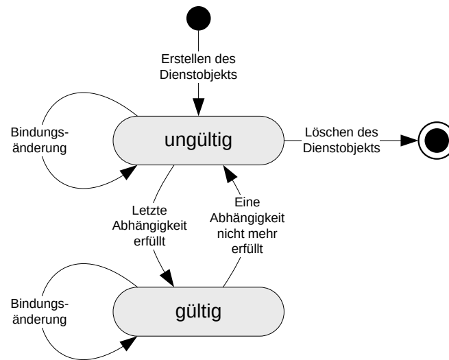
Abbildung 4.20: Zustandsdiagramm für die Konfigurierung von eHome-Diensten.
