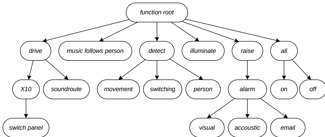
Abbildung 3.9: Hierarchie von Dienstfunktionalitäten. (in Anlehnung an [Nor07])
