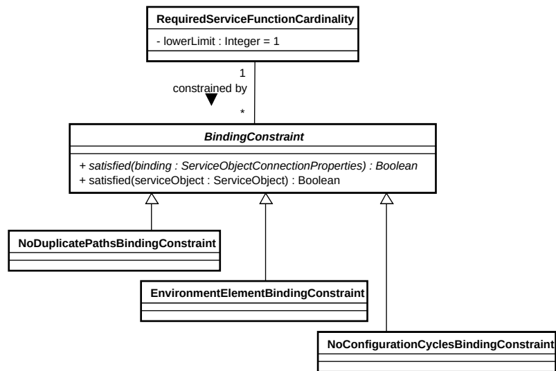
Abbildung 4.11: Modellierung der Bindungsbeschränkungen.
