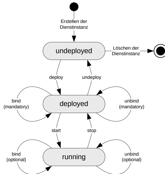
Abbildung 4.29: Zustandsdiagramm für das Deployment von eHome-Diensten.
