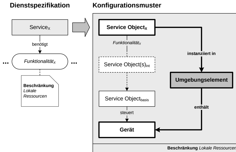
Abbildung 4.4: Bindungsbeschränkung auf lokale Ressourcen.
