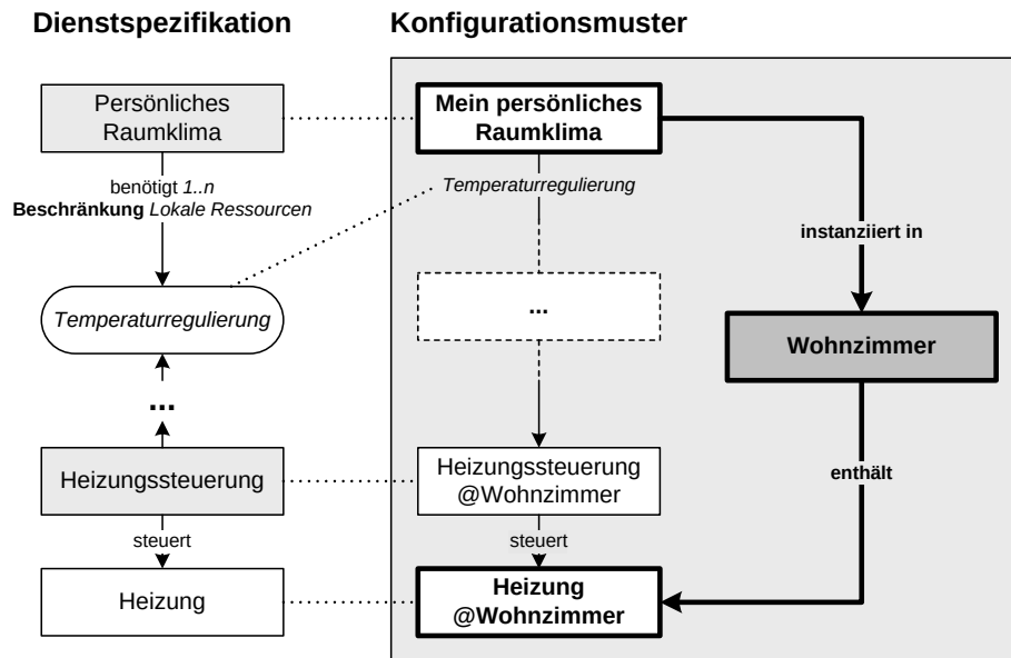
Abbildung 4.5: Beispiel zur Bindungsbeschränkung auf lokale Ressourcen.
