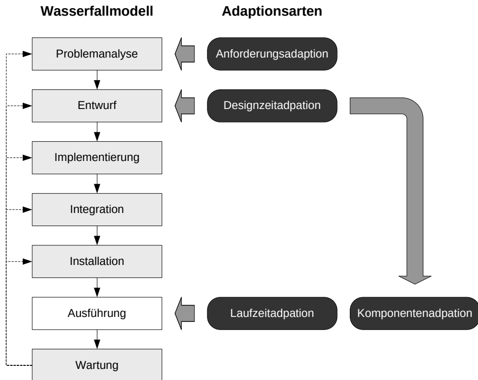
Abbildung 5.6: Zuordnung verschiedener Adaptionarten zu den Phasen des Wasserfallmodells der Softwareentwicklung.
