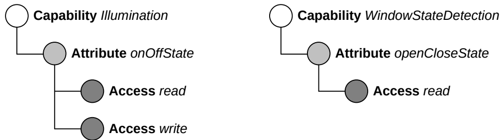
Abbildung 5.12: Beispiele zur Verwendung der Darstellungsontologie.
