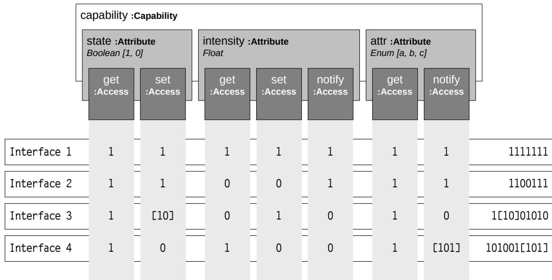
Abbildung 5.19: Beispiel zur Funktionalitätsüberdeckung.
