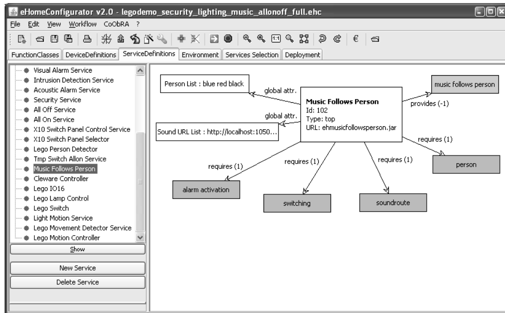
Abbildung 3.11: Dienstspezifikation im eHomeConfigurator.
