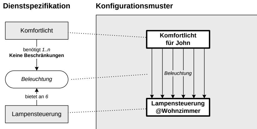
Abbildung 4.8: Beispiel ohne Bindungsbeschränkungen mit erwünschten semantisch äquivalenten Bindungspfaden.
