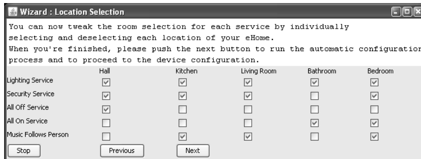
Abbildung 3.12: Zuordnung von Diensten und Räumen im eHomeConfigurator.
