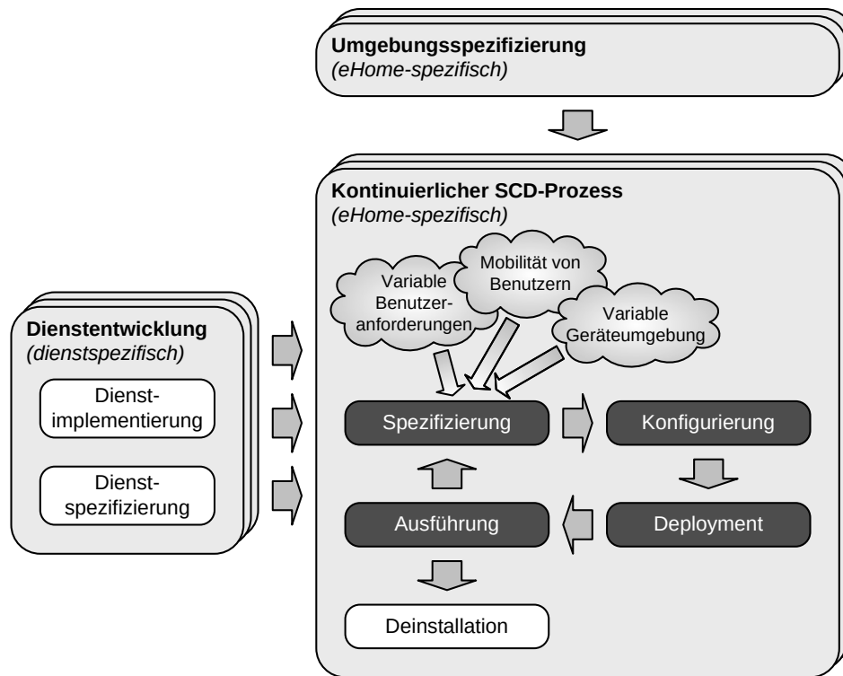
Abbildung 4.2: Erweiterter Entwicklungsprozess für dynamische eHome-Systeme mit eingebettetem kontinuierlichen SCD-Prozess.
