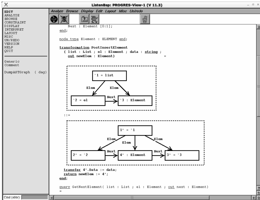
Abbildung 3.4: Editor der PROGRES-Entwicklungsumgebung.
