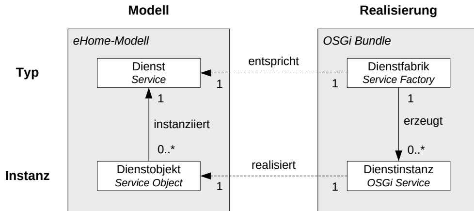
Abbildung 4.25: Zusammenhang von Modell- und Realisierungsebene.
