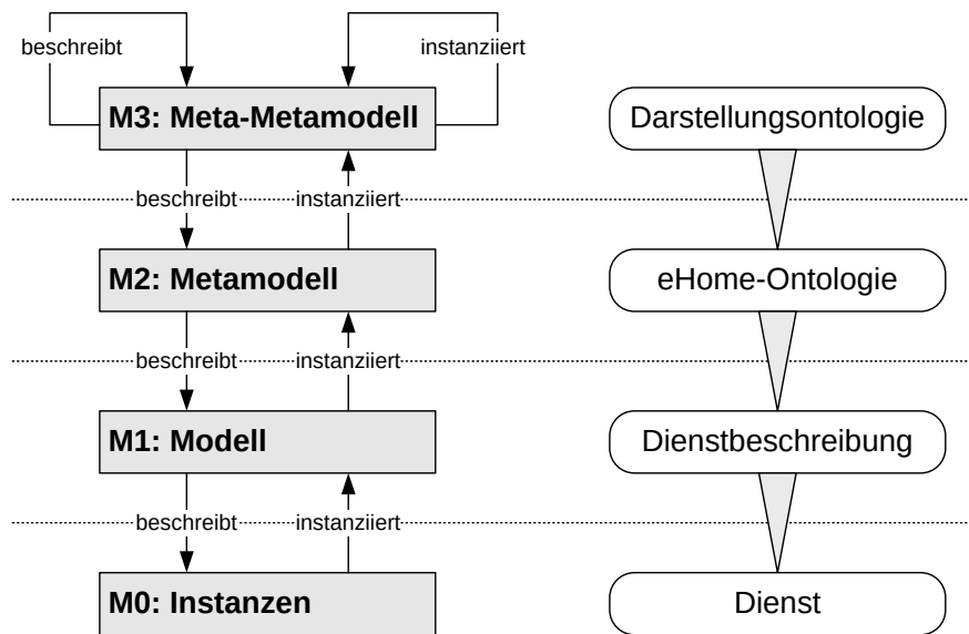
Abbildung 5.10: Vier Ebenen der Metamodellierung (nach [Völ04]) und deren Anwendung auf die Modellierung von eHome-Diensten.
