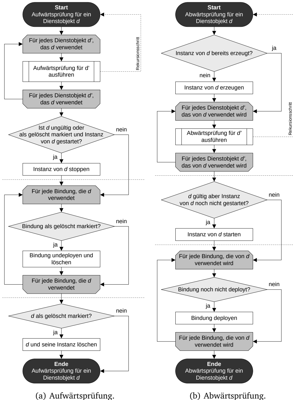
Abbildung 4.30: Adaptionalgorithmus für die Deploymentphase.
