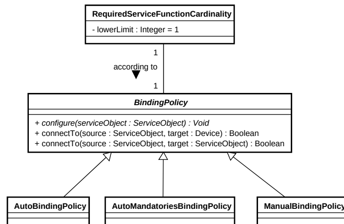
Abbildung 4.13: Modellierung der Bindungsstrategien.
