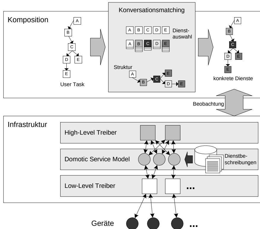
Abbildung 5.22: Übersicht der Architektur des Amigo-Projekts.
