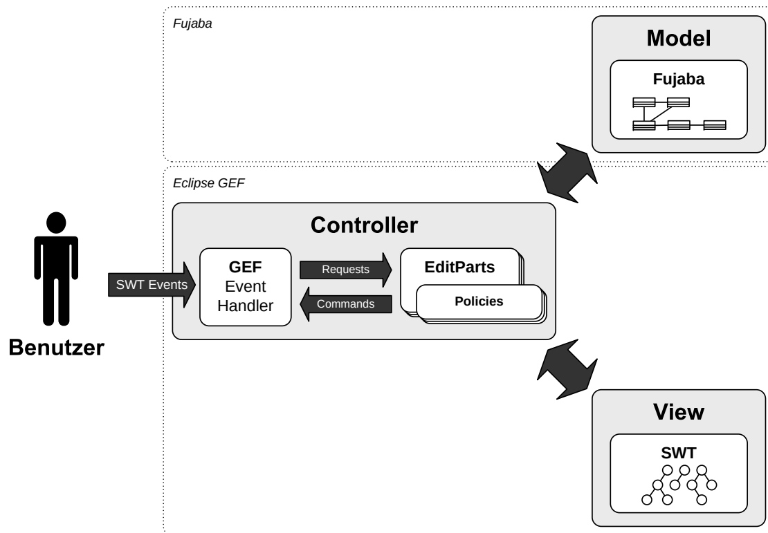
Abbildung 6.2: Anwendung des MVC-Musters mit GEF und Fujaba.
