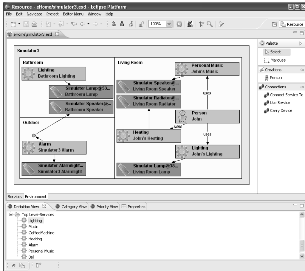
Abbildung 6.11: Hauptfenster des Laufzeit-Managers.
