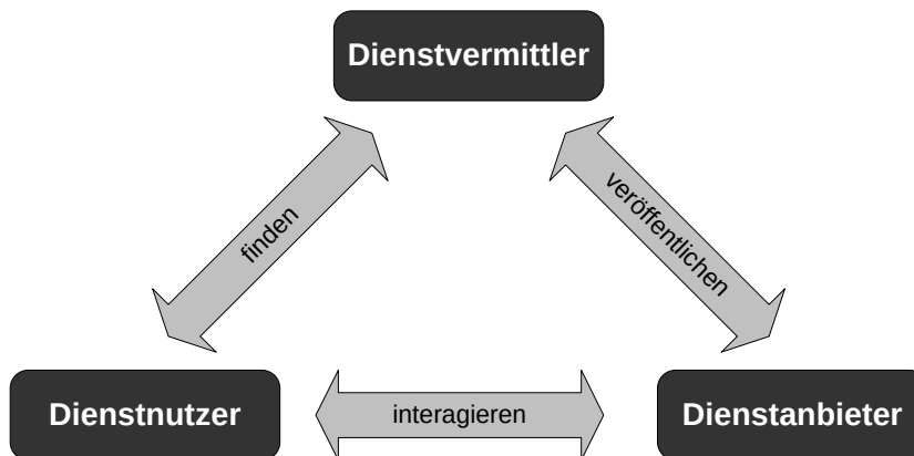
Abbildung 3.1: Rollen und Interaktion in einem serviceorientierten System.
