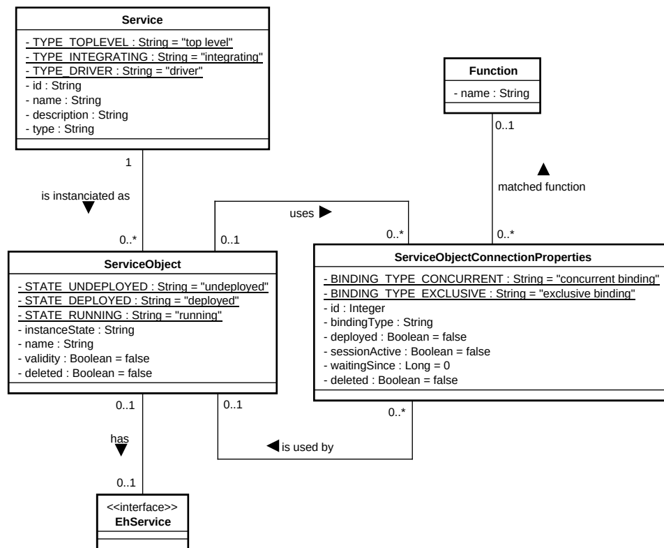
Abbildung 4.24: Modellierung von Dienstobjekten und -bindungen.
