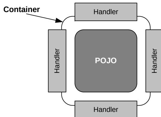
Abbildung 4.34: Nutzung von Handlern in iPOJO. (in Anlehnung an [EHL07])
