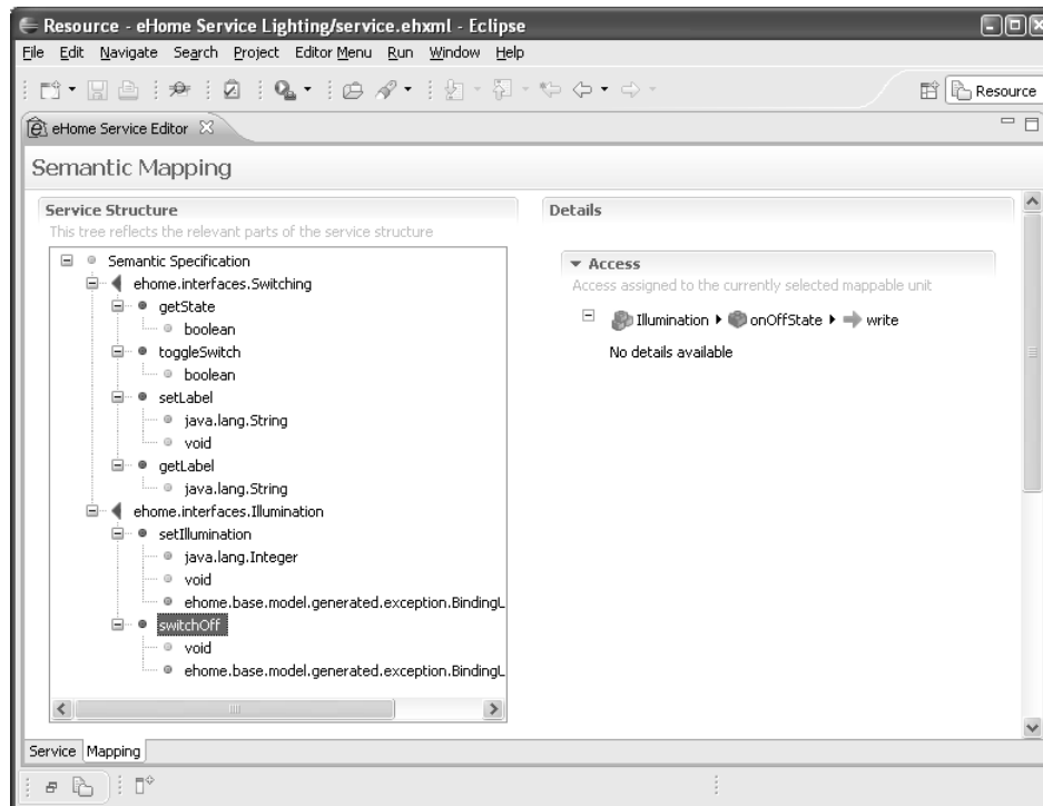
Abbildung 6.7: Spezifikation der semantischen Abbildung.
