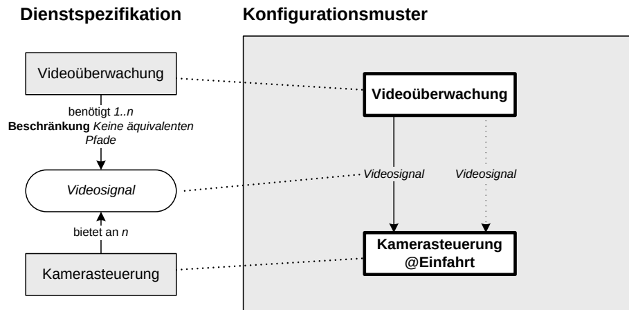
Abbildung 4.7: Beispiel einer Bindungsbeschränkung zum Verhindern semantisch äquivalenter Bindungspfade.
