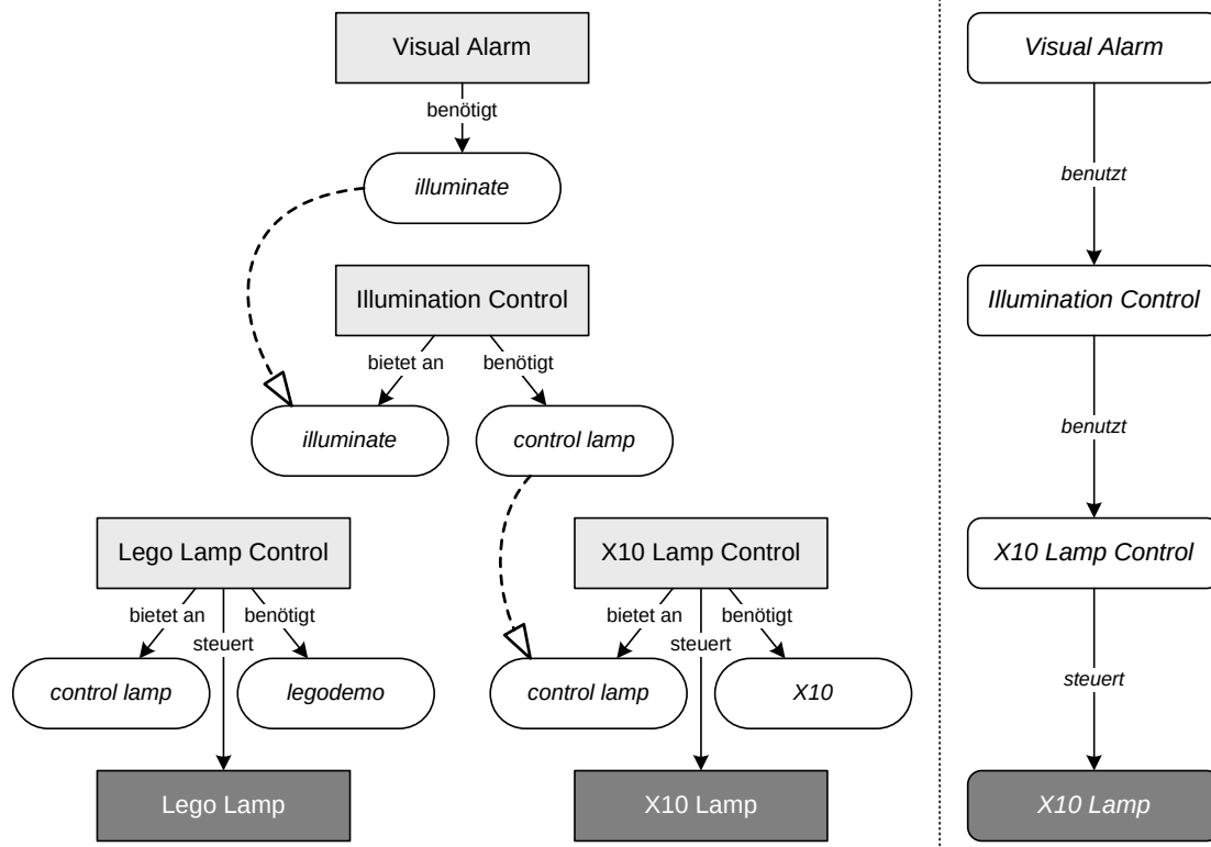
Abbildung 3.8: Schichtenarchitektur der eHome-Dienste.
