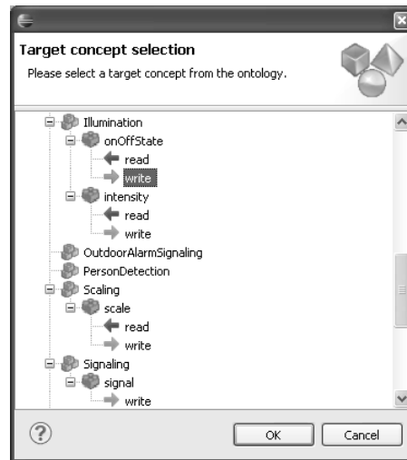
Abbildung 6.8: Auswahl einer Capability aus der eHome-Ontologie.
