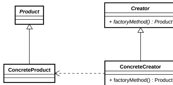
Abbildung 4.26: Entwurfsmuster Factory Method .
