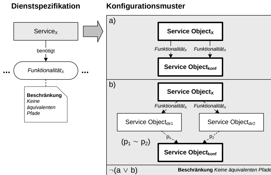
Abbildung 4.6: Bindungsbeschränkung zum Verhindern semantisch äquivalenter Bindungspfade.
