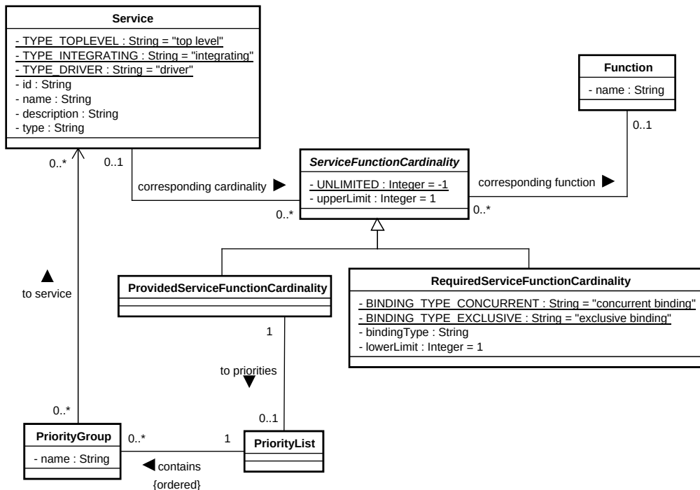
Abbildung 4.16: Modellierung der Bindungstypen.
