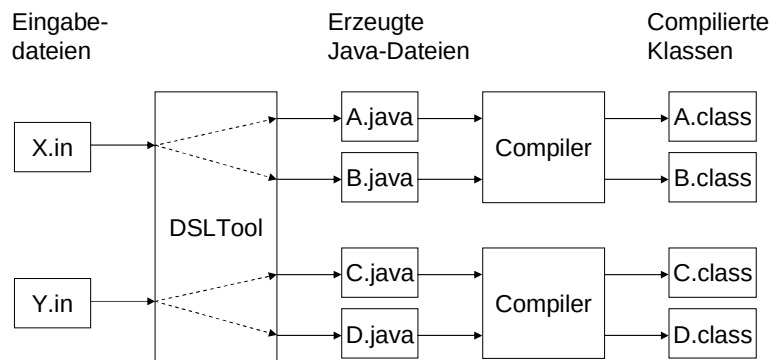
Abbildung 9.16: Unabhängige Codegenerierung aus den Eingabedateien X und Y
