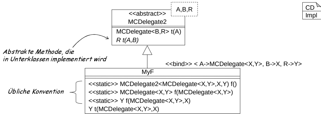
Abbildung 9.13: Klassendiagramm der Funktion MyF
