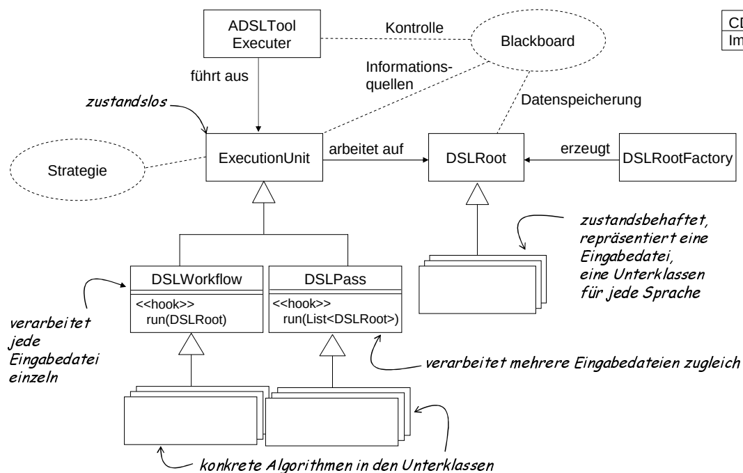
Abbildung 9.1: Zusammenhang zwischen Root-Objekten und ExecutionUnits
