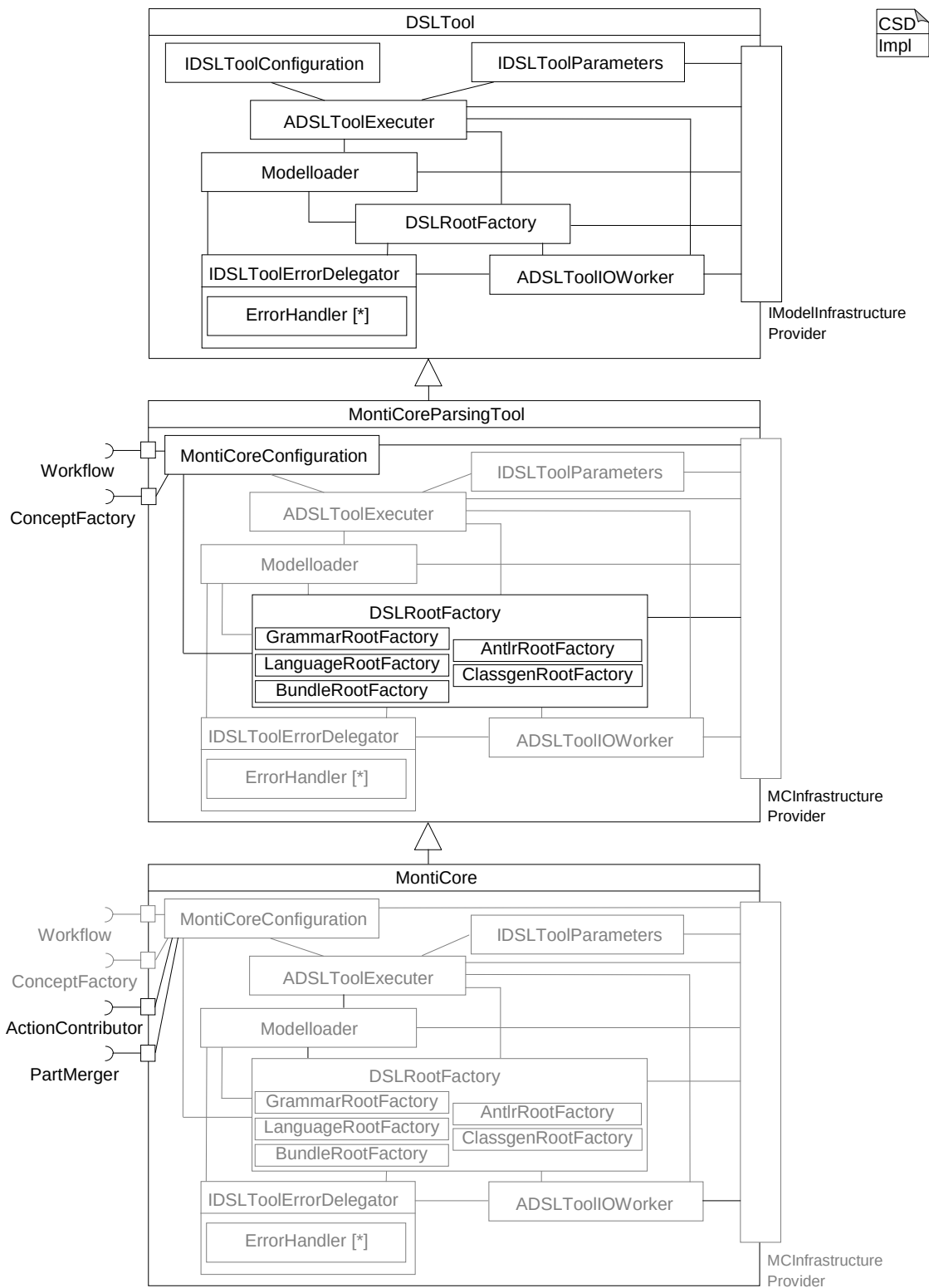
Abbildung 6.5: Zusammenhang der beiden Klassen MontiCoreParsingTool und MontiCore mit der Referenzarchitektur
