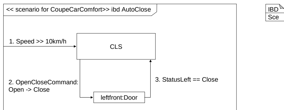
Abbildung 10.7: Funktionsnetz als Szenario
