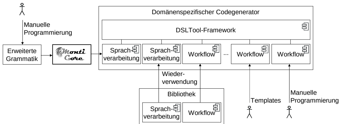
Abbildung 11.1: Übersicht über die Erstellung von domänenspezifischen Codegeneratoren mit MontiCore
