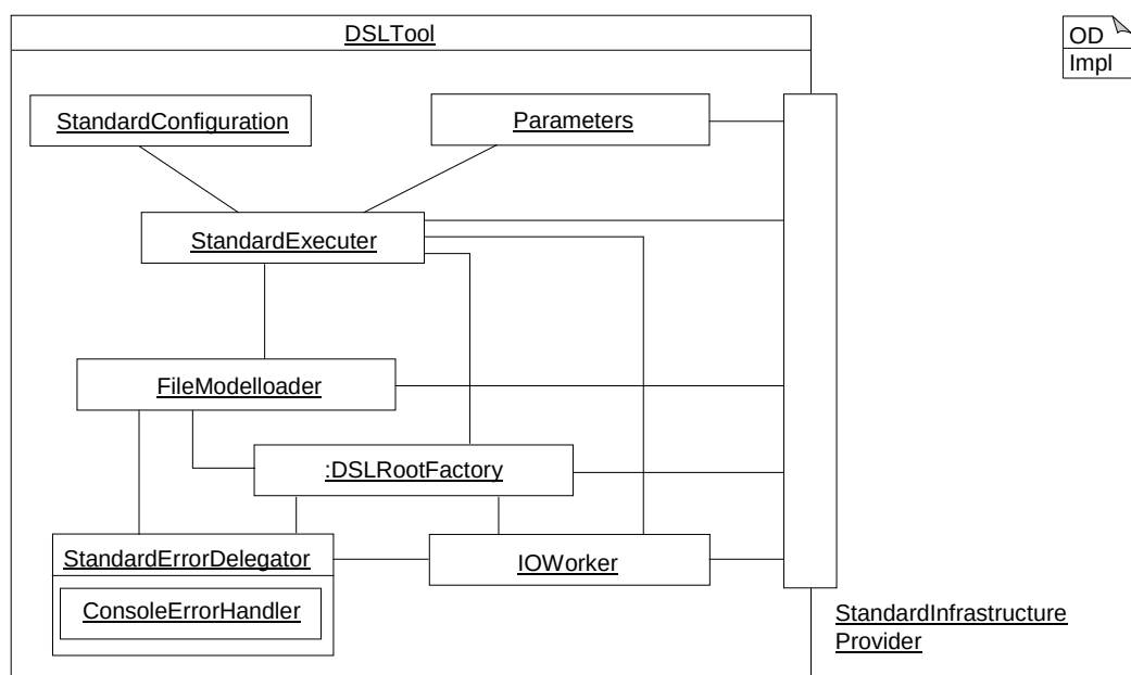
Abbildung 9.4: Standardimplementierungen innerhalb eines DSLTools
