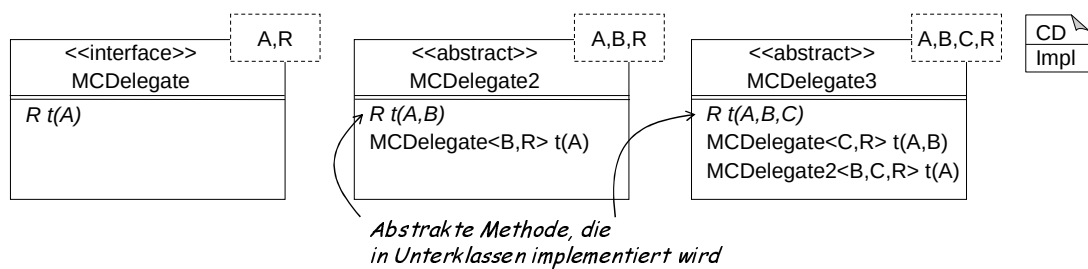
Abbildung 9.12: Übersicht über die MCDelegates
