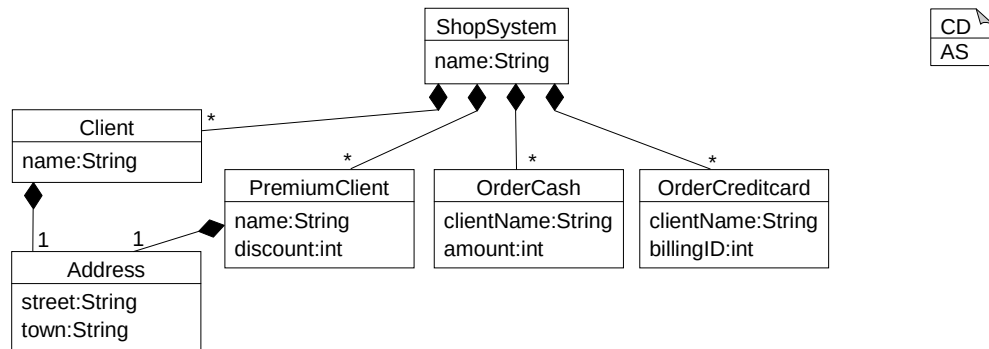
Abbildung 3.3: Aus der Grammatik in Abbildung 3.2 abgeleitete abstrakte Syntax
