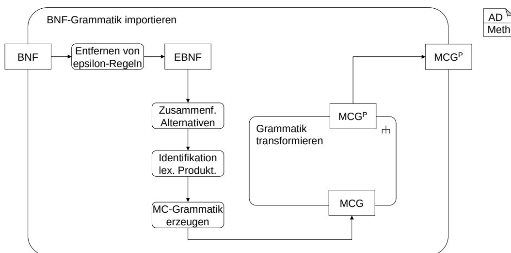
Abbildung 8.7: Importieren einer BNF-Grammatik in das MontiCore-Framework
