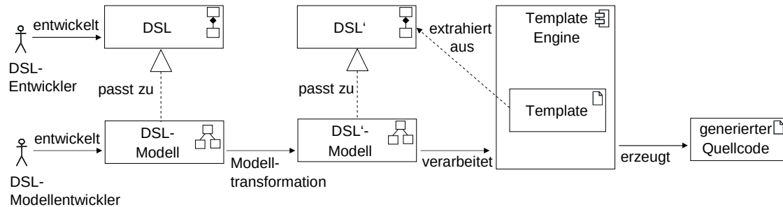
Abbildung 8.11: Einsatz von Templates und Modelltransformationen
