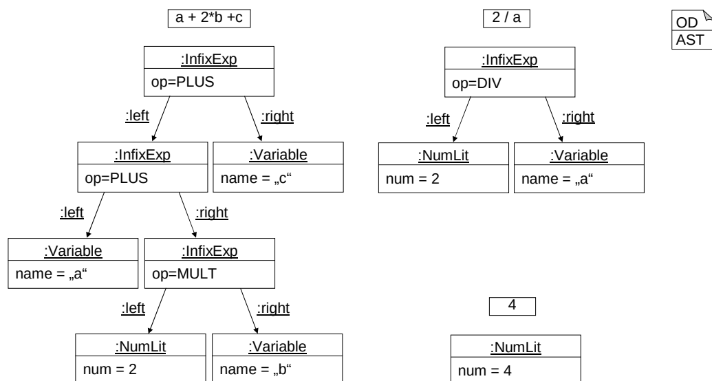
Abbildung 3.14: Beispiele für entstehende ASTs beim Parsen von Ausdrücken
