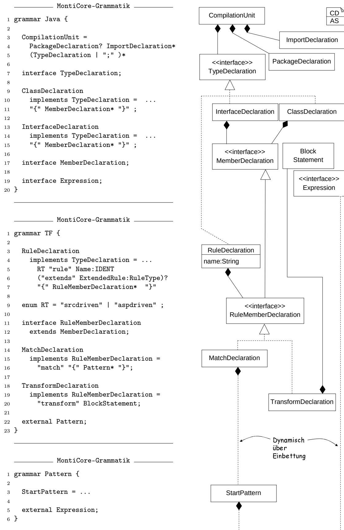
Abbildung 10.14: Grammatiken und abstrakte Syntax von JavaTF
