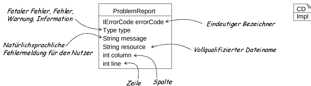
Abbildung 9.10: Attribute der Klasse mc.ProblemReport
