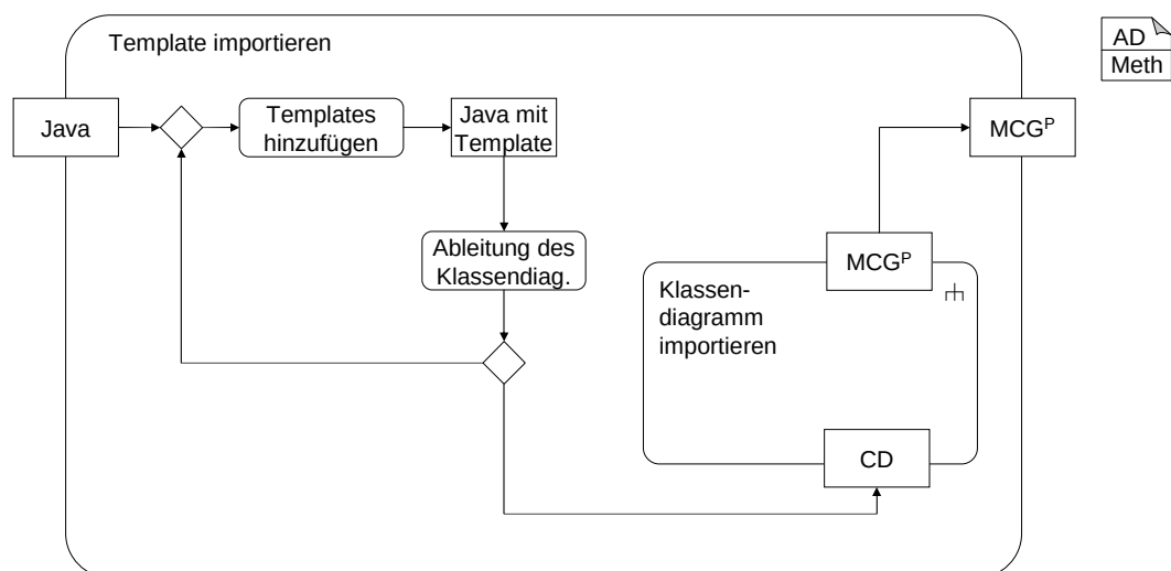
Abbildung 8.10: Importieren eines Templates
