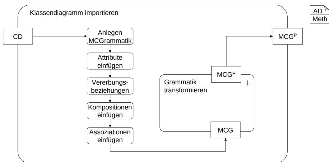
Abbildung 8.3: Importieren eines Klassendiagramms in das MontiCore-Framework
