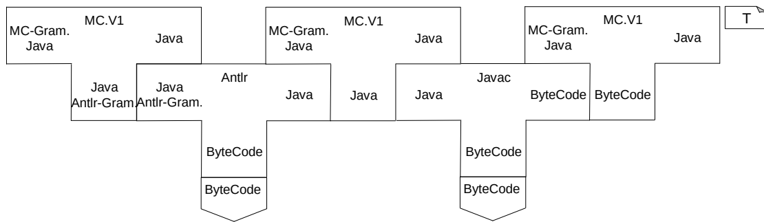
(a) Entwicklung der ersten MontiCore-Version mit Antlr
