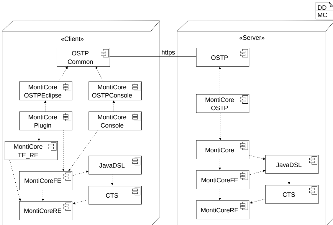
Abbildung 6.1: Komponentendiagramm für den installierten Generator in Eclipse und auf der Konsole mit den Abhängigkeiten zwischen den Modulen.
