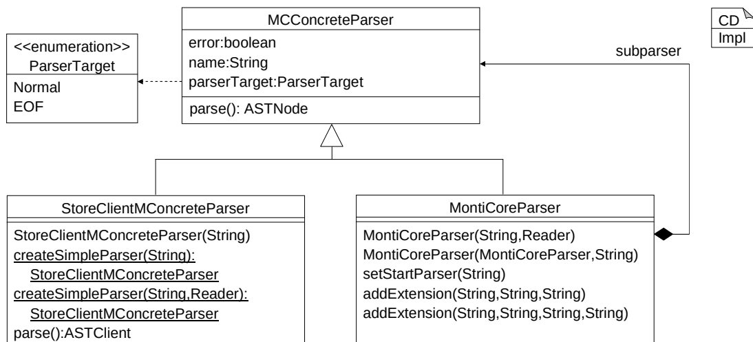
Abbildung 6.3: Grundstruktur der Parser im MontiCore-Framework
