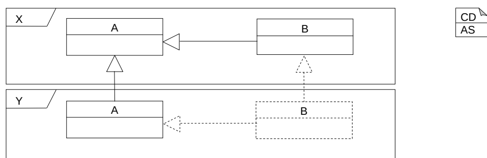
Abbildung 4.5: Problem bei der Grammatikvererbung von Klassenproduktion, die bereits Unterproduktionen haben
