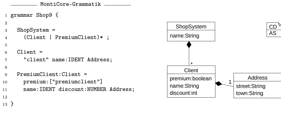
Abbildung 3.12: Mehrteilige Klassenproduktionen
