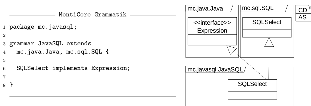
Abbildung 4.1: Mehrfache Grammatikvererbung
