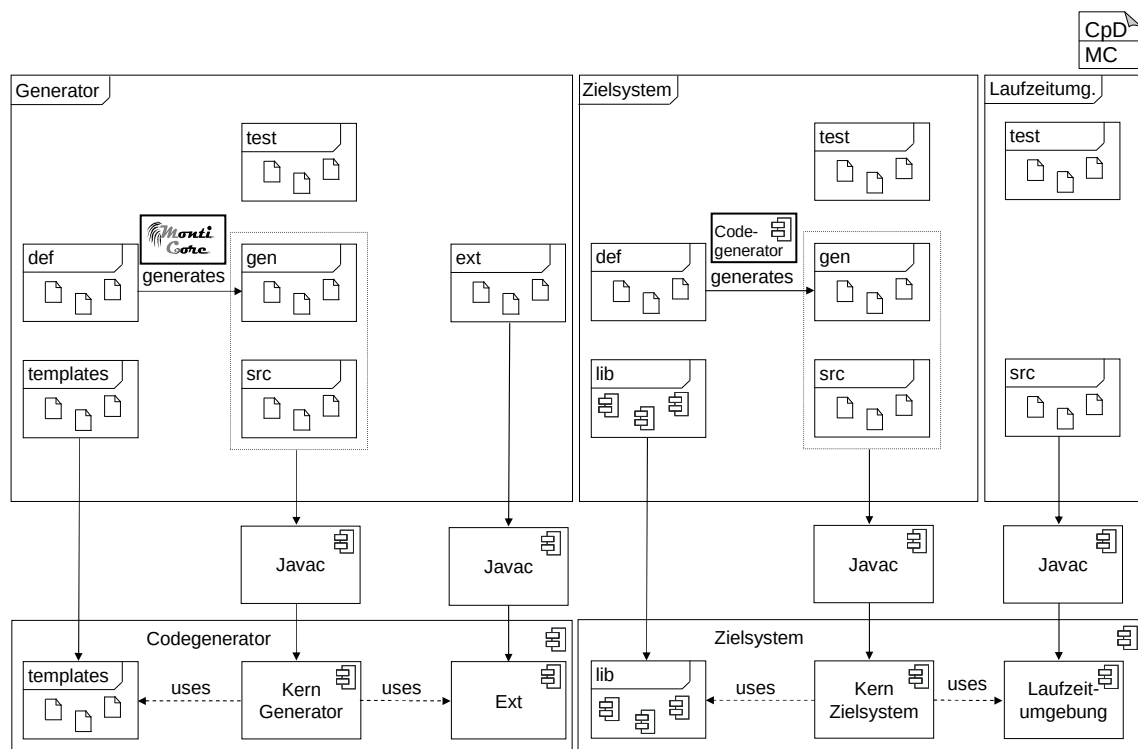
Abbildung 6.7: Komponentendiagramm eines Generators, der dazugehörigen Laufzeitumgebung und des Zielsystem.
