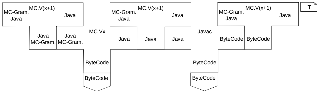
(b) Entwicklung der folgenden Versionen mit MontiCore
