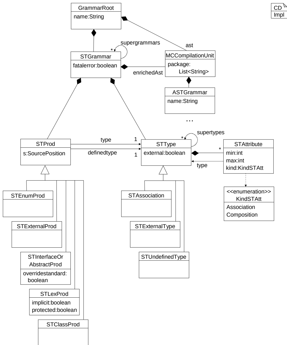
Abbildung 6.6: Klassendiagramm der Symboltabelle des MontiCore-Grammatikformats
