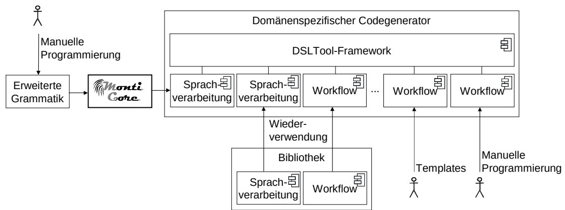
Abbildung 1.5: Übersicht über die Erstellung von domänenspezifischen Codegeneratoren mit MontiCore
