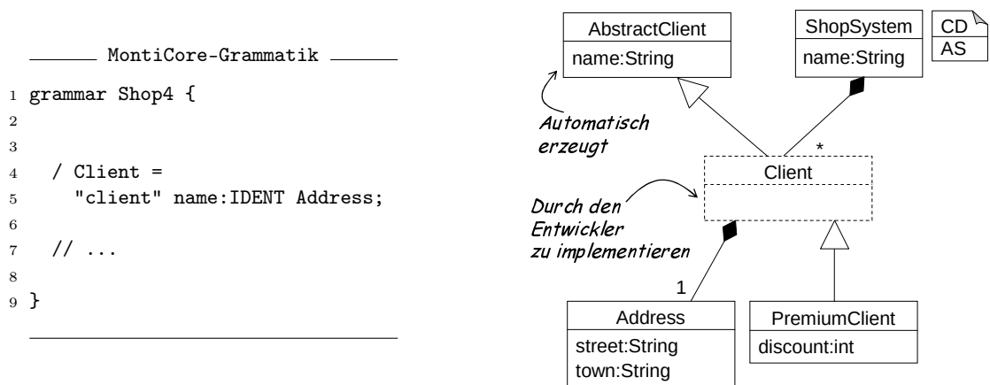
Abbildung 3.7: Verwendung von handcodierten Klassen (Erweiterung der Grammatik aus Abbildung 3.6).
