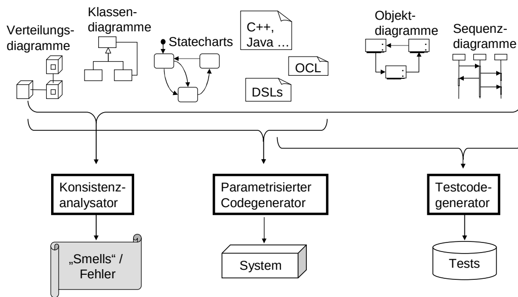
Abbildung 1.1: Agile modellgetriebene Entwicklung (adaptiert aus [Rum04a])
