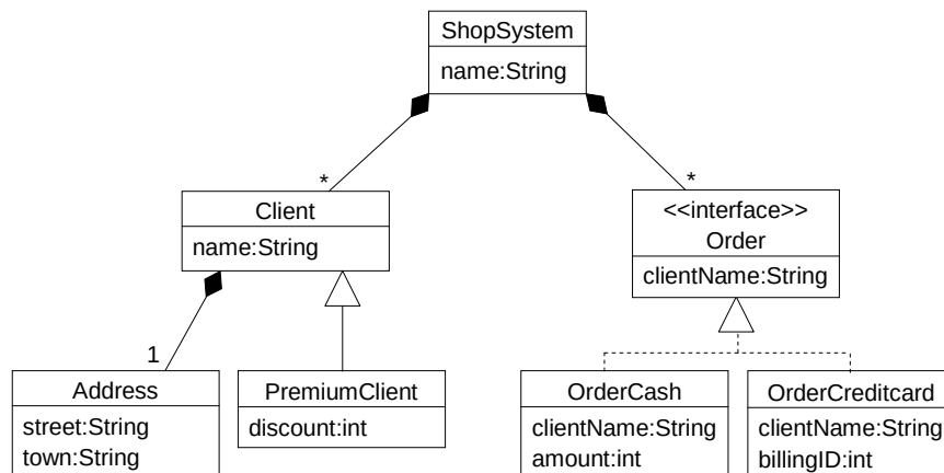
Abbildung 3.6: Vererbung und die Verwendung von Schnittstellen
