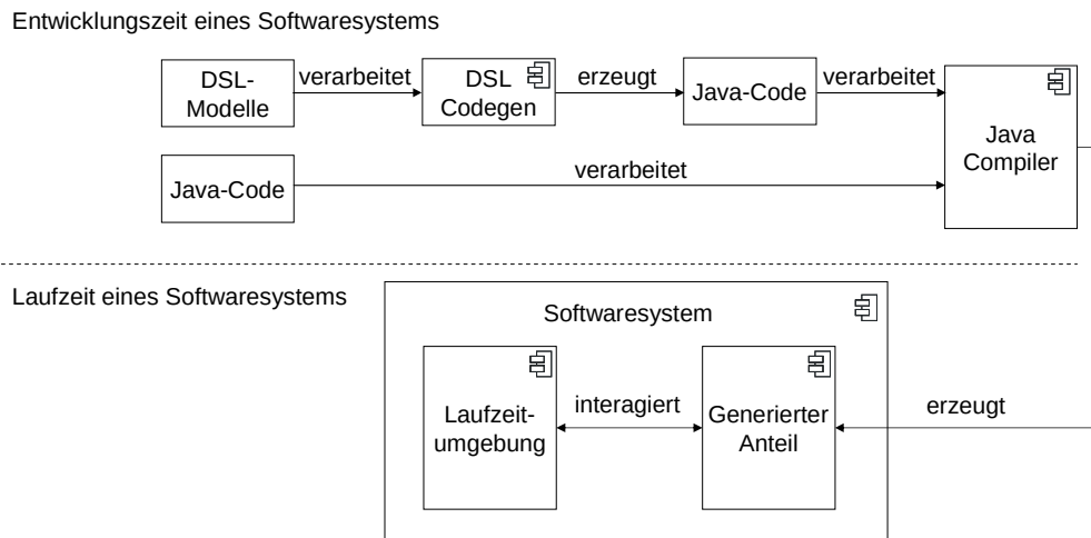
Abbildung 1.4: Verwendung von domänenspezifischen Codegeneratoren
