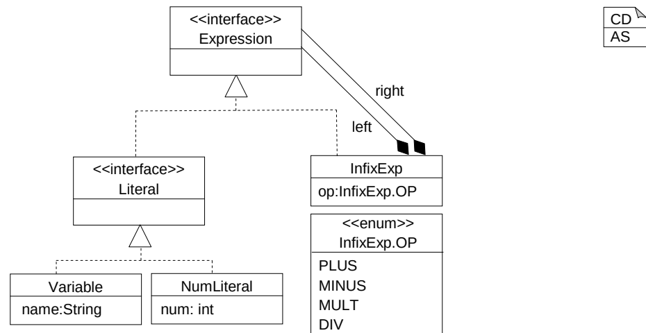
Abbildung 3.13: Realisierung von Ausdrücken in MontiCore
