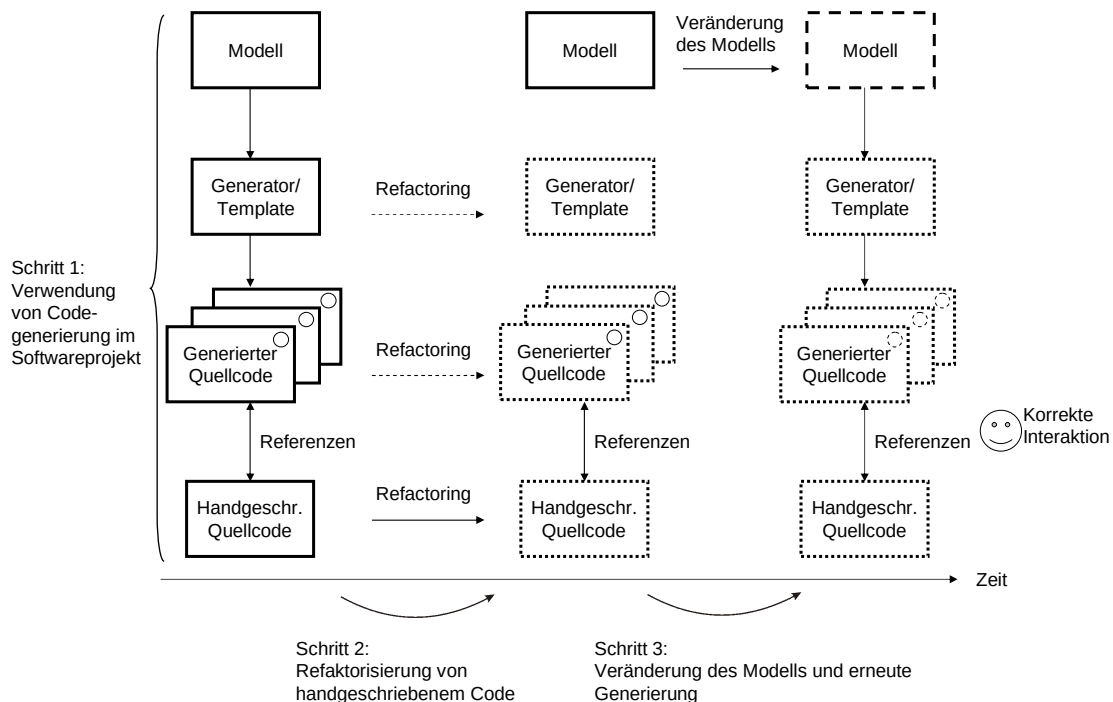
Abbildung 9.23: Koevolution des Templates mit dem generierten Code durch Refactoring
