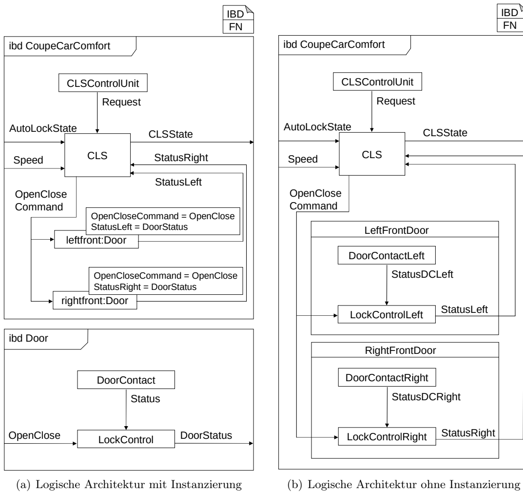
Abbildung 10.5: Modellierung der logischen Architektur mit Funktionsnetzen
