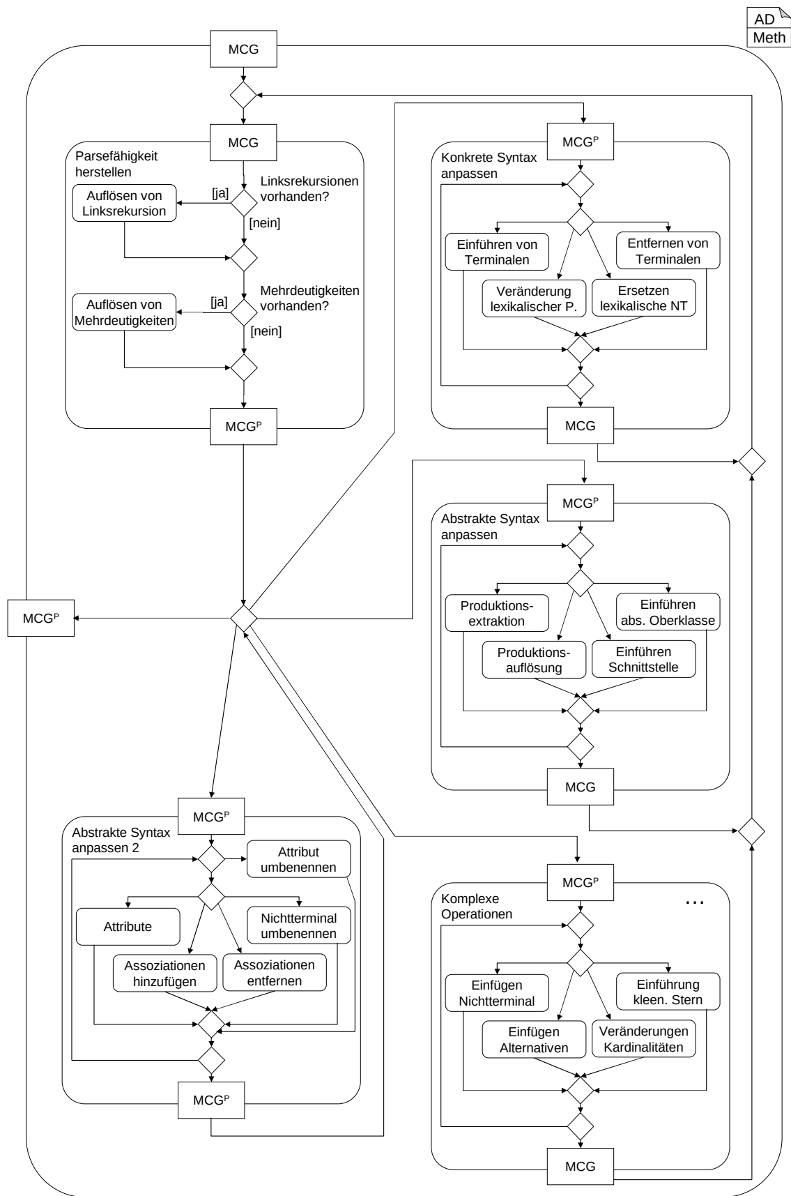
Abbildung 8.1: Transformationen einer MontiCore-Grammatik
