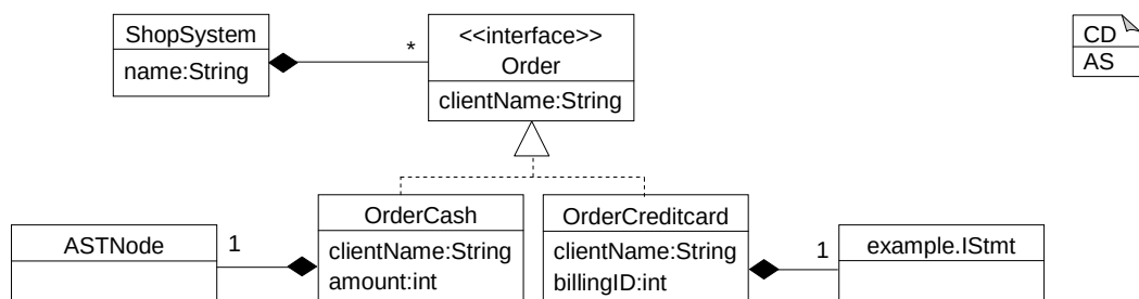
Abbildung 4.8: Aus Abbildung 4.7 abgeleitete abstrakte Syntax
