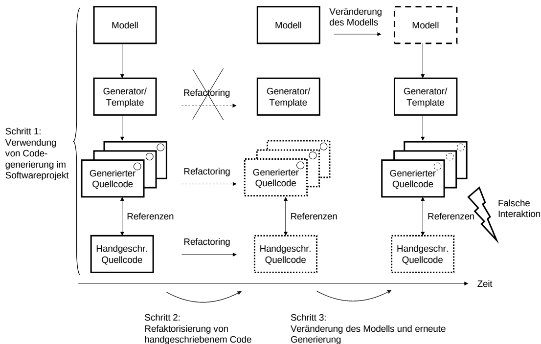
Abbildung 9.22: Inkonsistenz des Templates mit dem generierten Code durch Refactoring beim herkömmlichen Verfahren
