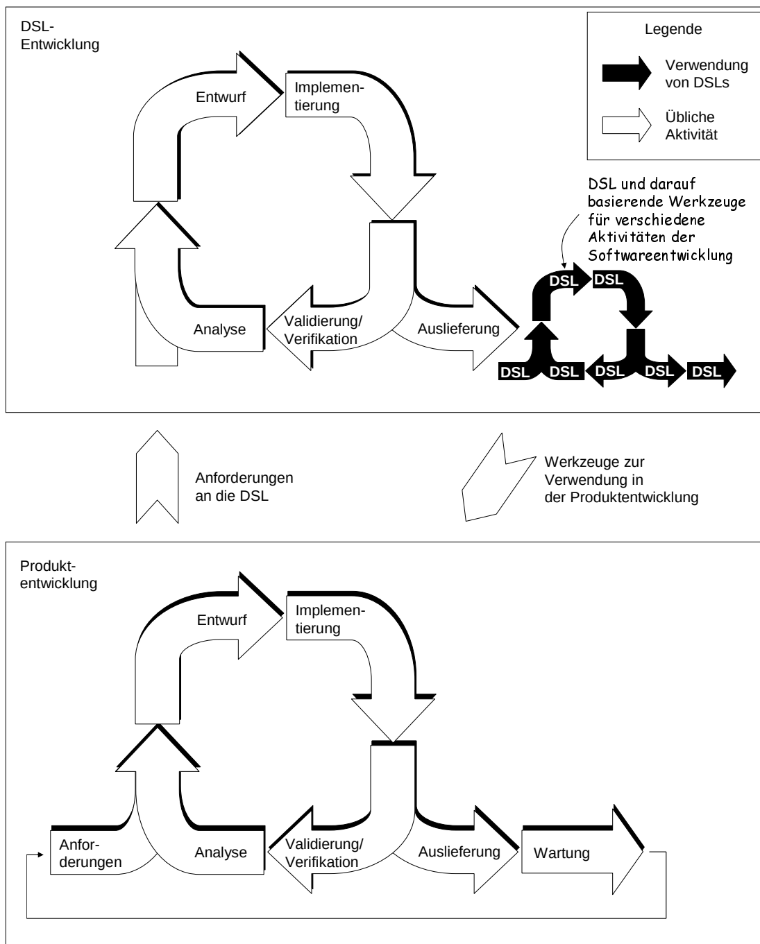
Abbildung 2.3: Agile Kopplung der DSL-Entwicklung mit der Softwareentwicklung
