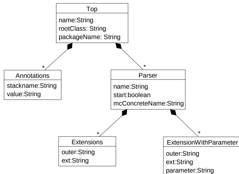
Abbildung 8.13: Das aus dem Template aus Abbildung 8.14 extrahierte Datenmodell
