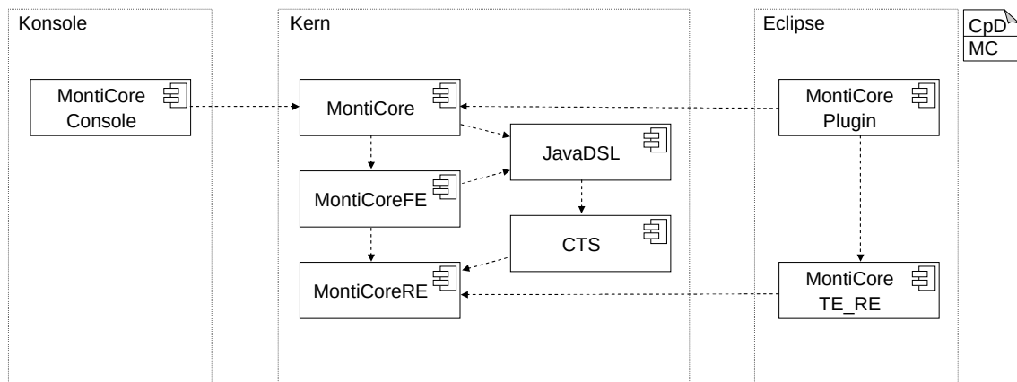
Abbildung 6.1: Komponentendiagramm für den installierten Generator in Eclipse und auf der Konsole mit den Abhängigkeiten zwischen den Modulen.
