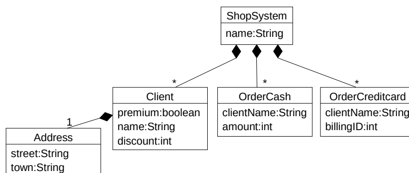
Abbildung 3.4: Definition des ShopSystems mit Konstanten und die daraus abgeleitete abstrakte Syntax
