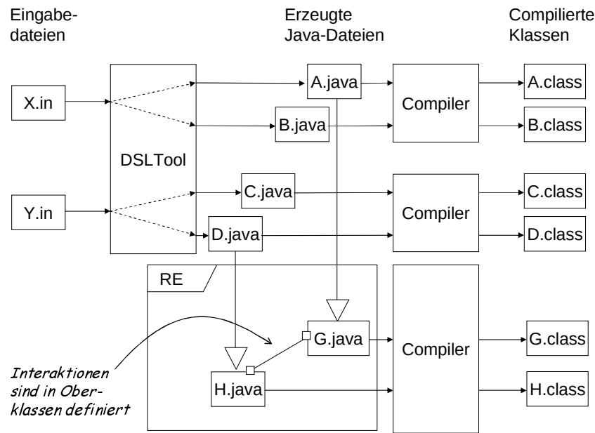
Abbildung 9.17: Verwendung einer Laufzeitumgebung zur unabhängigen Compilierung
