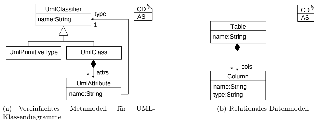
Abbildung 10.10: Abstrakte Syntax der Quell- und Zielmodelle
