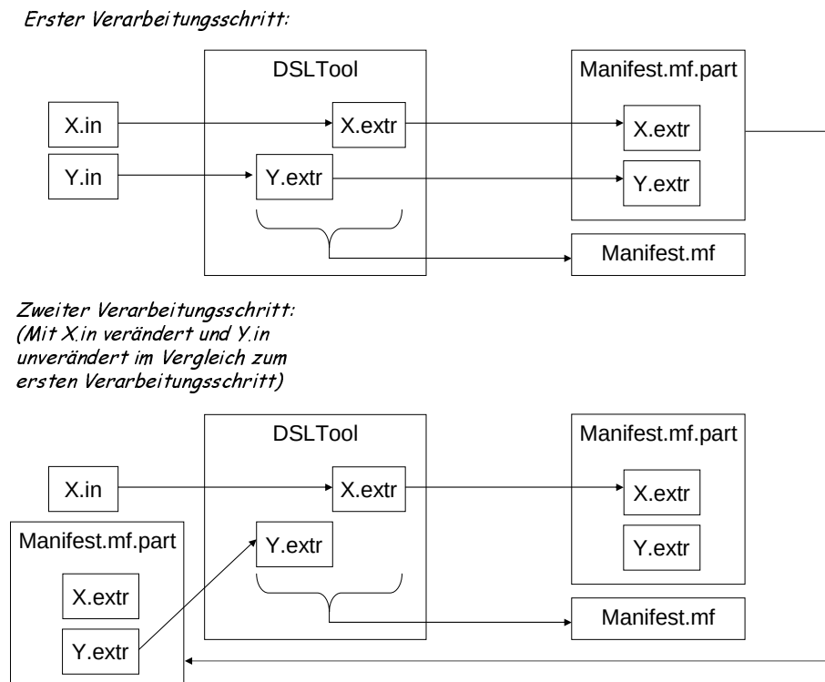
Abbildung 9.18: Verwenden von Parts innerhalb einer Codegenerierung
