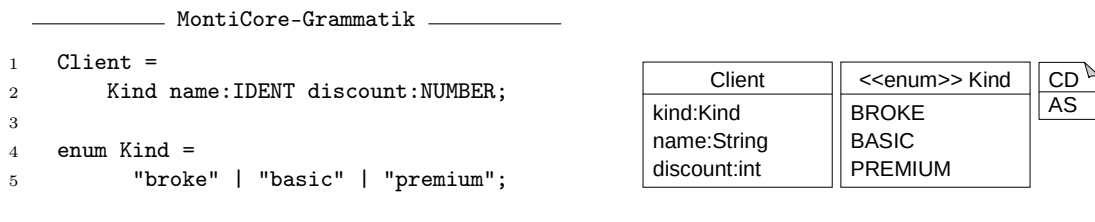
Abbildung 3.5: Verwendung von Enumerations-Produktionen
