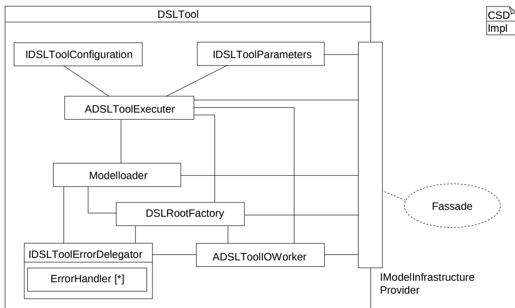
Abbildung 9.3: Architektur eines DSLTools
