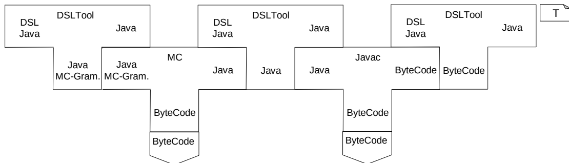
(c) Zweistufige Compilierung beim Einsatz von MontiCore zur Entwicklung eines DSLTools
