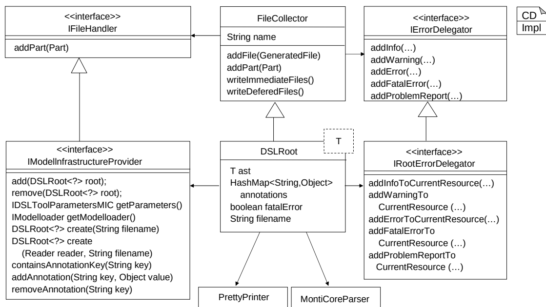
Abbildung 9.2: Umgebung der Klasse mc.DSLRoot
