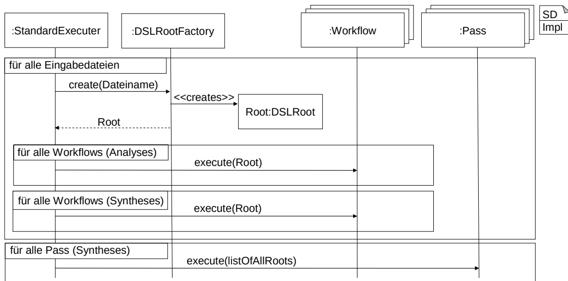
Abbildung 9.6: Verhalten der Klasse mc.StandardExecuter
