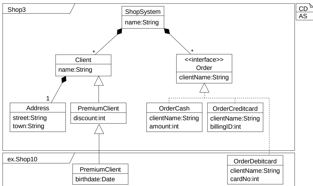
Abbildung 4.4: Abstrakte Syntax
