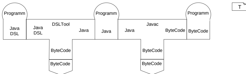
(d) Zweistufige Compilierung beim Einsatz des DSLTools zur Entwicklung eines Programms
