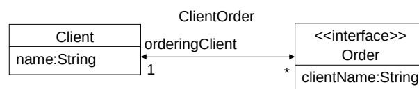
Abbildung 4.11: Auszug aus der aus Abbildung 4.10 abgeleiteten abstrakten Syntax
