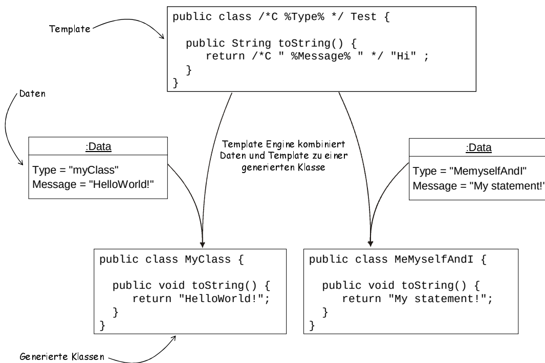
Abbildung 9.24: Anwendung der Template-Engine
