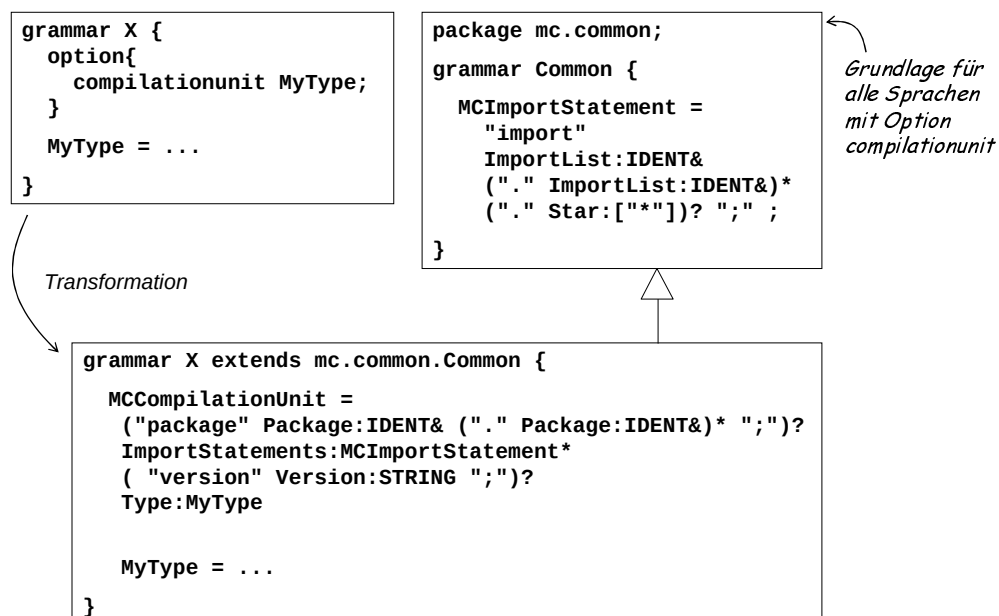
Abbildung 9.20: Auswirkungen der Option compilationunit auf die Sprachdefinition
