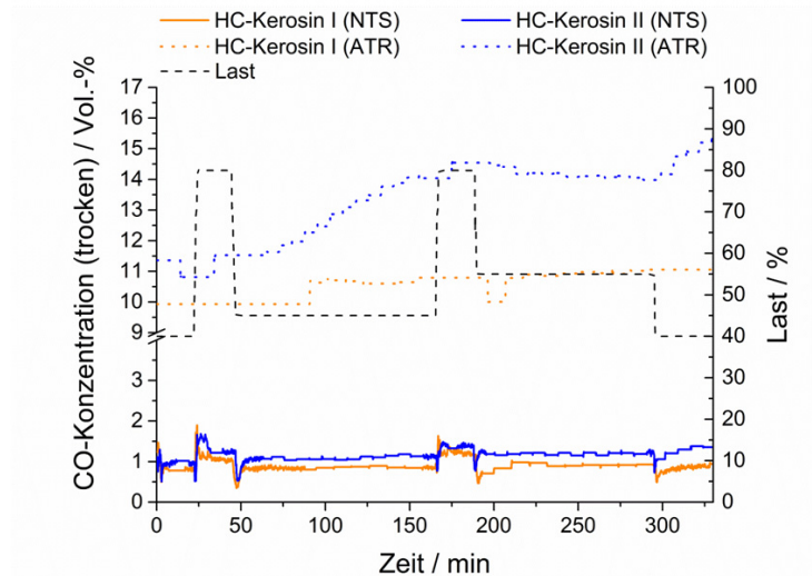
Abbildung 8.13: CO-Konzentrationen hinter dem NTS-Reaktor und dem ATR für die Versuche „HC-Kerosin I“ und „HC-Kerosin II“ bei dem Profil „Lutsey Modi Mittel“. Messwerte nach „Multigas™ 2030D“ und „Cirrus™ 2“.
