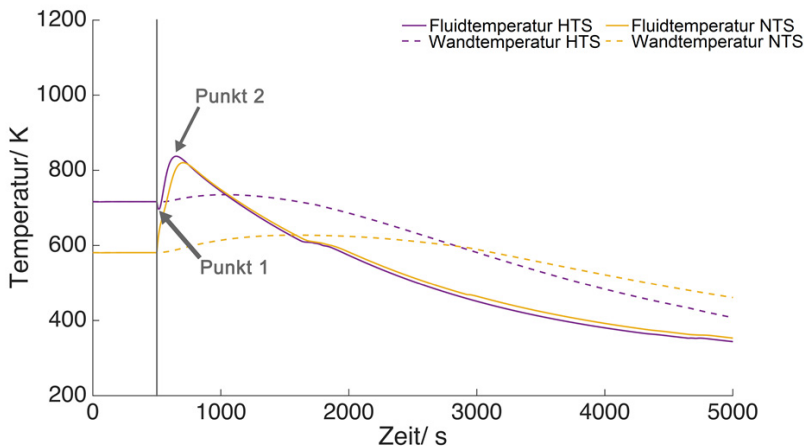
Abbildung 9.3: Fluid- und Wandtemperaturen im Wassergas-Shift-Reaktor während des Abfahrvorgangs. Als Spülmedium wurde Luft mit 20000\text{ l/h} gewählt.
