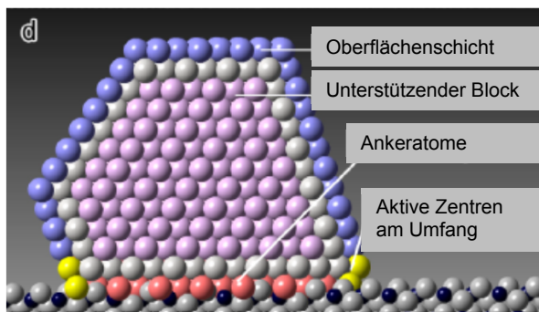
Abbildung 3.3: Schema eines Gold-Nanopartikels, welches auf dem Washcoat CeO 2 verankert ist. Nachgebildet mit Genehmigung von [93]. Copyright (2012) American Chemical Society.
