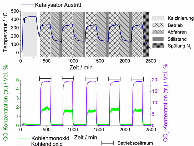
Abbildung 6.5: Testprozedur und Beispieltest des Abfahrvorgänge am Katalysator-Testreaktor. Nachgebildet aus [160] mit Genehmigung von ECS – The Electrochemical Society.
