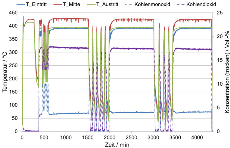
Abbildung 15.11: Stabilität von Katalysator B bei drei unterschiedlichen Temperaturzyklusintervallen. Betrieb unter HTS-Bedingungen und idealem Reformat. Messwerte nach „Multigas™ 2030D“ und „Circus™ 2“.
