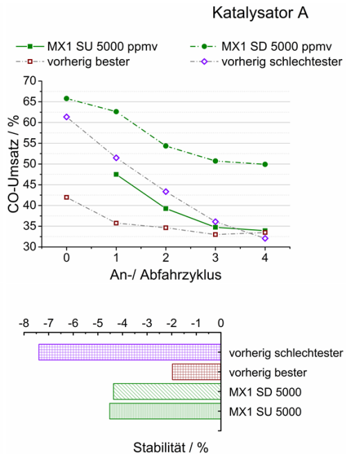
Abbildung 6.17: Einfluss von C_nH_m -Mischungen auf die Stabilität von Katalysator A während des An- und Abfahrens (MX=mixture, SU=startup, SD=shutdown). Messwerte nach „Multigas™ 2030D“ und „Cirrus™ 2“.
