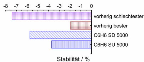
Abbildung 6.15: Einfluss von C_6H_6 auf die Stabilität von Katalysator A während des An- und Abfahrens (SU=startup, SD=shutdown). Messwerte nach „Multigas™ 2030D“ und „Cirrus™ 2“.
