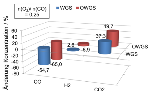
Abbildung 7.6: Durchschnittliche Änderung der Konzentrationen an \text{CO} , \text{H}_2 und \text{CO}_2 während des WGS- und OWGS-Betriebs mit Katalysator B. Es wurden HTS-Bedingungen und ein molares \text{O}_2/\text{CO} -Verhältnis von 0,25 gewählt. Messwerte nach „Multigas™ 2030D“ und „Cirrus™ 2“.
