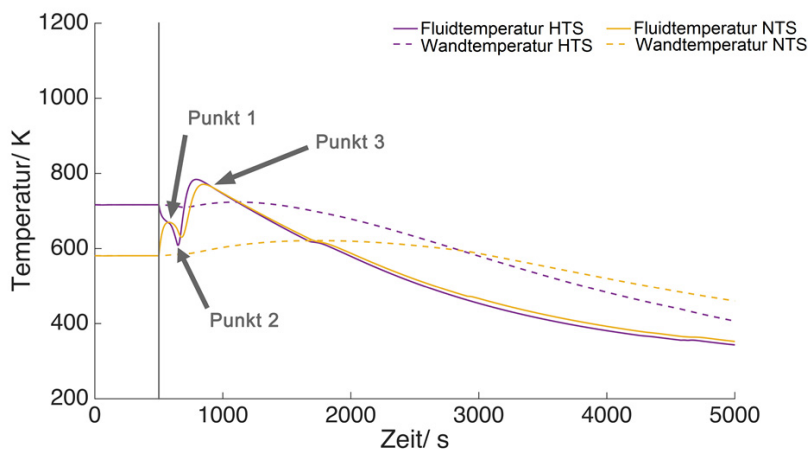
Abbildung 15.17: Fluid- und Wandtemperaturen im Wassergas-Shift-Reaktor während des Abfahrvorgangs. Als Spülmedium wurde Wasserdampf mit 10000 g/h gewählt. Nach T_{krit} wurden 20000 l/h Luft dem Reformier zugegeben.
