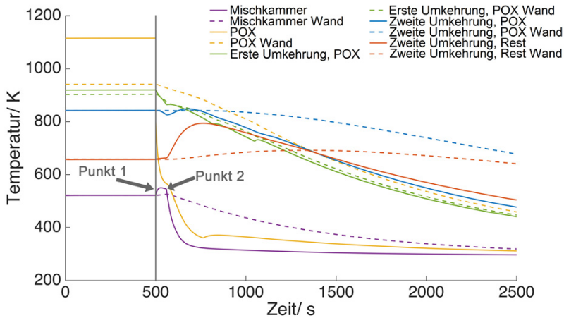
Abbildung 15.19: Fluid- und Wandtemperaturen im autothermen Reformier während des Abfahrvorgangs. Als Spülmedium wurde Luft/ Wasserdampf mit 10000 l/h Luft und 10000 g/h Wasserdampf gewählt. Nach T_{krit} wurde die Wasserdampfzufuhr unterbunden.
