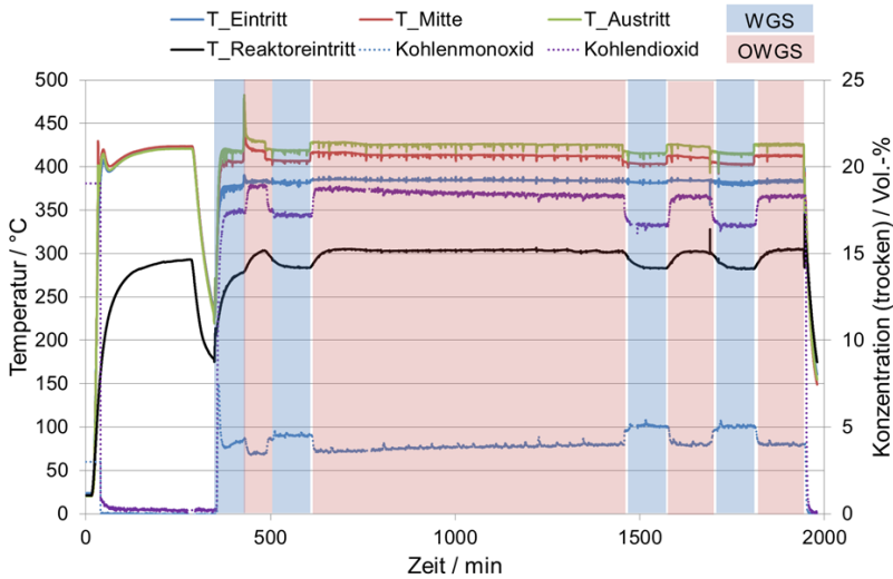
Abbildung 7.5: Temperaturen und Konzentrationen während der Untersuchung von wechselndem WGS und OWGS-Betrieb bei Katalysator B. Es wurden HTS-Bedingungen und ein molares \text{O}_2/\text{CO} -Verhältnis von 0,25 gewählt. Messwerte nach „Multigas™ 2030D“ und „Cirrus™ 2“.
