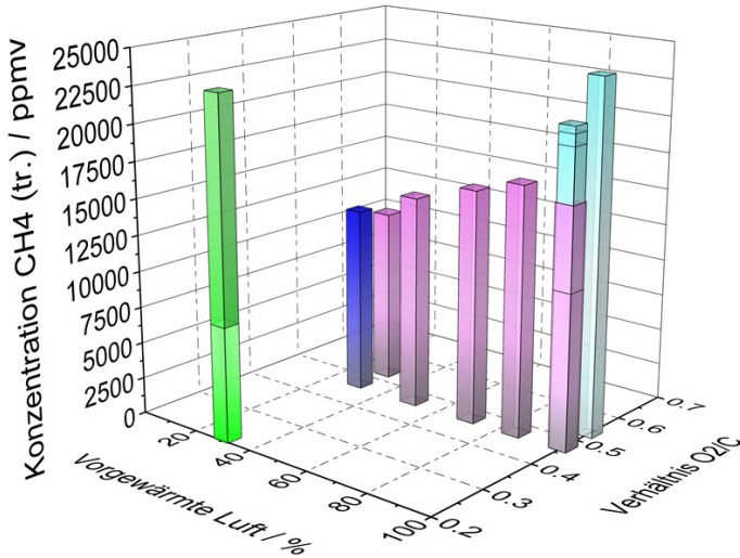
Abbildung 15.13: Maximalkonzentrationen von \text{CH}_4 während des Systemstarts mit NExBTL. Farben: grün: klassische Strategie; blau: neue Strategie 1; magenta: neue Strategie 2; cyan: neue Strategie 3.
