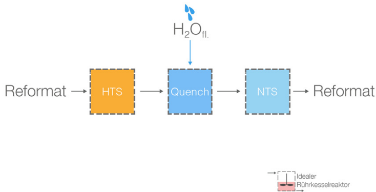
Abbildung 4.12: Gesamtmodell des Wassergas-Shift-Reaktors WGS 4.
