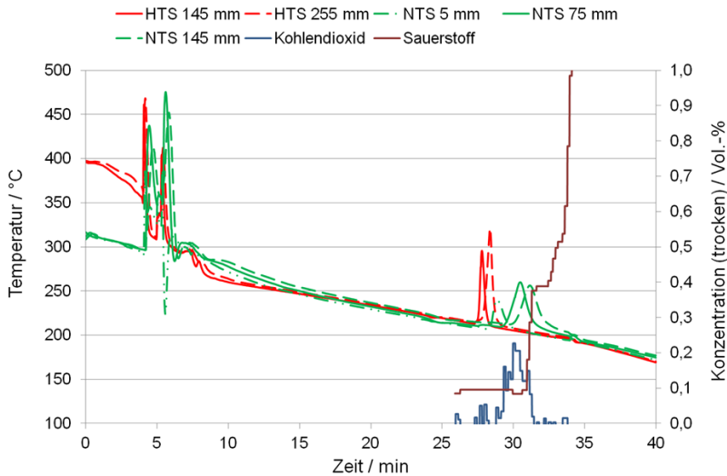
Abbildung 8.3: Temperaturspitzen im Wassergas-Shift-Reaktor während des Abfahrens des Systems und der anschließenden Regeneration mit 80 l N /h Luft. Messwerte nach „Multigas™ 2030D“ und „Cirrus™ 2“.
