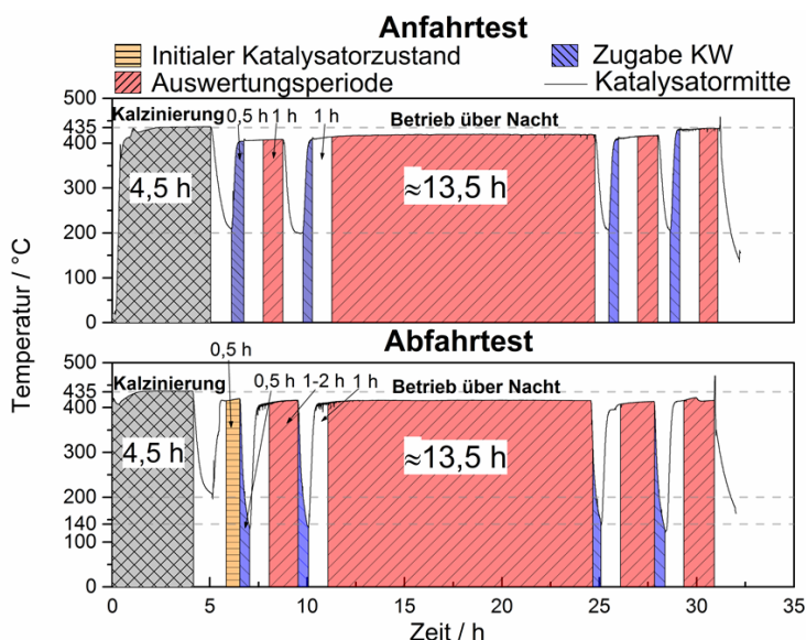
Abbildung 6.11: Testprozedur zur Identifikation kritischer Reformatkomponenten am Katalysator-Testreaktor.
