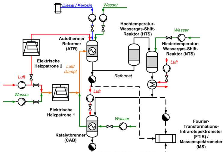
Abbildung 4.5: Fließbild des Systemteststands für Package 4.
