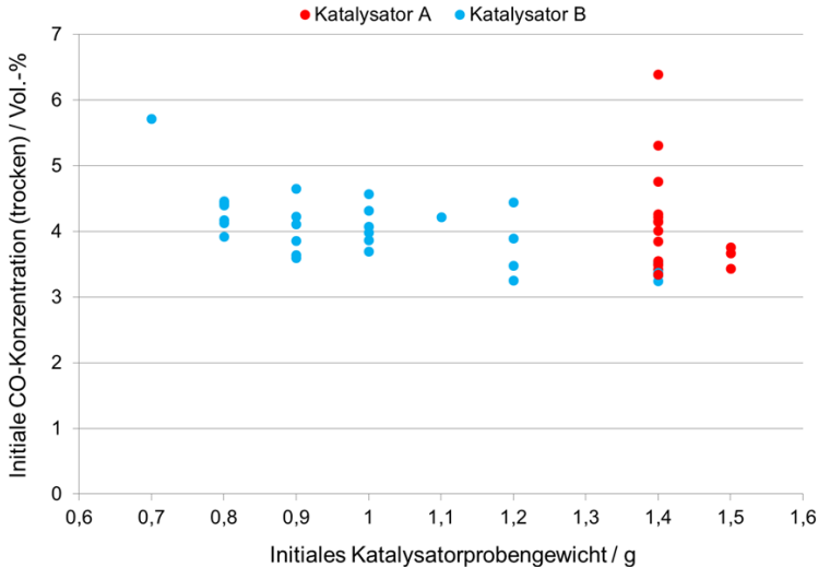
Abbildung 15.9: Probenvariabilität der Katalysatoren A und B. Aufgetragen ist die initial gemessene CO-Konzentration in Abhängigkeit des gemessenen Probengewichts.
