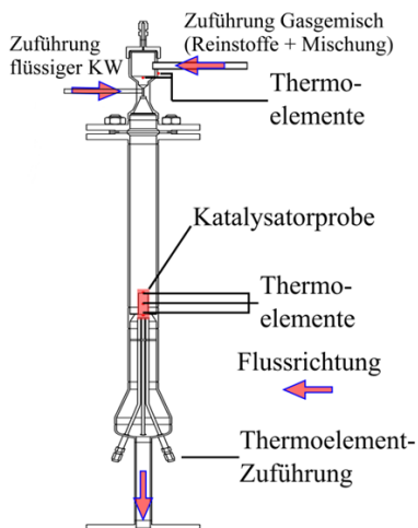
Abbildung 4.2: Schnittzeichnung des Katalysator-Testreaktors.
