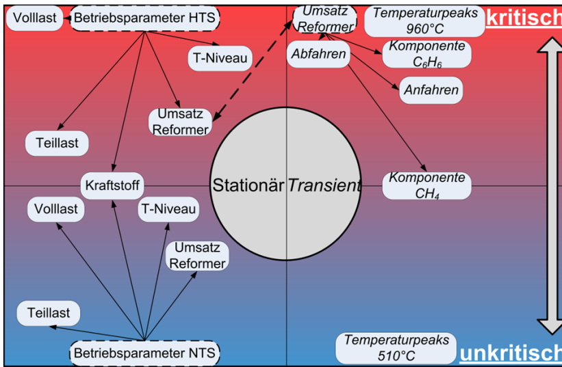
Abbildung 5.11: Übersicht der identifizierten, potentiell kritischen Parameter für den Betrieb des WGS-Reaktors unter stationären und transienten Bedingungen.
