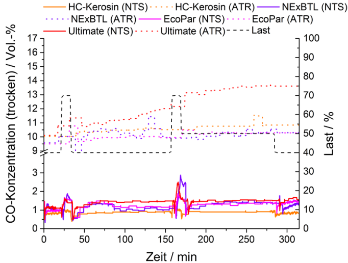
Abbildung 8.11: CO-Konzentrationen hinter dem NTS-Reaktor und dem ATR für alle vier Kraftstoffe bei dem Profil „Lutsey Modi Einfach“. Messwerte nach „Multigas TM 2030D“ und „Cirrus TM 2“.
