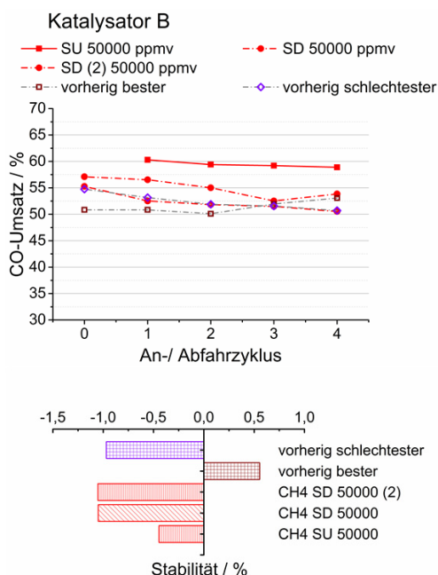
Abbildung 6.12: Einfluss von CH 4 auf die Stabilität von Katalysator B während des An- und Abfahrens (SU=startup, SD=shutdown). Messwerte nach „Multigas™ 2030D“ und „Cirrus™ 2“.
