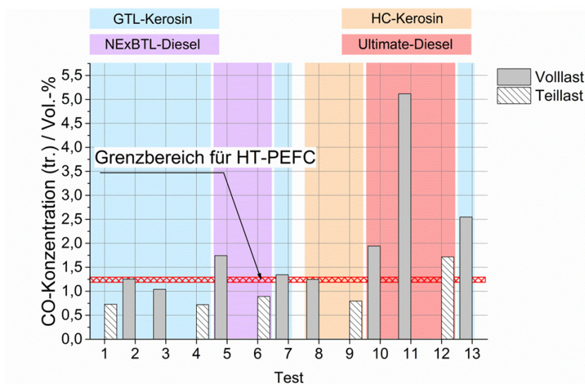
Abbildung 5.1: Kohlenmonoxidkonzentration (trocken) am Austritt des Wassergas-Shift-Reaktors über Versuchssreihe Package 2, Teil 1. Messwerte nach „Prima 600 S“. Nachgebildet aus [160] mit Genehmigung von ECS – The Electrochemical Society.
