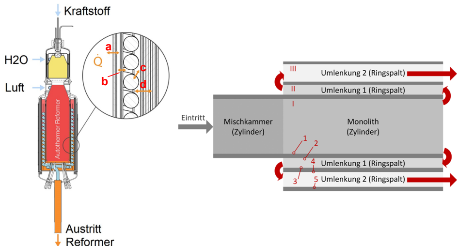
Abbildung 4.9: Abstraktion der Geometrie des autothermen Reformers ATR 9.2 und berechnete Wärmeübergänge im Modell.
