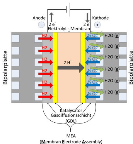
Abbildung 2.2: Funktionsweise einer Brennstoffzelle am Beispiel einer HT-PEFC, nach [50].
