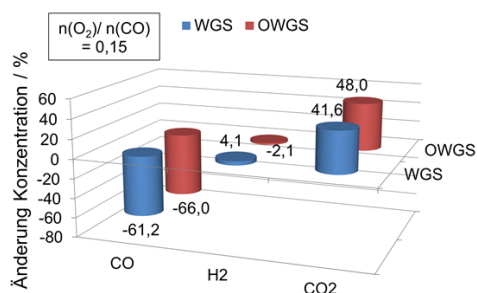
Abbildung 7.7: Durchschnittliche Änderung der Konzentrationen an \text{CO} , \text{H}_2 und \text{CO}_2 während des WGS- und OWGS-Betriebs mit Katalysator B. Es wurden HTS-Bedingungen und ein molares \text{O}_2/\text{CO} -Verhältnis von 0,15 gewählt. Messwerte nach „Multigas™ 2030D“ und „Cirrus™ 2“.
