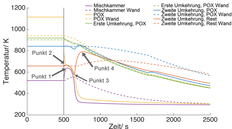
Abbildung 15.16: Fluid- und Wandtemperaturen im autothermen Reformier während des Abfahrvorgangs. Als Spülmedium wurde Wasserdampf mit 10000 g/h gewählt. Nach T_{krit} wurden 20000 l/h Luft dem Reformier zugegeben.
