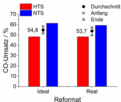
Abbildung 6.8: Einfluss der Reformatqualität auf die Katalysatoraktivität. Messwerte nach „Prima 600 S“ und „Multigas™ 2030D“ und „Cirrus™ 2“.
