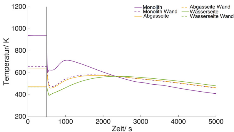
Abbildung 15.21: Fluid- und Wandtemperaturen im Katalytbrenner während des Abfahrvorgangs. Als Spülmedium wurde Luft/ Wasserdampf mit 10000 l N /h Luft und 10000 g/h Wasserdampf gewählt. Nach T_{krit} wurde die Wasserdampfzufuhr unterbunden.
