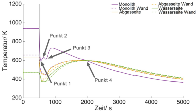
Abbildung 15.18: Fluid- und Wandtemperaturen im Katalytbrenner während des Abfahrvorgangs. Als Spülmedium wurde Wasserdampf mit 10000 g/h gewählt. Nach T_{krit} wurden 20000 l/h Luft dem Reformier zugegeben.
