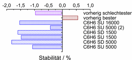
Abbildung 6.14: Einfluss von C_6H_6 auf die Stabilität von Katalysator B während des An- und Abfahrens (SU=startup, SD=shutdown). Messwerte nach „Multigas™ 2030D“ und „Cirrus™ 2“.
