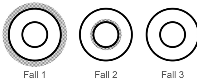
Abbildung 15.7: Fallunterscheidung bei der Wärmeübertragung am konzentrischen Ringspalt. Fall 1: Wärme­übertragung am Innenrohr, Außenrohr wärmege­dämmt; Fall 2: Wärmeübertragung am Außen­rohr, Innenrohr wärmege­dämmt; Fall 3: Wärmeübertragung an beiden Rohren, nach [150].
