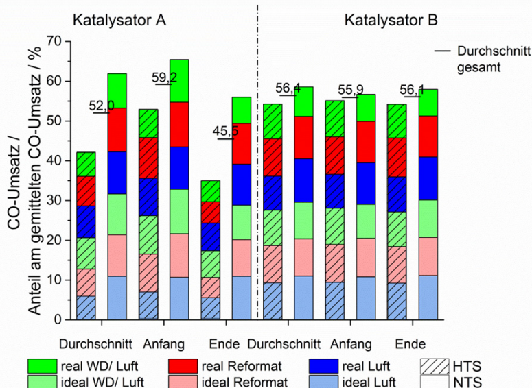
Abbildung 6.10: Unterschiedliche Aktivität/ Stabilität der Katalysatoren A und B. Messwerte nach „Prima 600 S“ und „Multigas™ 2030D“ und „Cirrus™ 2“.
