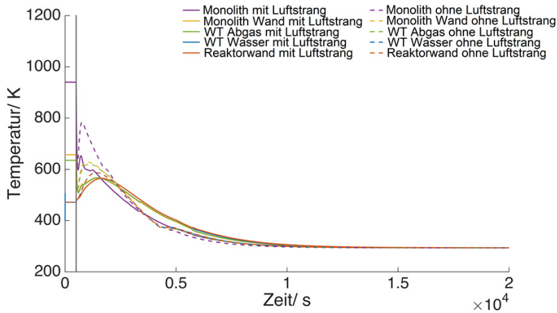
Abbildung 15.23: Verbesserung (a): kurze Abfahrdauer. Temperaturverläufe im Katalytbrenner. Im Fall mit zusätzlichem Luftstrang wurde zunächst mit 10000 l N /h Luft und 500 g/h Wasserdampf gespült. Nach T_{krit} wurden zusätzlich 10000 l N /h Luft hinzugegeben. Im Fall ohne zusätzlichen Luftstrang wurde von Anfang an mit 20000 l N /h Luft und 500 g/h Wasserdampf gespült. Nach T_{krit} wurde die Wasserzufuhr gestoppt.
