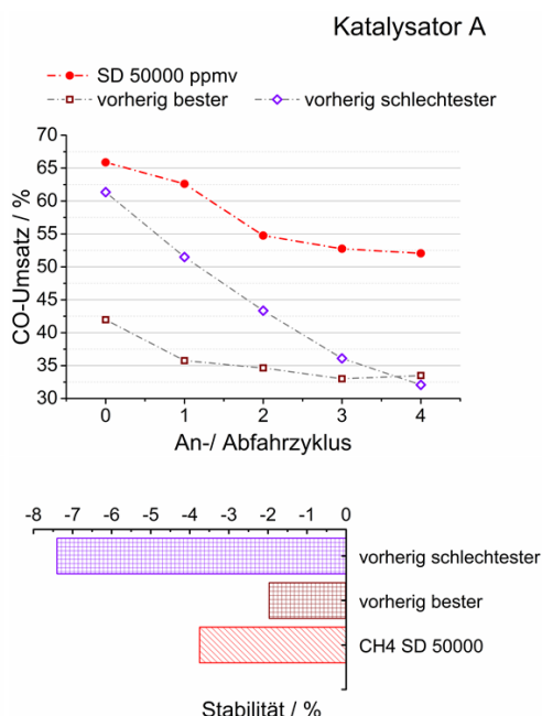
Abbildung 6.13: Einfluss von CH 4 auf die Stabilität von Katalysator A während des An- und Abfahrens (SU=startup, SD=shutdown). Messwerte nach „Multigas™ 2030D“ und „Cirrus™ 2“.
