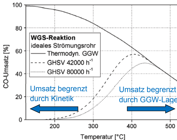
Abbildung 2.7: Gleichgewichtslage (GGW) und angepasste S-Kurven für ein ideales Strömungsrohr bei unterschiedlichen Raumgeschwindigkeiten in Abhängigkeit von der Temperatur [11]. Nachgebildet aus [63] mit Genehmigung von Elsevier.
