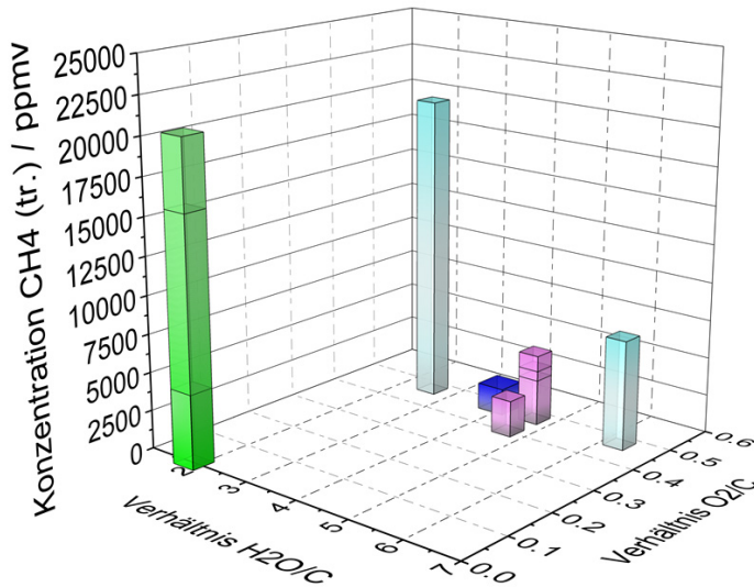
Abbildung 15.14: Maximalkonzentrationen von \text{CH}_4 während des Abfahrens des Systems mit NExBTL. Farben: grün: klassische Strategie; blau: neue Strategie 1; magenta: neue Strategie 2; cyan: neue Strategie 3.
