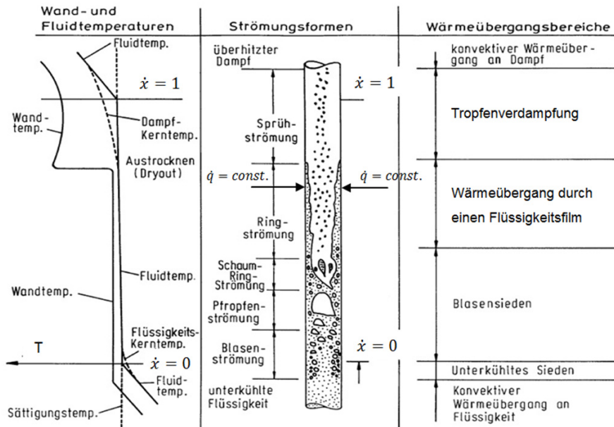
Abbildung 15.8: Wand- und Fluidtemperaturen, Strömungsformen und entsprechende Wärmeübergangsbereiche bei einem vertikal aufwärts durchströmten Rohr, nach [151].
