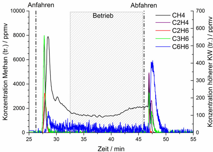
Abbildung 5.9: Beispiel für die unterschiedlichen Konzentrationen an Methan und höheren Kohlenwasserstoffen während des Anfahrens, des stationären Betriebs und des Abfahrens. Messwerte nach „Mulltigas™ 2030D“ und „Cirrus™ 2“. Nachgebildet aus [162] mit Genehmigung von Elsevier.
