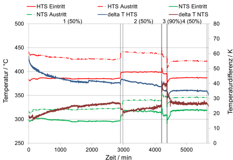
Abbildung 8.1: WGS-Temperaturen während des 100 h-Versuchs mit Katalysator B und NExBTL-Diesel.
