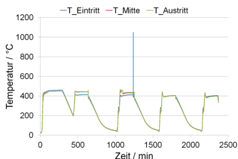
Abbildung 6.20: Vollständige Deaktivierung von Katalysator A durch eine kurzzeitige Temperaturspitze bis 1048 °C.
