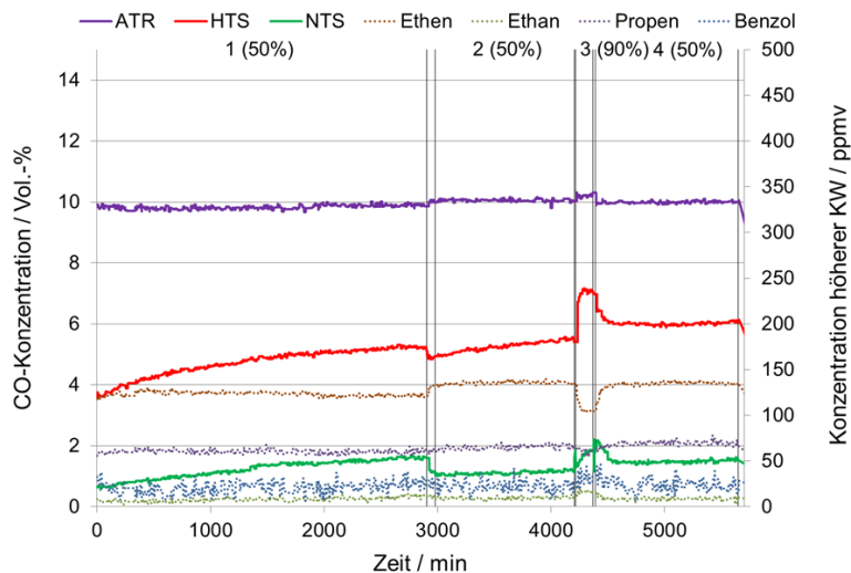
Abbildung 8.2: Konzentrationen von CO und höherer Kohlenwasserstoffe (ATR) während des 100 h-Versuchs mit Katalysator B und NExBTL-Diesel. Messwerte nach „Multigas™ 2030D“ und „Cirrus™ 2“.
