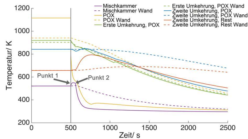
Abbildung 15.19: Fluid- und Wandtemperaturen im autothermen Reformer während des Abfahrvorgangs. Als Spülmedium wurde Luft/ Wasserdampf mit 10000 l N /h Luft und 10000 g/h Wasserdampf gewählt. Nach T_{krit} wurde die Wasserdampfzufuhr unterbunden.
