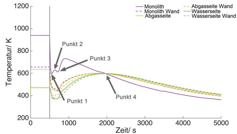
Abbildung 15.18: Fluid- und Wandtemperaturen im Katalytbrenner während des Abfahrvorgangs. Als Spülmedium wurde Wasserdampf mit 10000 g/h gewählt. Nach T_{krit} wurden 20000 l N /h Luft dem Reformer zugegeben.
