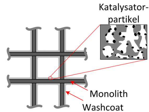
Abbildung 3.2: Monolith, Washcoat und Partikel eines Katalysators, nach [72].
