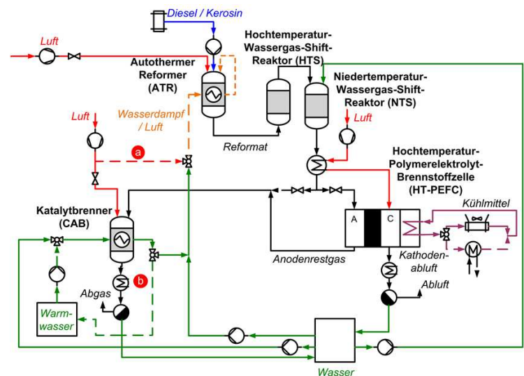
Abbildung 9.5: Fließbild des Brennstoffzellensystems des IEK-3 mit den Verbesserungen (a) kurze Abfahrdauer und (b) Energierückgewinnung.
