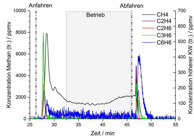
Abbildung 5.9: Beispiel für die unterschiedlichen Konzentrationen an Methan und höheren Kohlenwasserstoffen während des Anfahrens, des stationären Betriebs und des Abfahrens. Messwerte nach „Muiltigas™ 2030D“ und „Cirrus™ 2“. Nachgebildet aus [162] mit Genehmigung von Elsevier.
