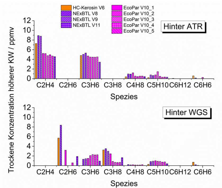
Abbildung 5.5: Unterschiedliche Konzentrationen höherer Kohlenwasserstoffe hinter dem Reformer und dem Wassergas-Shift-Reaktor bei stationärem Betrieb. Messwerte nach „HP 6890 Series“ und „HP G1099A“. Nachgebildet aus [160] mit Genehmigung von ECS – The Electrochemical Society.
