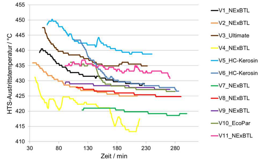
Abbildung 5.6: Profil der HTS-Austrittstemperatur innerhalb der ersten drei Betriebsstunden.
