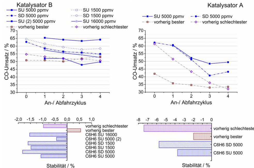
Abbildung 6.14: Einfluss von C 6 H 6 auf die Stabilität von Katalysator B während des An- und Abfahrens (SU=startup, SD=shutdown). Messwerte nach „Multigas™ 2030D“ und „Cirrus™ 2“.
