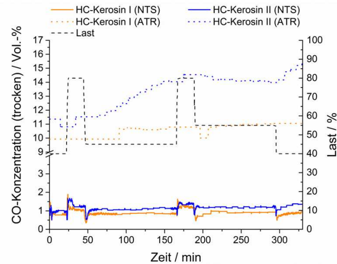
Abbildung 8.13: CO-Konzentrationen hinter dem NTS-Reaktor und dem ATR für die Versuche „HC-Kerosin I“ und „HC-Kerosin II“ bei dem Profil „Lutsey Modi Mittel“. Messwerte nach „Multigas™ 2030D“ und „Cirrus™ 2“.
