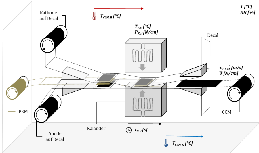
Abbildung 3.2: Schematische Darstellung des prozessualen Parameterraums für die indirekte Fertigung der CCM durch das Decalverfahren. Der gesamte Prozess steht unter dem Einfluss von Schwankungen in der klimatischen Fertigungsumgebung
