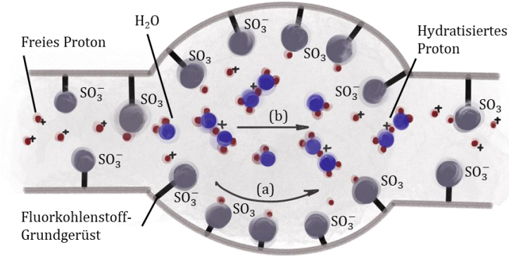
Abbildung 2.5: Schematische Darstellung der Protonenleitung in der PEM (vgl. [38])
