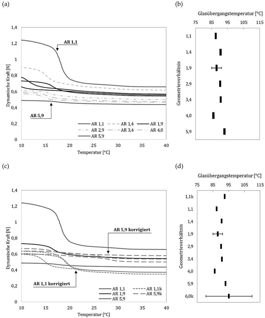
Abbildung 4.5: (a) CCM-Kraftantwort von Proben unterschiedlichen Geometrieverhältnisses auf die sinusförmige Anregung mit der konstanten Amplitude von 25 µm; (c) CCM-Kraftantwort von Proben unterschiedlichen Geometrieverhältnisses auf die sinusförmige Anregung mit einer angepassten Amplitude, die eine gleichwertige Dehnung der Proben zu (a) gewährleistet; (b) und (d) Variation der Probengeometrie besitzt keine Auswirkung auf den Glasübergang der CCM, der basierend auf dem lokalen Maximum von \tan \delta -Kurve mit einer Frequenz 1 Hz und Aufheizrate 1 K/min bestimmt wird
