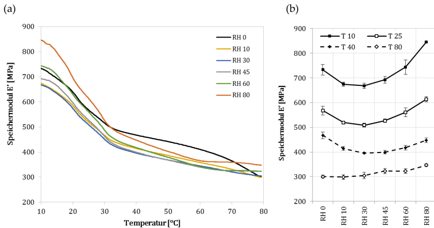
Abbildung 5.6: Auswirkung der beiden Hauptfaktoren Temperatur und relativer Feuchte auf das Speichermodul der Referenz-CCM bis 80°C und 80%. Der thermische Verlauf des (a) Speichermoduls und die (b) detaillierte Aufschlüsselung auf Isothermen dienen als Erweiterung und Bestätigung der Signifikanzberechnung im Rahmen der statistischen Versuchsplanung
