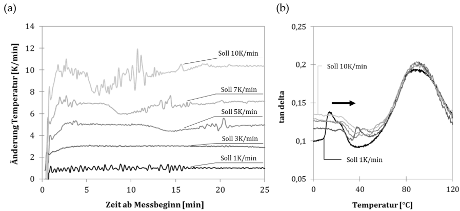
Abbildung 4.8: (a) Zeitlicher Bedarf ab Messbeginn für die schwankungsfreie Regelung der DMA-Heizrate bis 10 K/min; (b) Auswirkung der Heizrate auf das \tan \delta -Verhalten der Referenz-CCM im Temperaturbereich von 0 °C bis 120 °C (Geometrieverhältnis 2,0; Amplitude 25 \mu\text{m} ; Frequenz 1 Hz)
