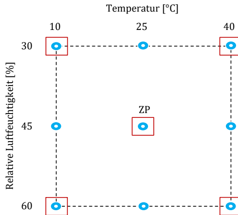
Abbildung 4.3: ●: Quantitativer Modellansatz zur Bestimmung nichtlinearer mechanischer DMA-Eigenschaften anhand eines vollfaktoriellen Versuchsplans mit den zwei Faktoren Temperatur und relativer Feuchte auf jeweils drei Stufen. □: Nachstellung der Faktorstufenkombinationen mit mechanisch/optischem Prüfaufbau in Klimaschrank, jedoch ohne mathematische Modellierung der Ergebnisse (siehe Abschnitt 4.4.1)
