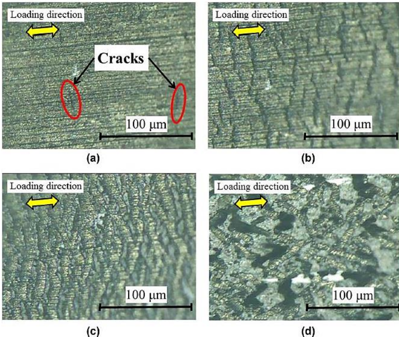
Abbildung 3.10: Darstellung einer Elektrodenoberfläche bei Raumbedingungen 25°C und 50% relativer Feuchte mit Dehnung (a) \varepsilon = 0,07 , (b) \varepsilon = 0,1 , (c) \varepsilon = 0,5 und (d) \varepsilon = 1,0 [96]
