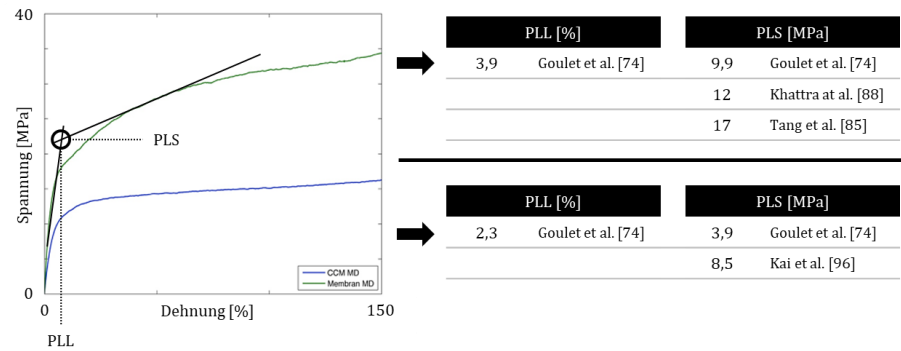
Abbildung 3.7: Spannungs-Dehnungskurve einer exemplarischen CCM/PEM. Im Übergang von elastischer zu plastischer Verformung können die mechanischen Kennwerte PLL/PLS im Schnittpunkt der jeweiligen Tangenten bestimmt werden
