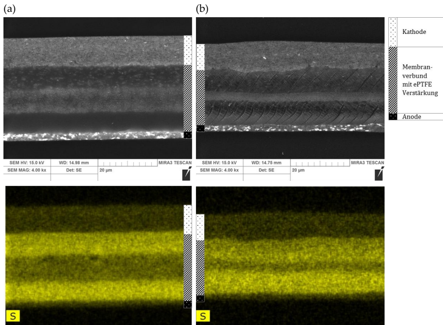
Abbildung 4.1: SE- und EDX-Darstellung der (a) Referenz-CCM mit Gore M735 Membran und (b) Vorserien-CCM. Die diagonalen Linien sind Artefakte der Erstellung von Böschungsschnitten mittels Ionoenmühle. Beide anoden- als auch kathodenseitigen reinen Ionomerschichten können durch den erhöhten Schwefelanteil in der spektralen Analyse identifiziert werden
