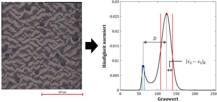
Abbildung 4.14: Kathodendarstellung einer 50%ig gestreckten Referenz-CCM durch das Alicona Infinite Focus Mikroskop. Das entsprechende Grauerthistogramm weist zwei lokale Maxima auf, deren Abstand als auch die jeweilige Halbwertsbreite in die quantitative Bewertung des Farbkanals durch Gl. 4.6 einfließen
