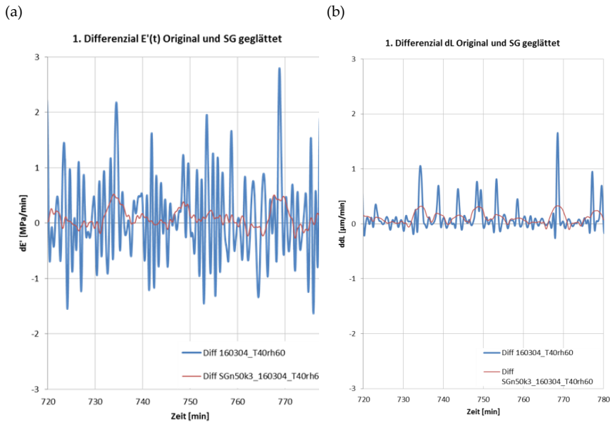
Abbildung 4.10: Glättung der ersten Ableitung der DMA-Rohsignale (a) Speichermodul E' und (b) Längenänderung anhand dem Savitzky-Golay-Verfahren (Fensterbreite 50, dritter Grad einer nichtlinearen Regression)
