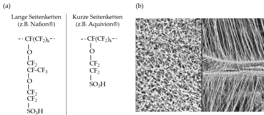
Abbildung 2.4: (a) Chemische Strukturunterschiede zwischen perfluorsulfonisierten Ionomeren mit langen (engl. long side chain, LSC) und kurzen (engl. short side chain, SSC) funktionalen Seitenketten; (b) Möglichkeiten der Streckung von PTFE dargestellt durch REM-Aufnahmen [37] (© 2008 from "Filtration and purification in the biopharmaceutical industry" by Meltzer, Theodore H. and Jornitz, Maik W.. Reproduced by permission of Taylor and Francis Group, LLC, a division of Informa plc.)
