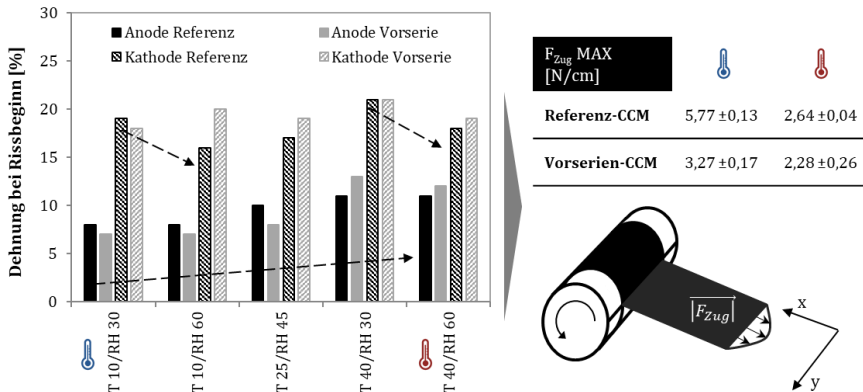
Abbildung 5.11: Rissbeginn auf den Elektrodenoberflächen der beiden CCM-Systeme in Abhängigkeit der Faktorstufenkombinationen. Mithilfe des Verlaufs der zum Beispiel benötigten Zugkraft im Gleichgewichtszustand der Relaxationsversuche, kann eine maximal zulässige Zugkraft bestimmt werden, für die keine Veränderung der Oberflächen stattfindet
