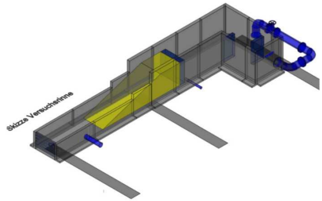
Abbildung 5: Versuchstand in der wasserbaulichen Versuchshalle des IWW.
