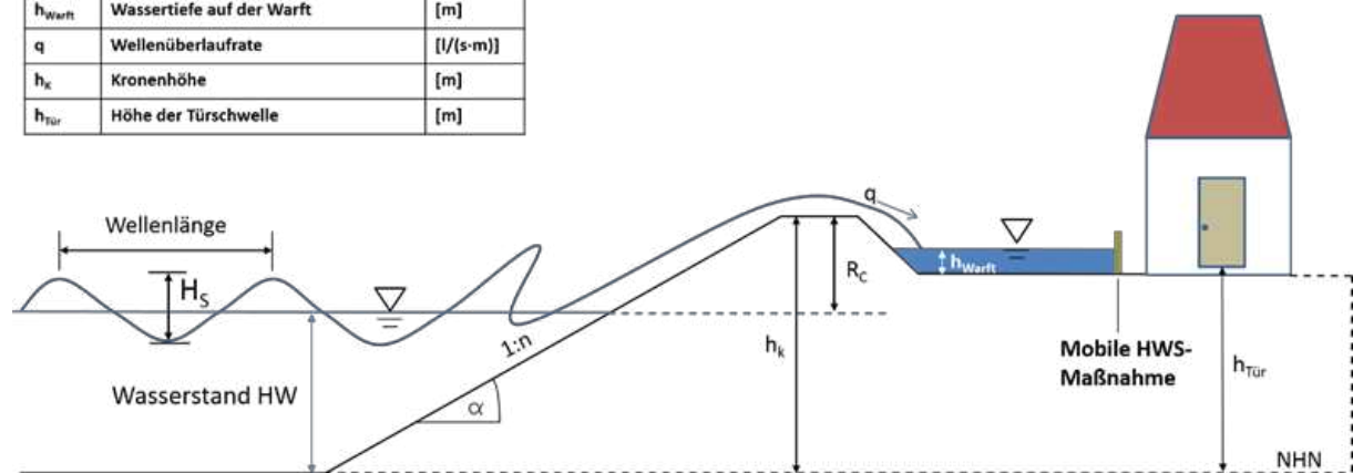
Abbildung 2: Mobile HWS-Maßnahme als Objektschutz im zentralen Warftbereich sowie geometrische und hydraulische Parameter an einer Warft (nach Wöffler und Schüttrumpf 2017).
