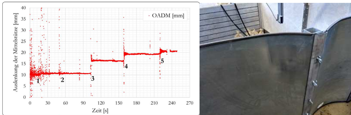
Abbildung 15: Auslenkung der Mittelstütze infolge Treibgutanprall an der Maßnahme HWS-mobil (ohne zusätzliche Abstützung) und Verformungen am Stahlblech nach Abschluss der Anprallversuche.
