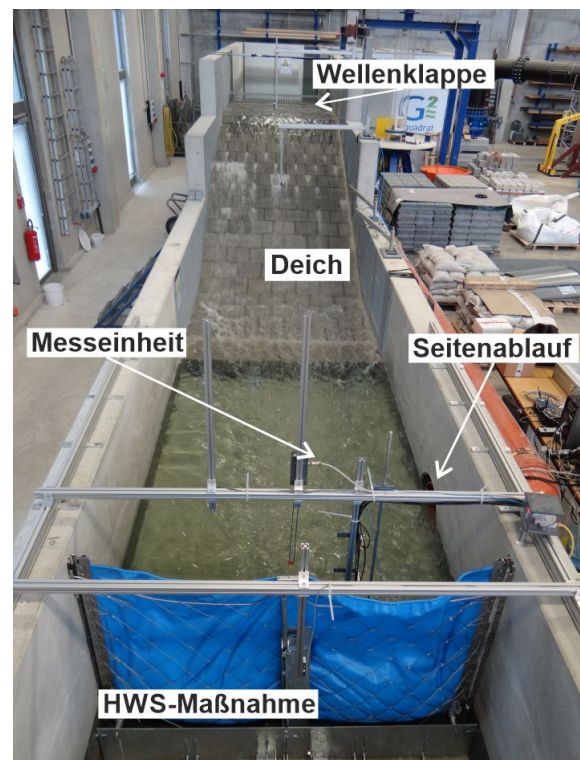
Abbildung 6: Versuchstand (links: Blickrichtung von Deichkrone, rechts: polderseitiger Blick).
