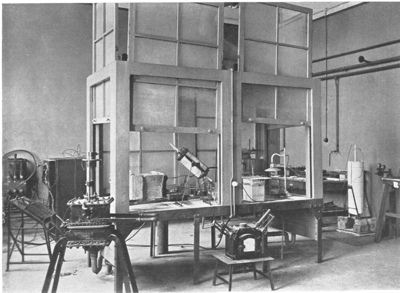
Kleines elektrisches Schmelzlaboratorium.
