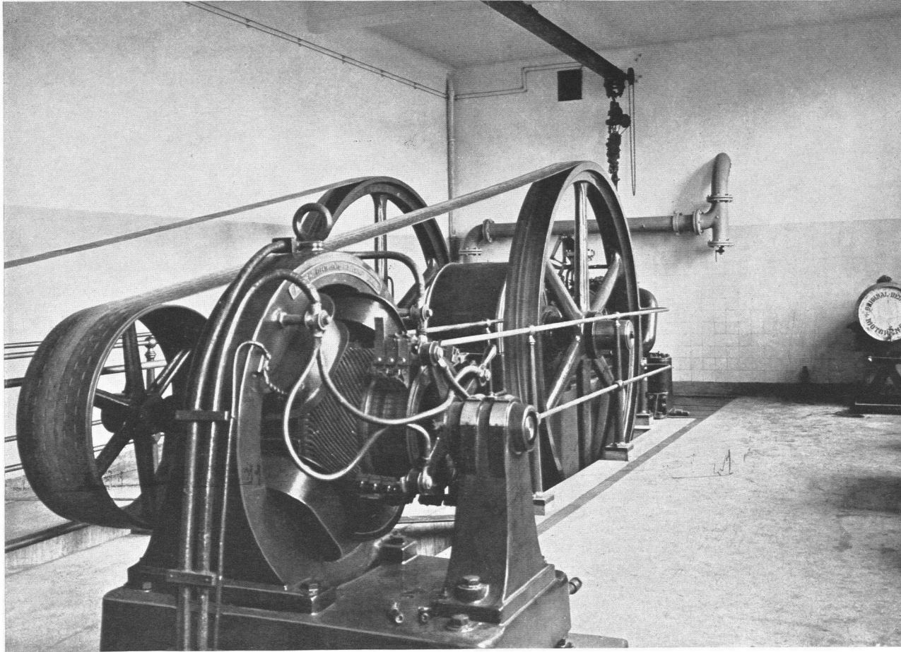
Gasmotor mit Dynamos (40 KW.).
