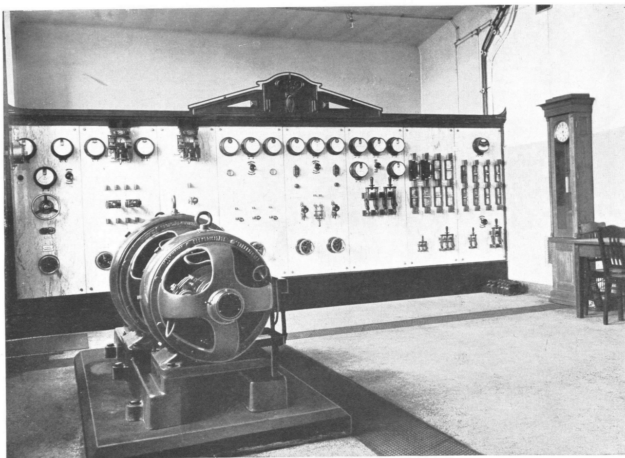
Hauptschalttafel. (Geschenk der Allgemeinen Elektrizitäts-Gesellschaft.)
