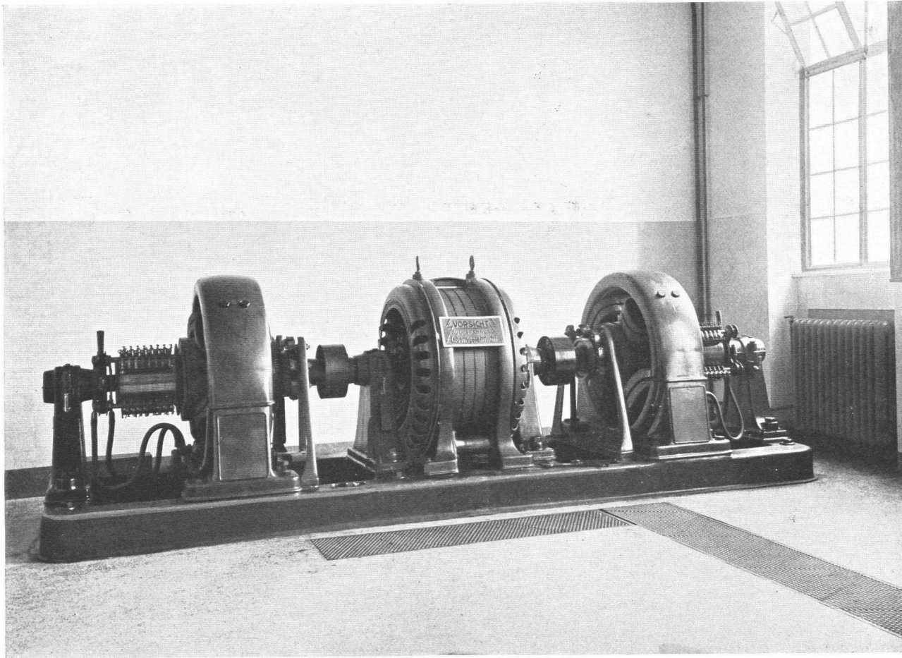
Transformator (120 KW.).
