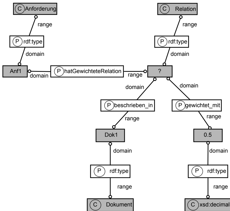
Abbildung 6.26: Verwendung einer Relationsklasse für n-äre Relationen
