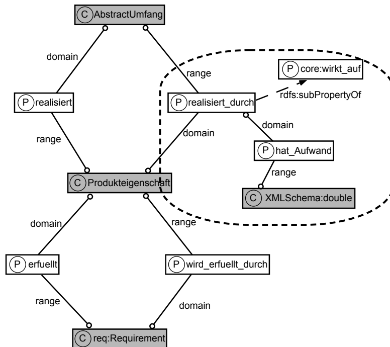
Abbildung 6.25: Gewichtungen von Eigenschaften zur automatisierten Kostenbetrachtung
