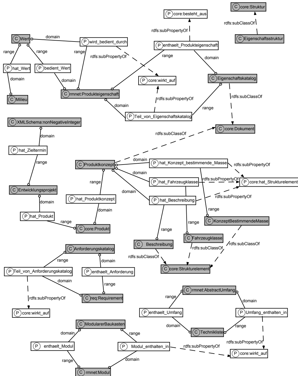
Abbildung 6.12: Eine graphische Repräsentation der Ontologie für die Produktentwicklung ohne Visualisierung der stark kreuzenden Relationen
