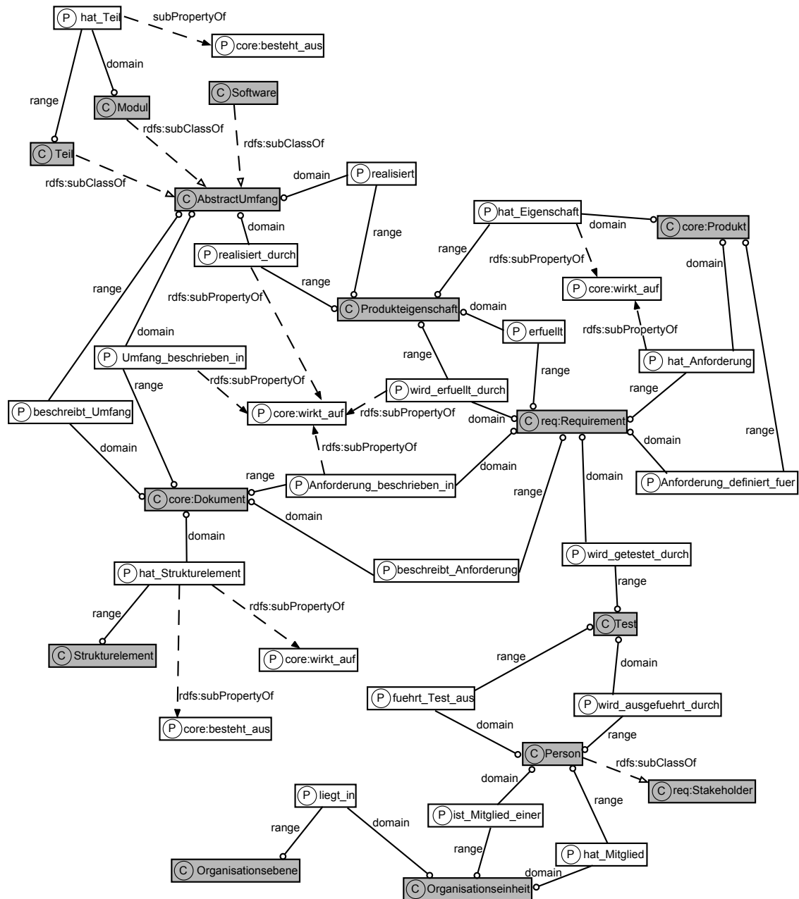
Abbildung 6.11: Eine reduzierte graphische Repräsentation der RMNet-Ontologie
