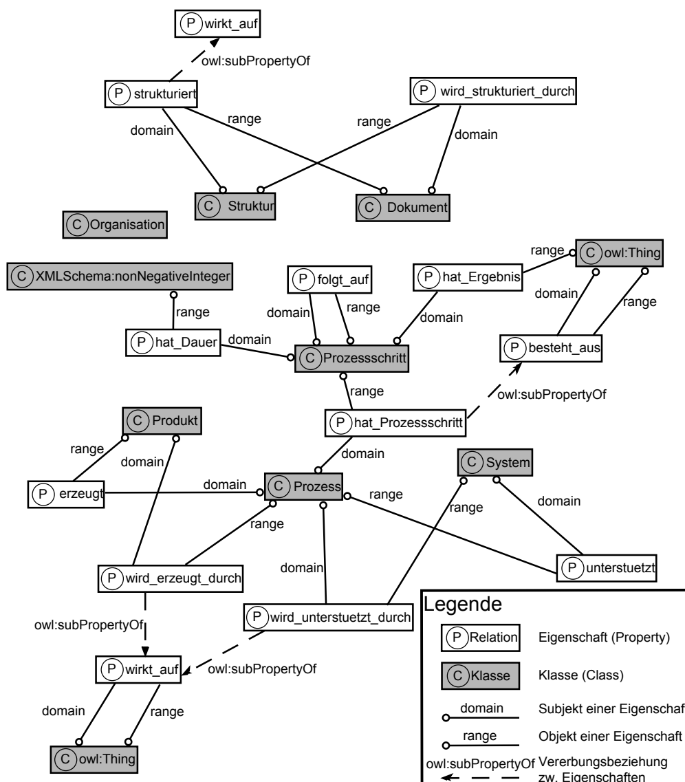
Abbildung 6.10: Eine graphische Repräsentation der Core-Ontologie
