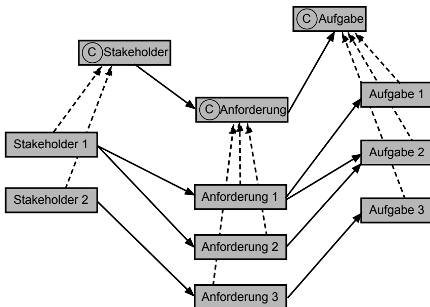
Abbildung 5.4: Ein simples Modell mit Instanzen von Projektartefakten
