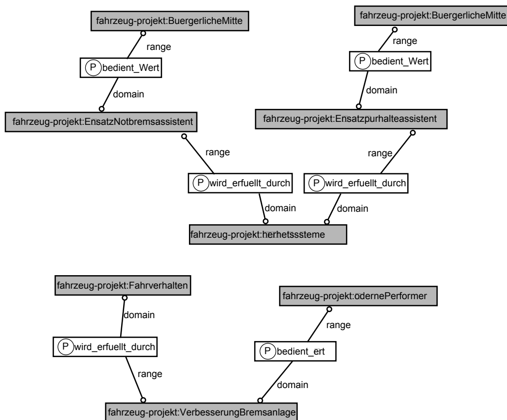
Abbildung 6.16: Darstellung der Zusammenhänge zwischen Milieus und Anforderungen.
