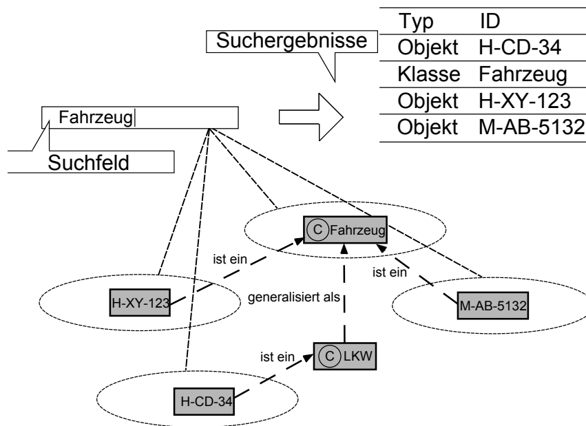
Abbildung 5.2: Suchen in Klassen und Objekten
