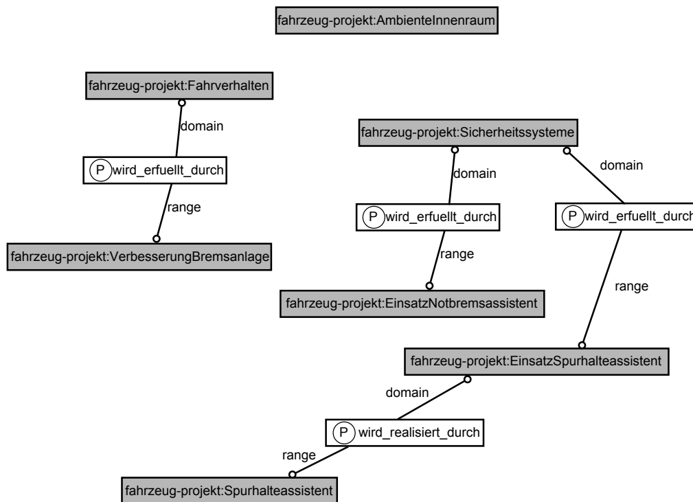
Abbildung 6.14: Eine graphische Repräsentation der SPARQL-Abfrage zum Reifegrad
