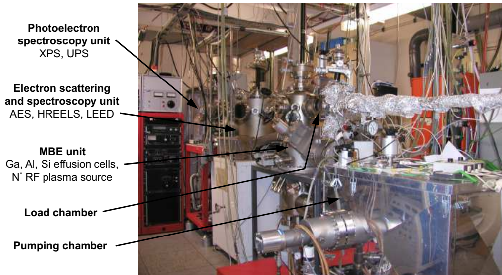
Figure 4.1: Picture of the MBE apparatus at the Institut für Schichten und Grenzflächen (ISG-1) of Forschungszentrum Jülich, used for the III-Nitride layer growth.
