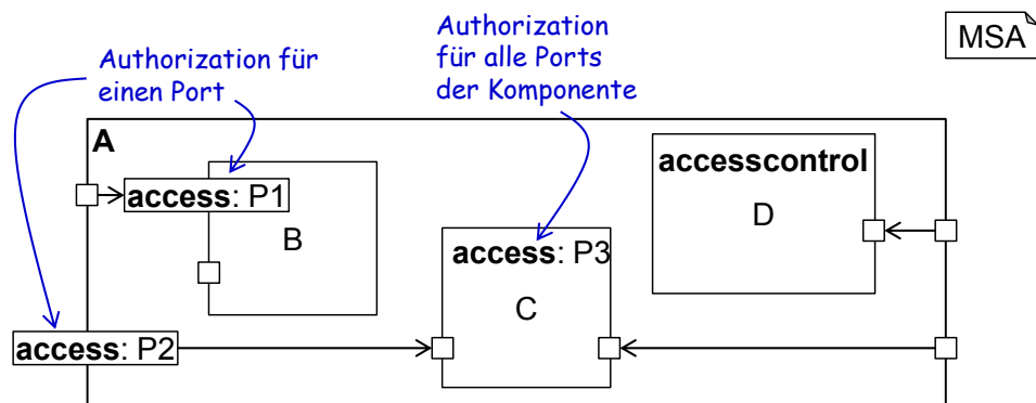
Abbildung 4.7.: Grafische Darstellung der Zugriffskontrolle.
