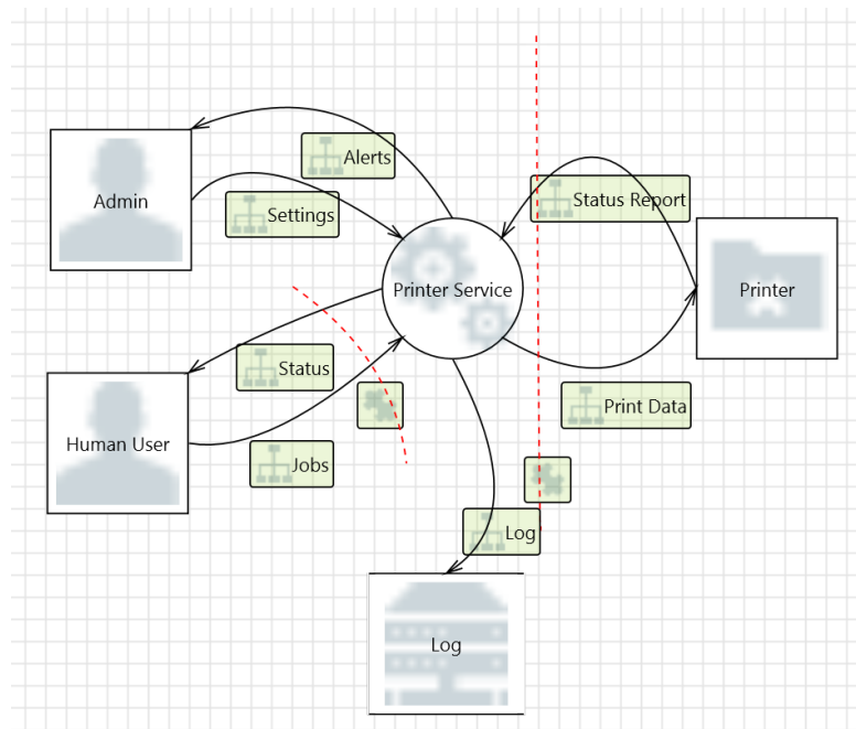
Abbildung 2.1.: Dieses Data Flow Diagram beschreibt die Datenflüsse zwischen einem Printer Service und seinen Nutzern.
