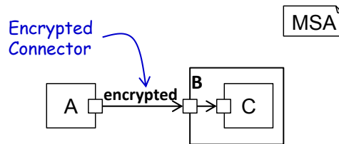
Abbildung 4.5.: Grafische Darstellung des Encrypted Connector.
