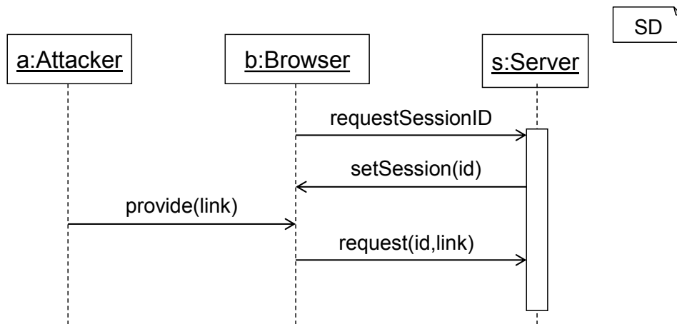
Abbildung 7.2.: Ablauf eines Cross-Site Request Forgery Angriffs.
