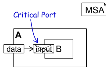
Abbildung 4.3.: Grafische Darstellung eines Critical Port.
