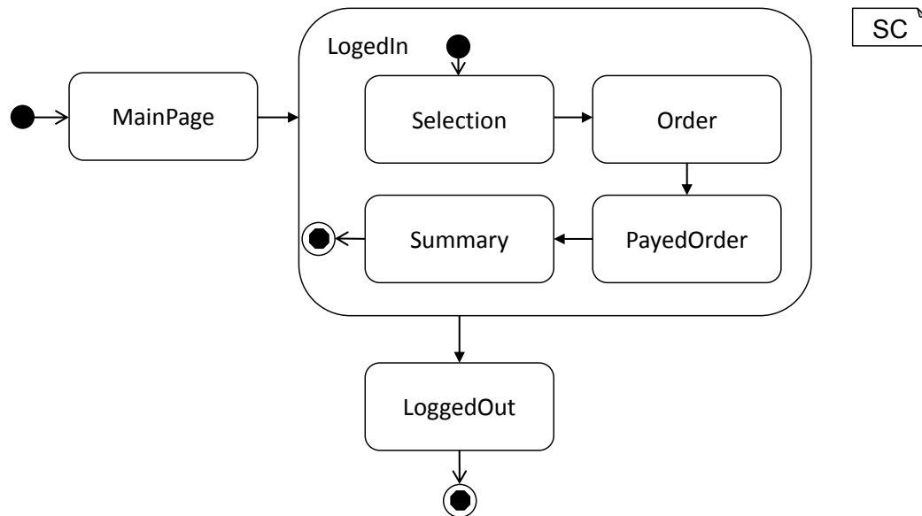
Abbildung 7.4.: Das Statechart beschreibt das Verhalten einer Webseite zur Pizzabestellung.
