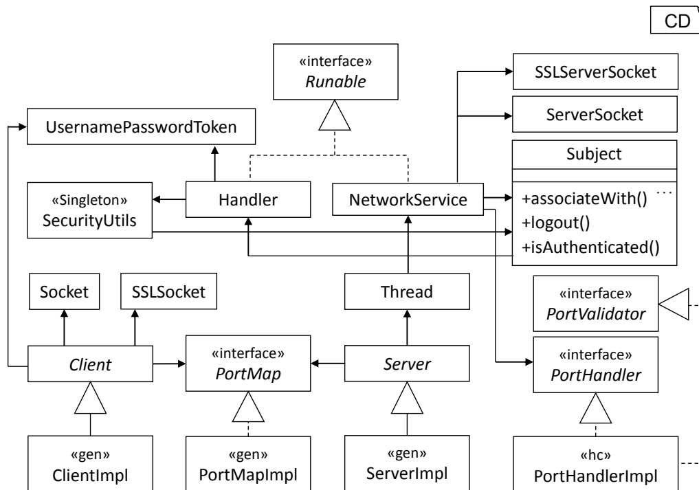
Abbildung 6.4.: Architektur der Java Implementierung.
