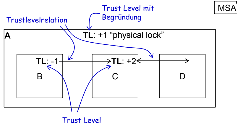
Abbildung 4.1.: Grafische Darstellung von Trustlevel und Trustlevelrelation.
