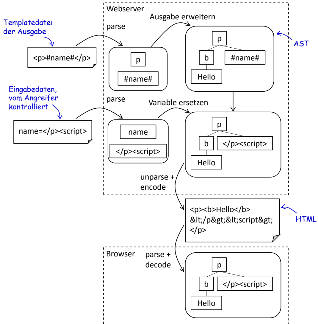
Abbildung 8.2.: Zeigt das Zusammenspiel von encoden und decoden bei der Übertragung eines HTML-Dokuments.
