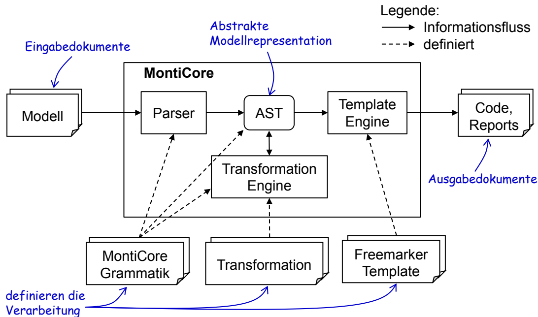
Abbildung 2.7.: Überblick über die Komponenten, Artefakte und Datenstrukturen von MontiCore.
