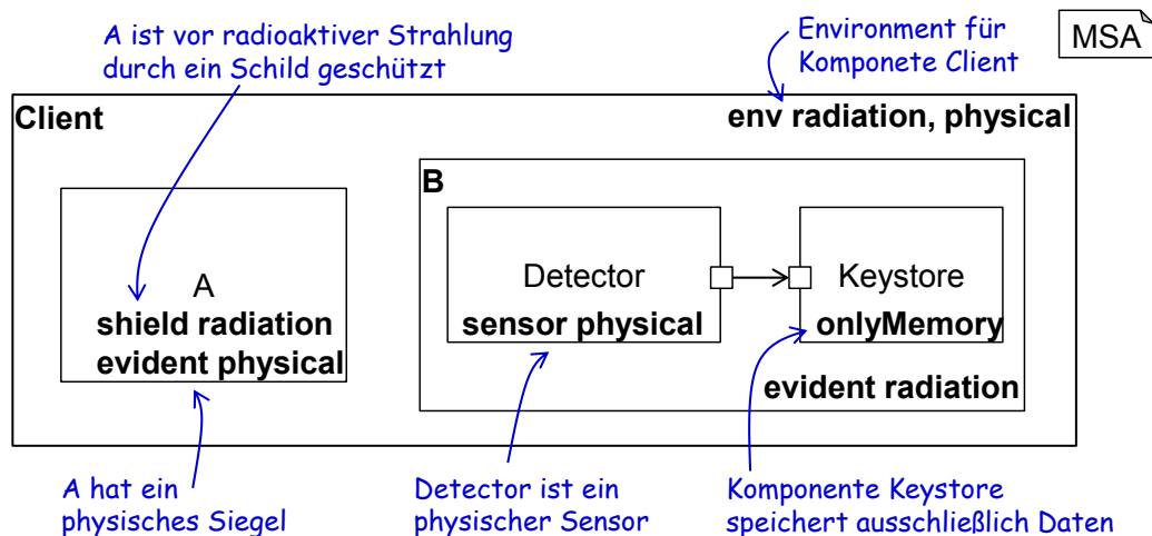
Abbildung 4.13.: Grafische Darstellung von physikalischen Kanälen und Schutzmaßnahmen.
