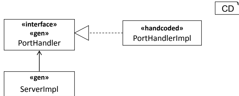
Abbildung 6.1.: Integration von handgeschriebenem Code in den generierten Server.
