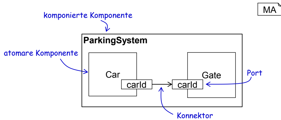
Abbildung 2.12.: Dieses graphische MontiArc Modell beschreibt genauso wie Listing 2.13 die Zufahrtsskontrolle eines Parkhauses.
