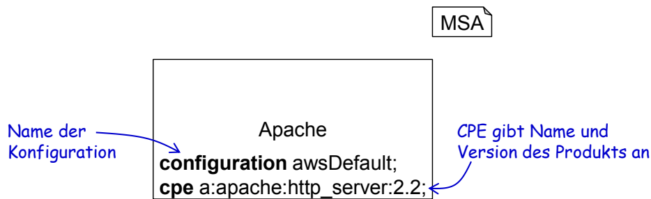
Abbildung 4.11.: Grafische Darstellung von Drittanbieterkomponenten.
