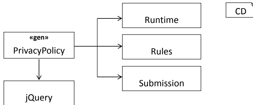
Abbildung 9.3.: Struktureller Zusammenhang in der Privacy Policy HTML Single-Page-Application.
