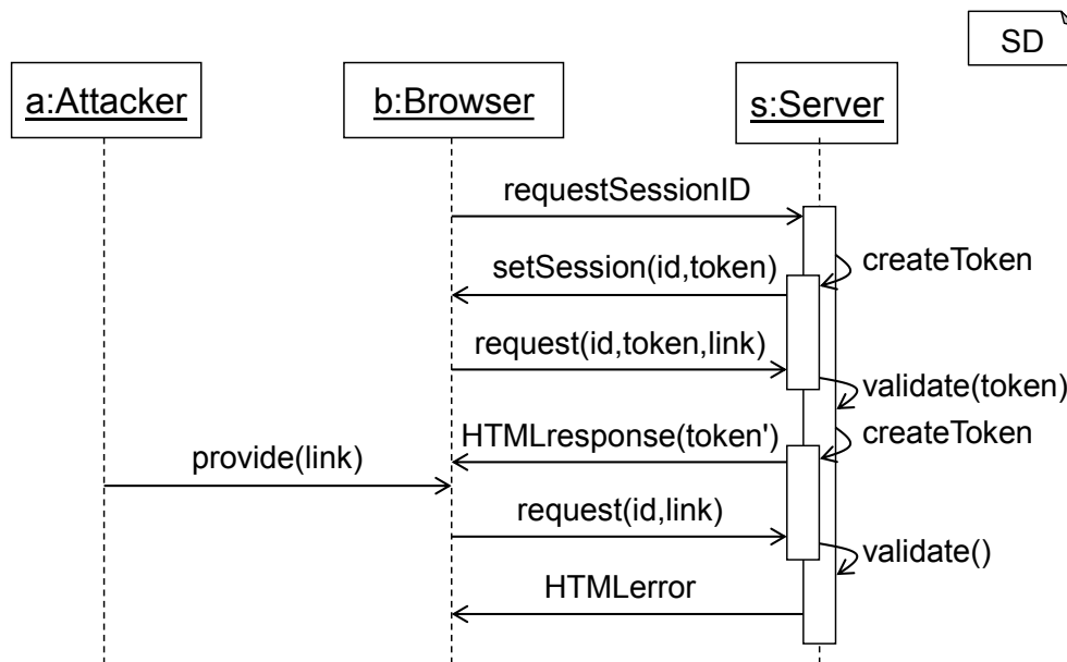
Abbildung 7.3.: Ablauf einer Anfrage mit CSRF-Token als Schutz gegen CSRF.
