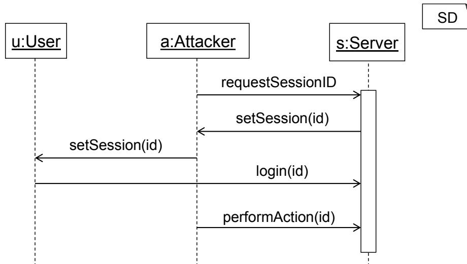
Abbildung 7.1.: Ablauf eines Session Fixation Angriffs.
