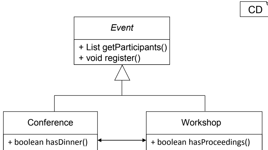
Abbildung 2.4.: Dieses Klassendiagramm in grafischer UML Darstellung beschreibt genau wie die textuelle Version in Listing 2.3 die Datenstruktur einer Konferenz.
