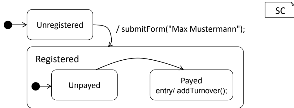
Abbildung 2.6.: Dieses Statechart in grafischer UML Darstellung beschreibt genau wie die textuelle Version in Listing 2.5 das Verhalten des Registrierungsprozess einer Konferenz.
