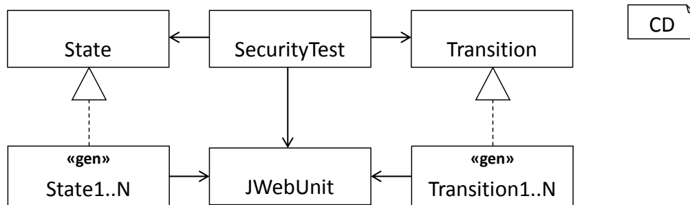
Abbildung 7.11.: Struktureller Aufbau der Security-Tests.
