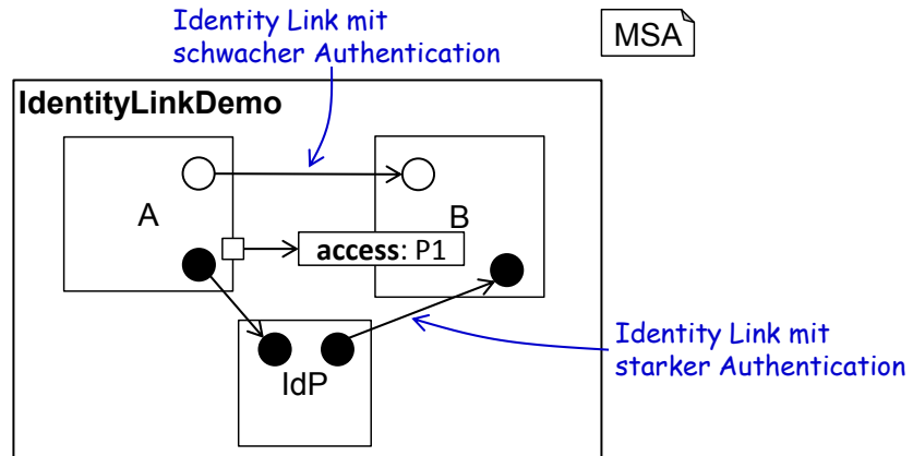
Abbildung 4.9.: Grafische Darstellung von identity Links.
