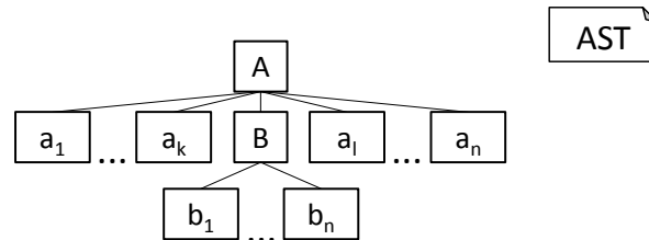
Abbildung 8.4.: Zeigt einen AST der Obersprache A, in dem A mit einer Untersprache B kombiniert wird.
