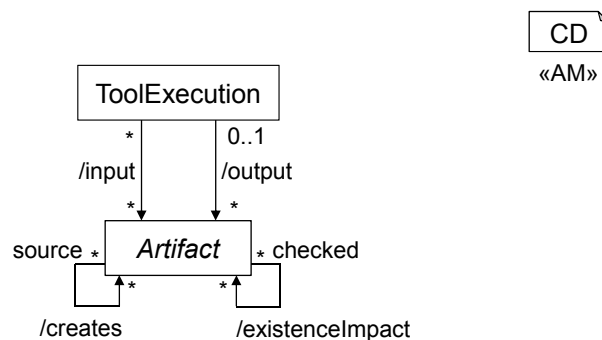
Abbildung 6.26.: Eingabe- und Ausgabeartefakte von Werkzeugausführungen.
