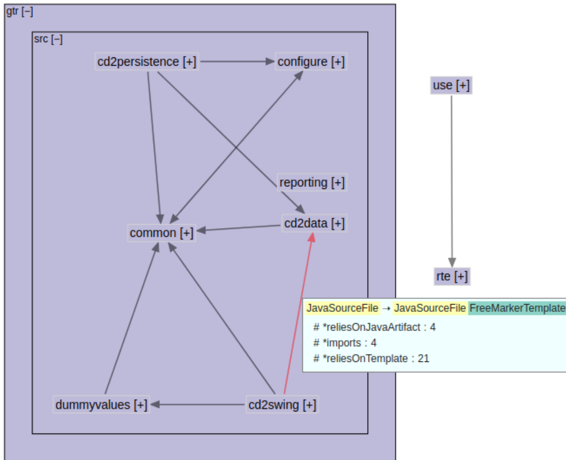
Abbildung 8.40.: Hierarchische Graphvisualisierung von Artefaktdaten mit ArtViz.
