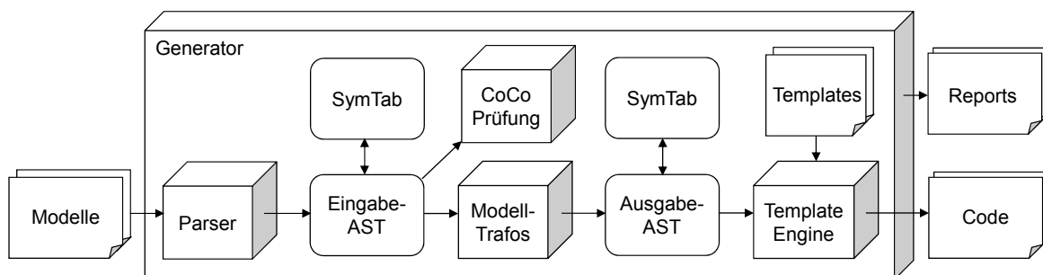
Abbildung 2.1.: Aufbau und Ablauf von MontiCore-basierten Generatoren.
