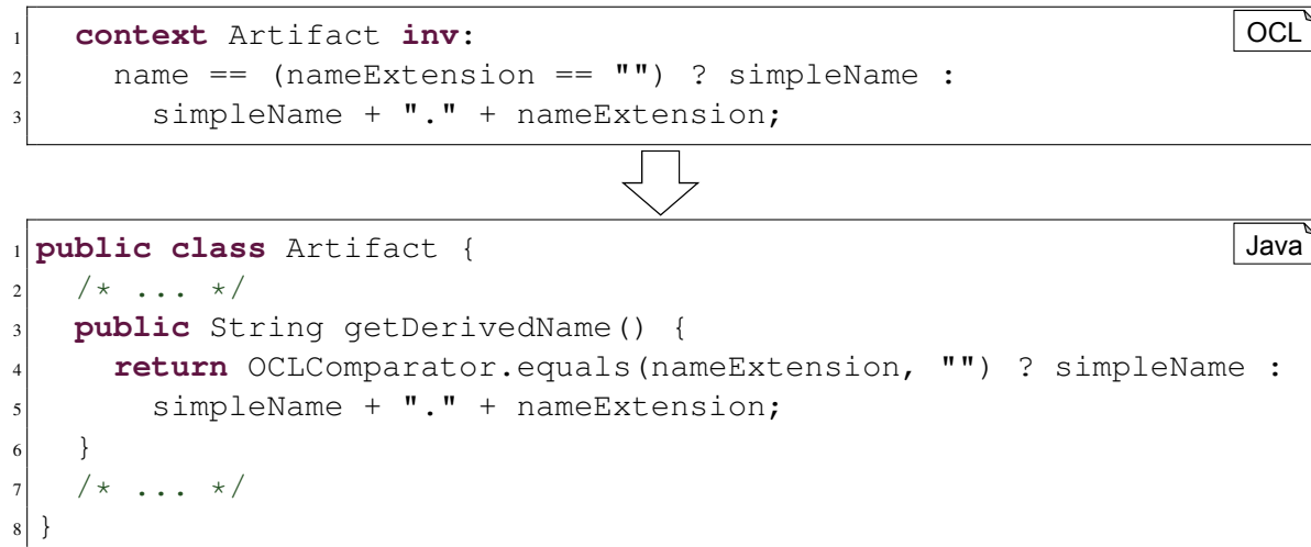
Abbildung 8.30.: Überführung einer OCL-Berechnungsvorschrift in eine Java-Methode zur Berechnung eines abgeleiteten Attributs (entnommen aus [Cuj17]).
