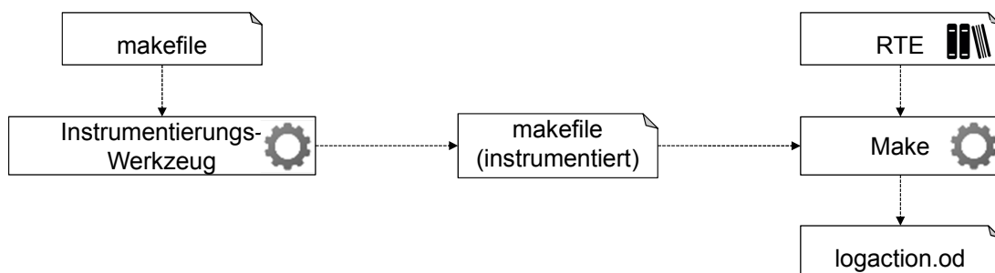
Abbildung 10.18.: Überblick über den Ansatz zur automatisierten Instrumentierung von Makefiles und dem Beobachten Make-basierter Buildprozesse.
