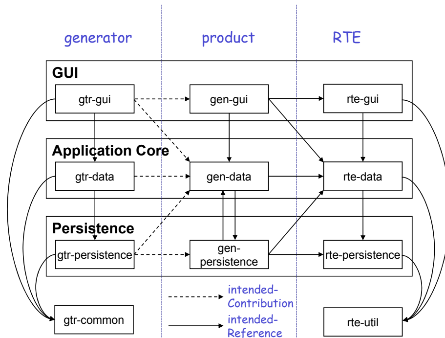
Abbildung 10.1.: Die Soll-Architektur des DEx-Projekts.
