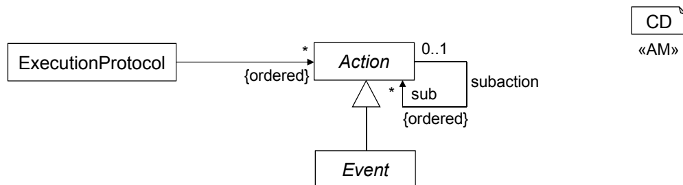
Abbildung 6.21.: Aktionen, Events und deren Beobachtung.
