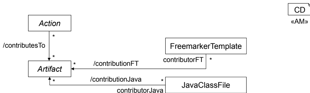
Abbildung 6.28.: Template- und Java-Arefakte tragen zur Erstellung von Artefakten bei.
