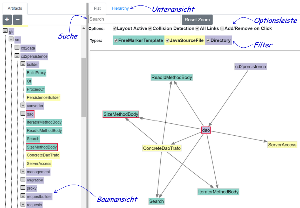
Abbildung 8.37.: Graph Visualisierung von Artefaktdaten mit ArtViz.
