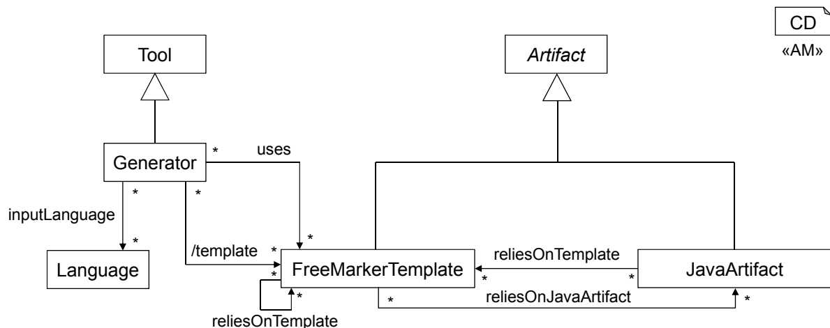
Abbildung 6.18.: Generatoren sind Werkzeuge, die zu den Eingabesprachen passende Modelle einlesen und unter anderem aus FreeMarker-Templates und Java-Artefakten bestehen.
