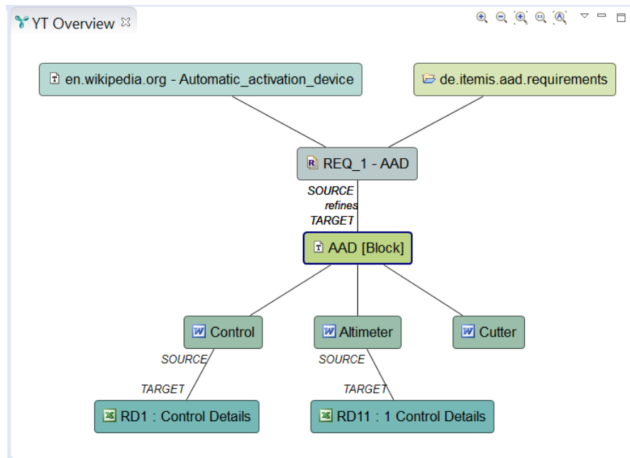
Abbildung 3.3.: Vertikale Traceabilityinformationen dargestellt als Graph unter Verwendung eines hierarchischen Layouts (entnommen von [Yak17b]).
