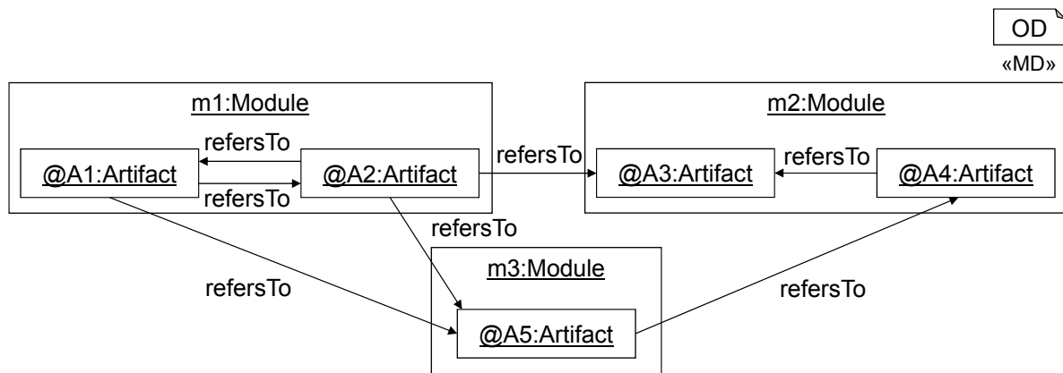
Abbildung 7.19.: Die Moduldefinition, zugeordnete Artefakte und deren Beziehungen, als Eingabe für die Berechnung der Ist-Architektur.
