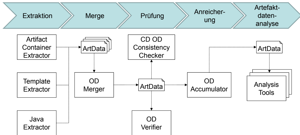
Abbildung 8.1.: Beispielhafte MontiArT-Instanz mit Zuordnung der Werkzeuge zu den Schritten der artefaktbasierten Analyse.
