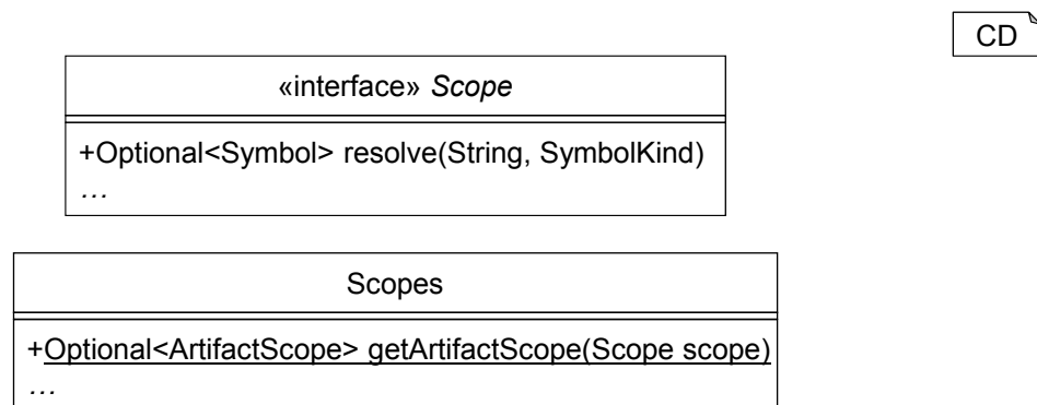
Abbildung 9.3.: Das Scope-Interface und die Scopes-Klasse.
