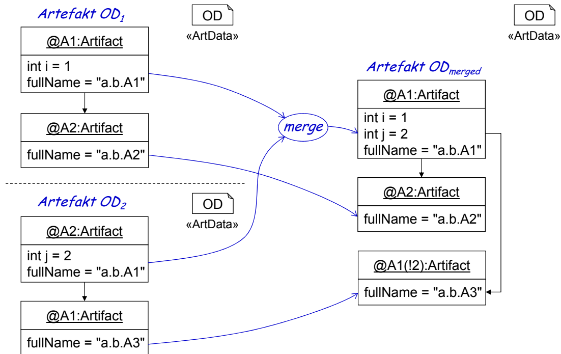
Abbildung 7.13.: Beispielhafte Durchführung des Mergealgorithmus unter Verwendung des fullname-Attributs als Zuordnungskriterium für Objekte.
