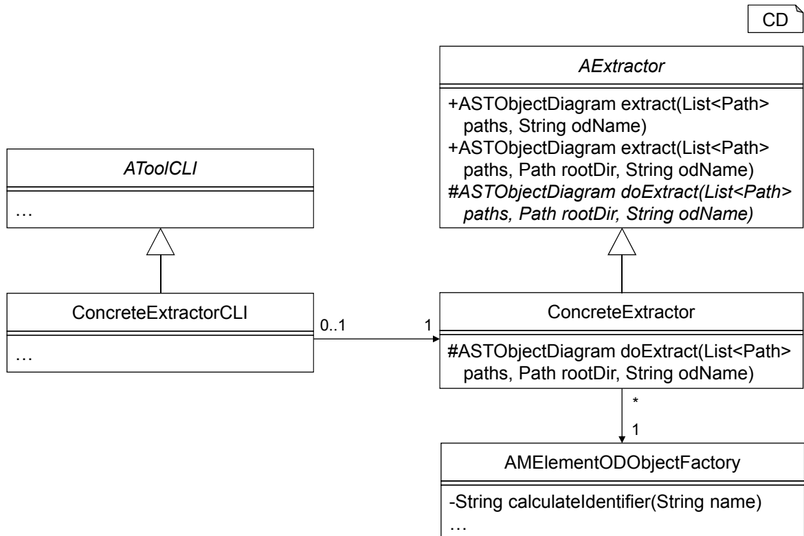
Abbildung 8.10.: Schematische Darstellung der Klassenstruktur der konkreten, statischen MontiArT-Extraktoren.
