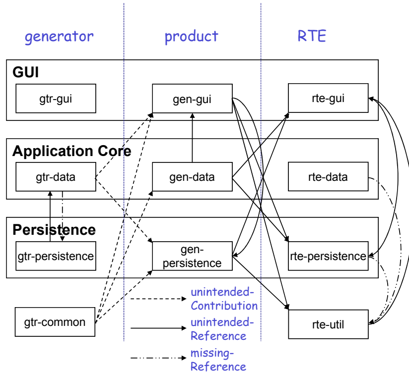
Abbildung 10.9.: Die Differenzarchitektur des DEx-Projekts.
