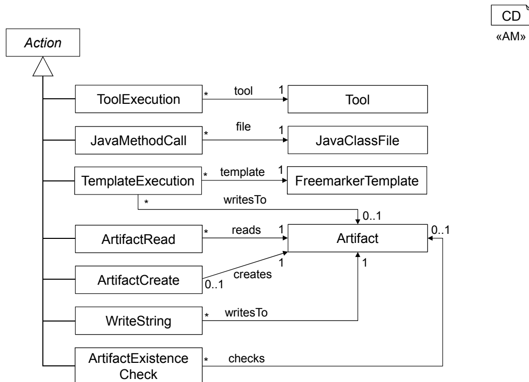
Abbildung 6.24.: Relevante Aktionen des Generierungsprozesses.
