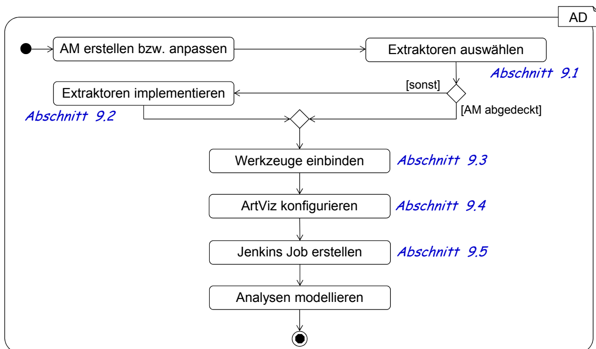
Abbildung 9.1.: Methodik zur Verwendung der MontiArt-Werkzeugkette.
