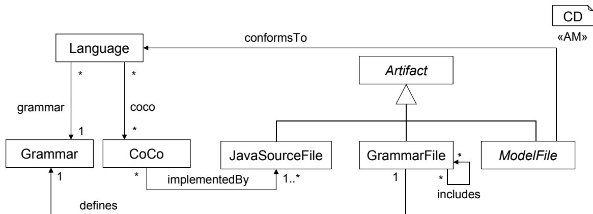
Abbildung 6.11.: Eine Sprache wird durch eine Grammatik und mehrere Wohlformtheitsregeln beschrieben.
