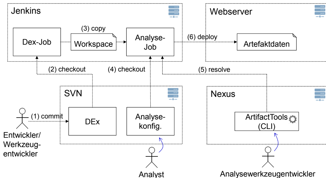
Abbildung 9.13.: Integration der Artefaktdatenanalyse in die bestehende Infrastruktur.
