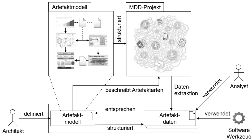
Abbildung 4.2.: Lösungsansatz zur artefaktbasierten Analyse modellgetriebener Softwareentwicklungsprojekte (angepasst aus [BGRW18]).
