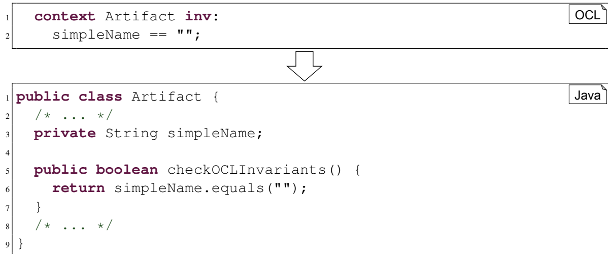
Abbildung 8.28.: Überführung einer OCL-Prüfbedingung in eine Java-Prüfmethode (entnommen aus [Cuj17]).
