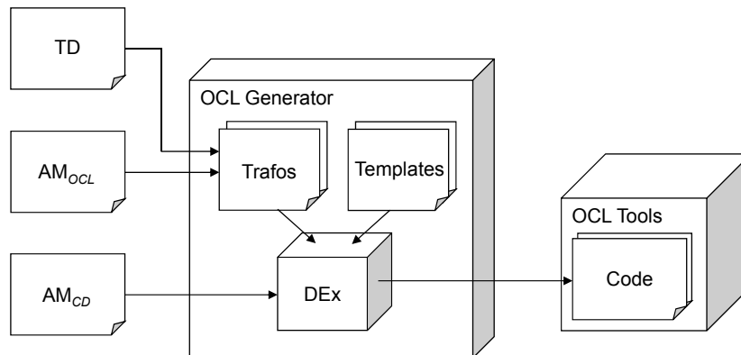
Abbildung 8.23.: Überblick über den Ablauf des OCLGenerator.
