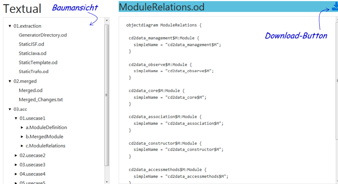
Abbildung 8.36.: Textuelle Darstellung von Artefaktdaten durch die Textansicht von ArtViz.
