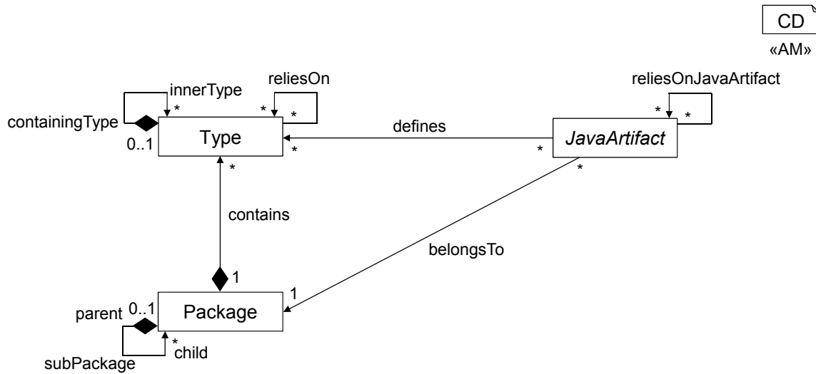
Abbildung 6.7.: Java-Typen und deren Beziehungen.
