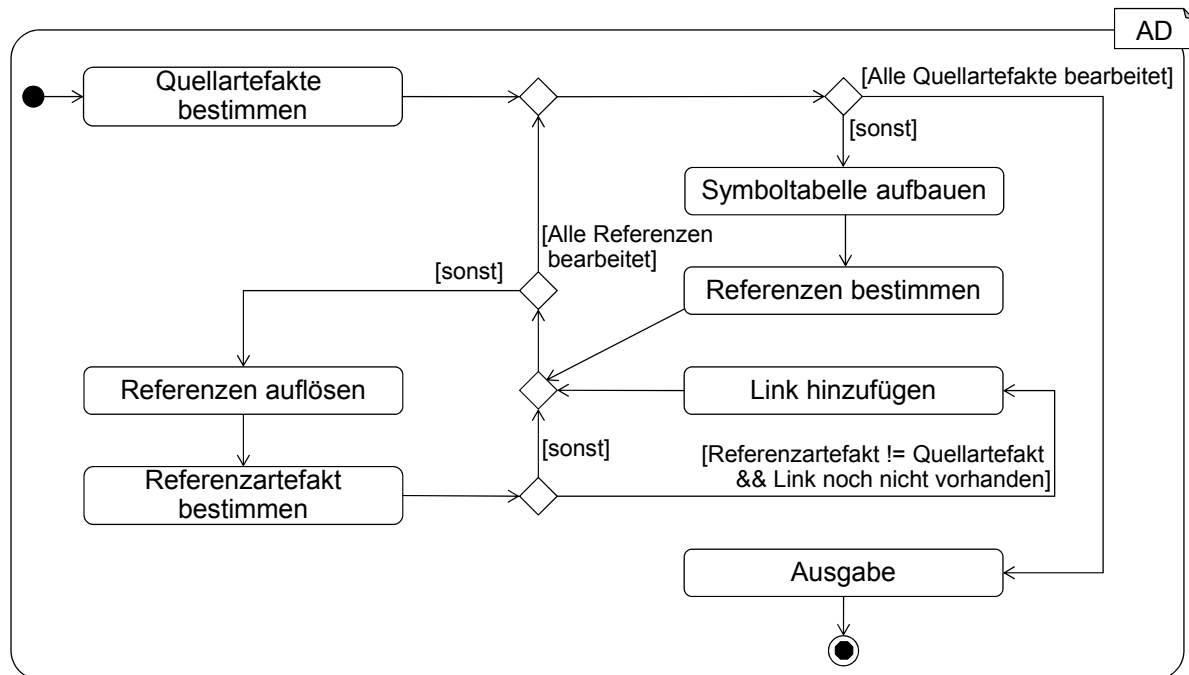
Abbildung 9.2.: Methodik zur Extraktion von Beziehungen zwischen Artefakten mit Hilfe der Symboltabelle.
