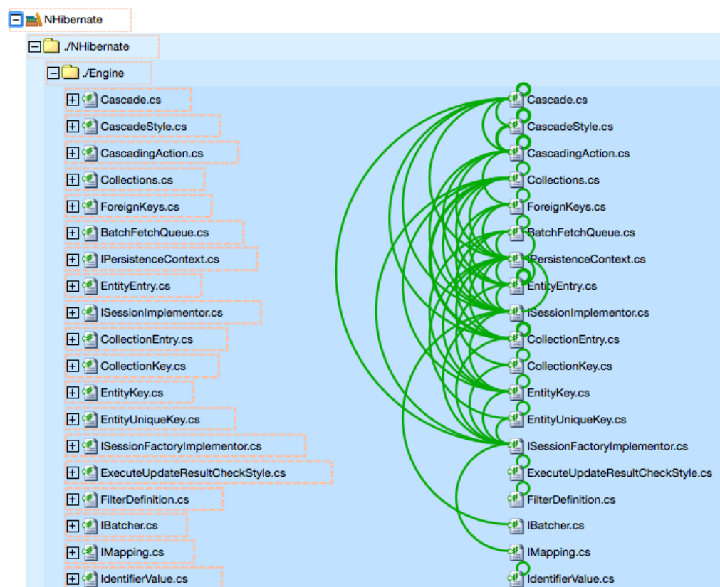
Abbildung 3.7.: Die Exploration View von Sonargraph zur Darstellung von Architekturbeziehungen (entnommen von [Hel17b]).
