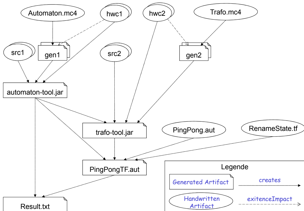
Abbildung 10.24.: Artefaktbeziehungen eines beispielhaften, inkrementellen Generierungsprozesses mit MontiCore.
