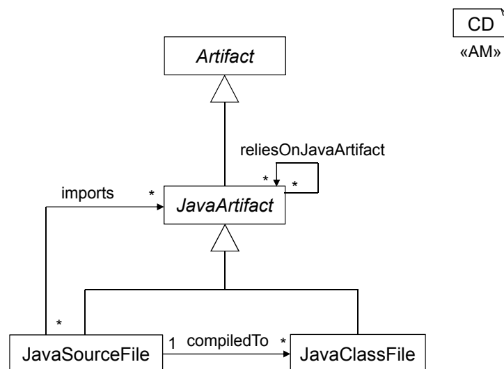
Abbildung 6.1.: Modellierung von Java-Artefakten und zugehörigen Beziehungen.
