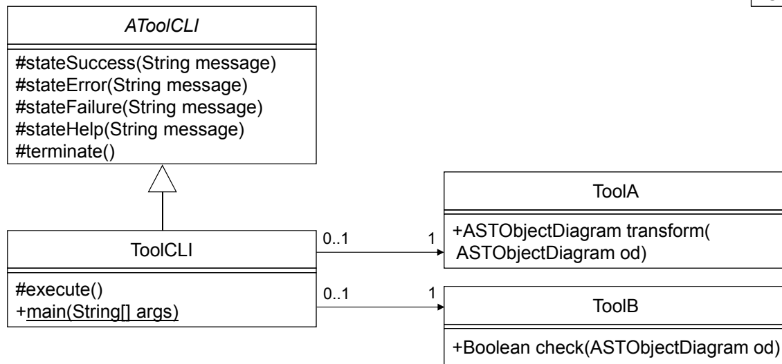
Abbildung 8.5.: Schematische Darstellung der Klassenstruktur für ausführbare Jar-Archive.
