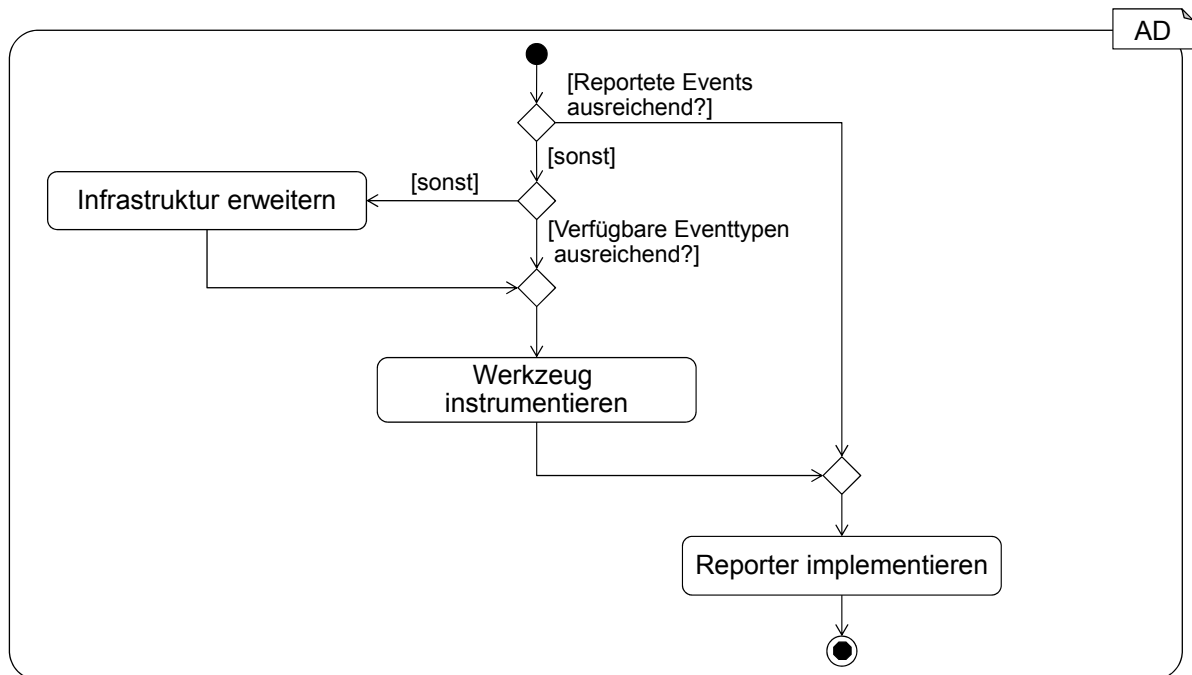
Abbildung 9.4.: Entscheidungshilfe für die Verwendung und Anpassung der Reportinginfrastruktur.
