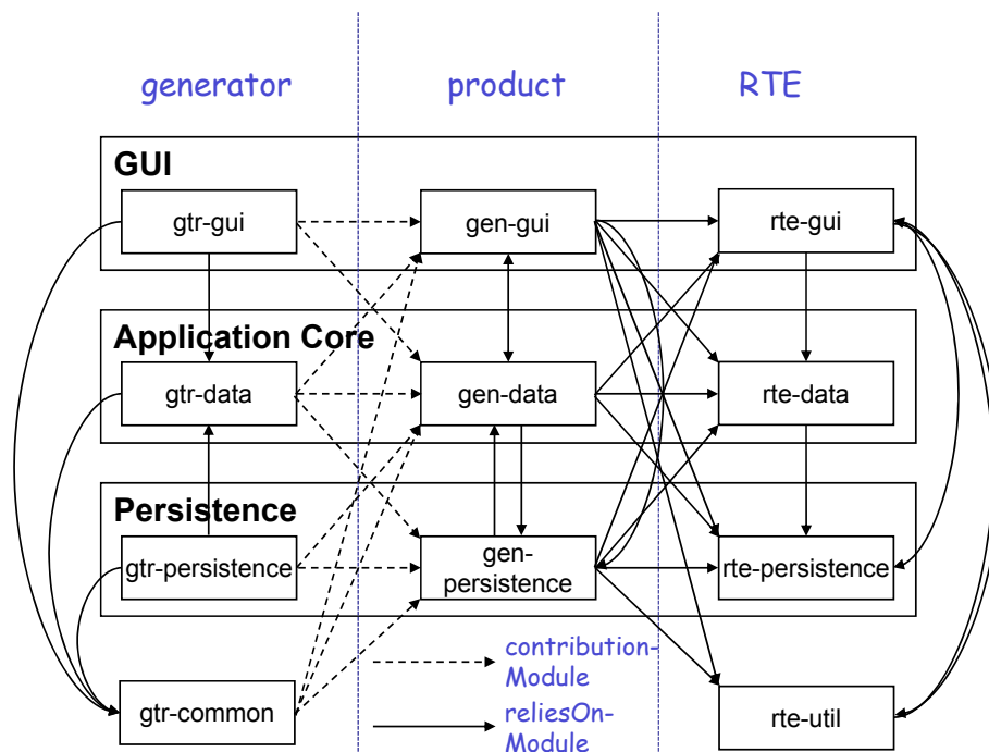
Abbildung 10.8.: Die Ist-Architektur des DEX-Projekts.
