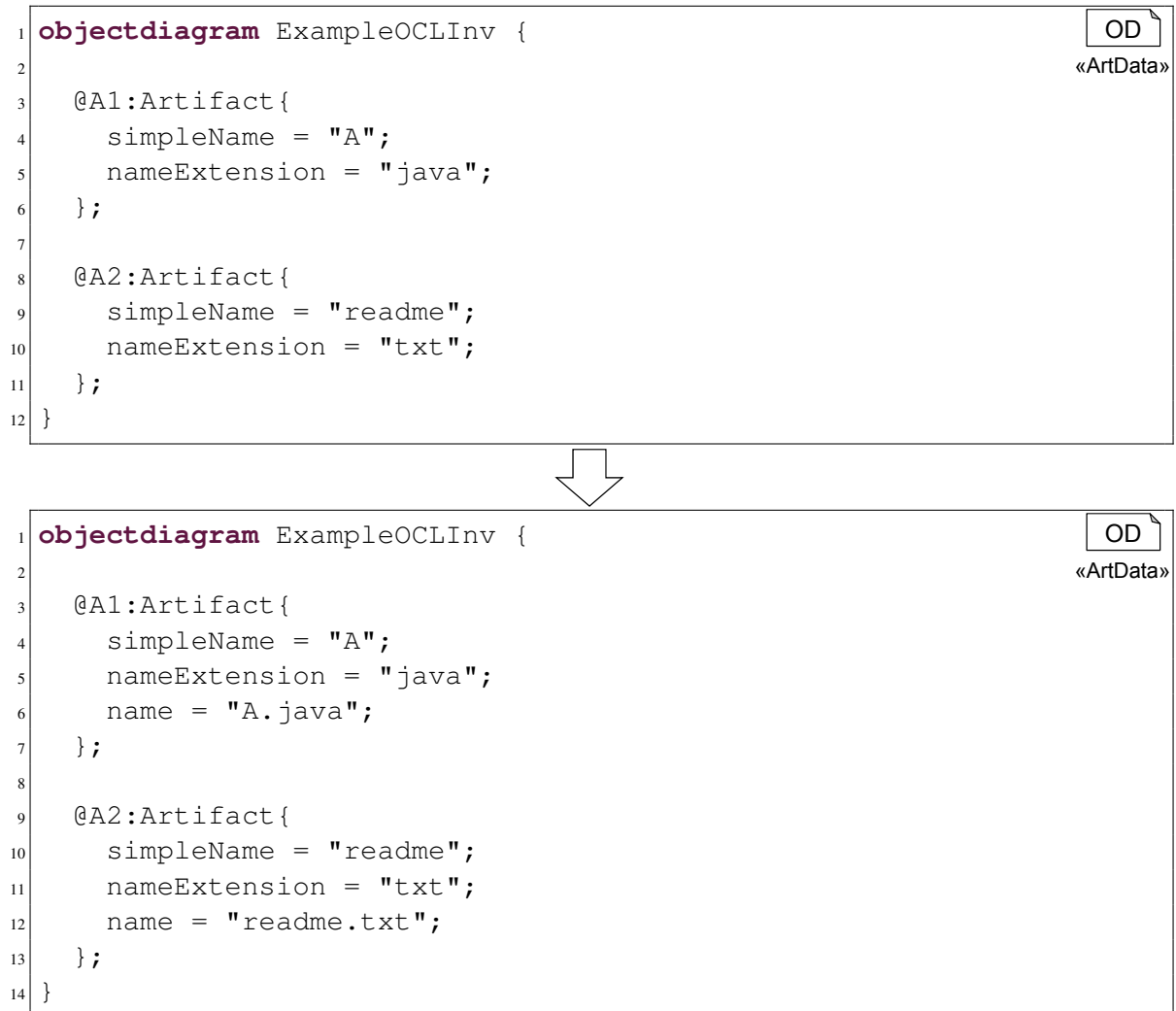
Abbildung 7.16.: Beispielhafte Anreicherung von Artefaktdaten.
