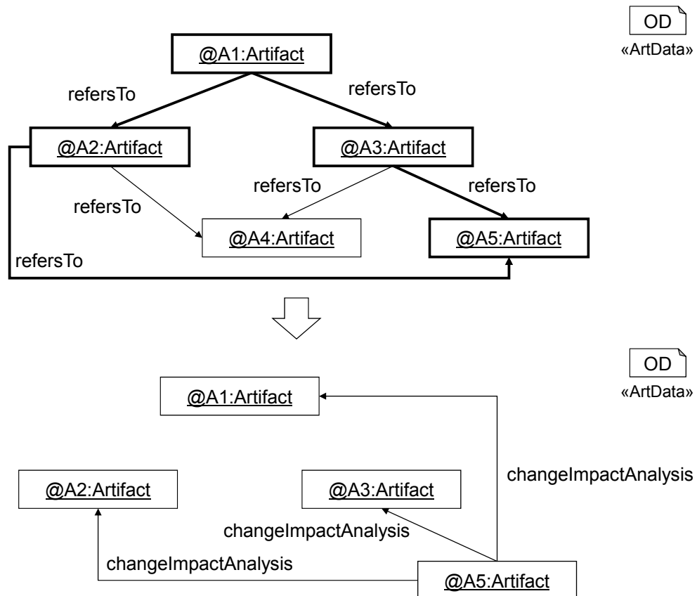
Abbildung 7.17.: Schematische Durchführung einer OCL-basierten Analyse am Beispiel der Change-Impact-Analyse für das Artefakt @A5.
