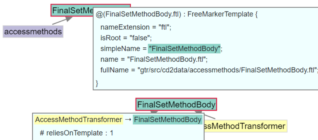
Abbildung 8.38.: Oben: Details eines Knotens; unten: Details einer Kante.
