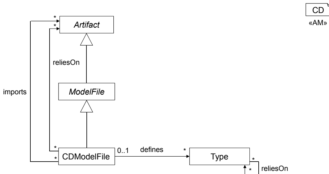
Abbildung 6.16.: CD-Modelldateien, verwandte Elemente und Beziehungen.
