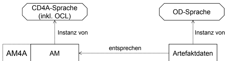
Abbildung 5.1.: Übersicht über den Zusammenhang der verwendeten Sprachen und Modelle bei der Artefaktmodellierung.
