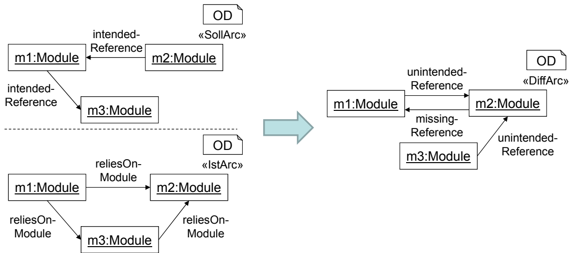
Abbildung 7.20.: Oben links: Soll-Architektur; Unten links: Berechnete Ist-Architektur; Rechts: Berechnete Differenzarchitektur aus Soll- und Ist-Architektur.
