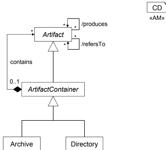
Abbildung 5.2.: Abstrakte Beziehungen zwischen Artefakten und die Organisation von Artefakten in Containern.
