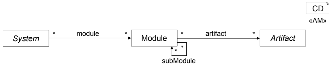
Abbildung 5.12.: Module repräsentieren die architektonische Substruktur des Systems. Sie bestehen aus Artefakten und können sich aus Submodulen zusammensetzen.
