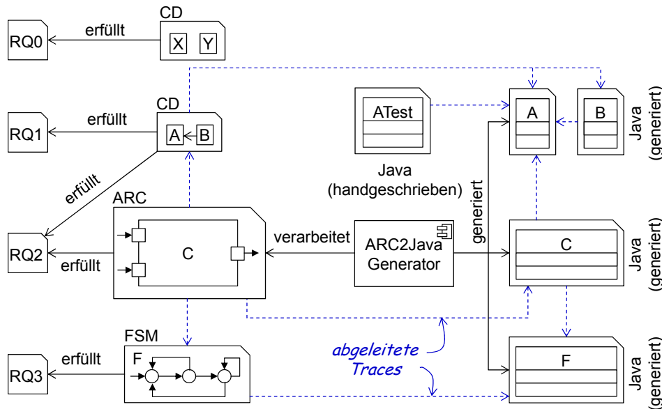
Abbildung 4.1.: Beispielszenario eines Softwareentwicklungsprojekts mit MAA (angepasst aus [BGRW18]).
