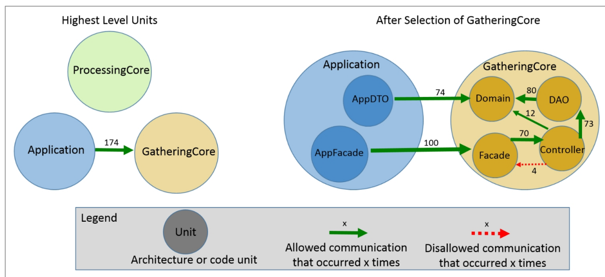
Abbildung 3.6.: Die Circle-based hierarchical view von ARAMIS zur Darstellung von Architekturbeziehungen (entnommen aus [NLG + 15]).
