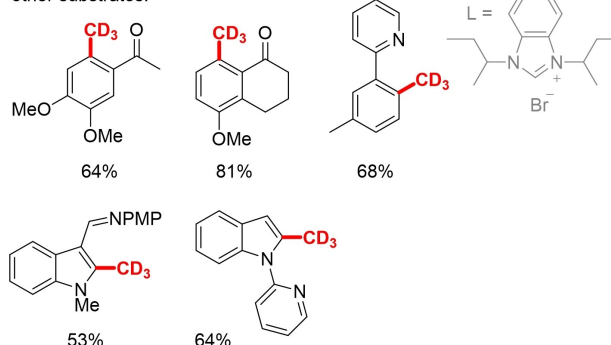
Scheme 23. \text{C-H} Trideuteromethylation strategies with \text{CD}_3\text{OTs} .
