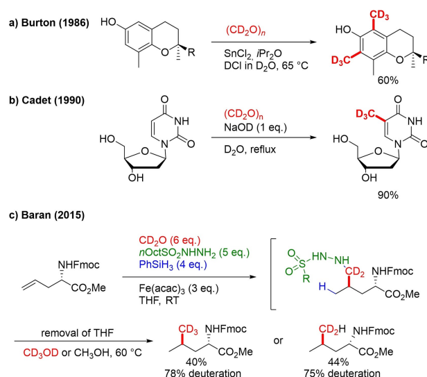
Scheme 29. \text{CD}_2\text{O} -mediated trideuteromethylation.
