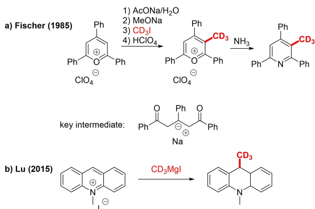
Scheme 10. C–H trideuteromethylation of aromatic salts.
