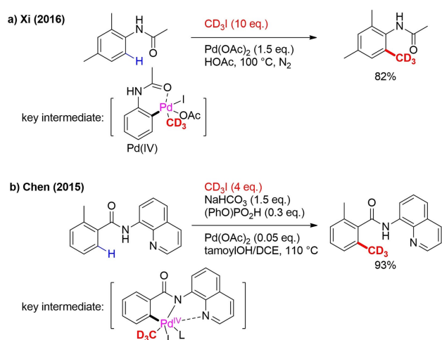
Scheme 9. Pd-catalyzed ortho C–H trideuteromethylation with CD 3 I.
