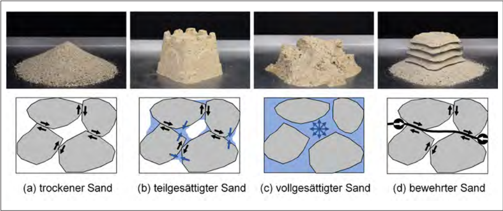
Bild 2: Auswirkung von Wasser im Boden bei einem Sand
