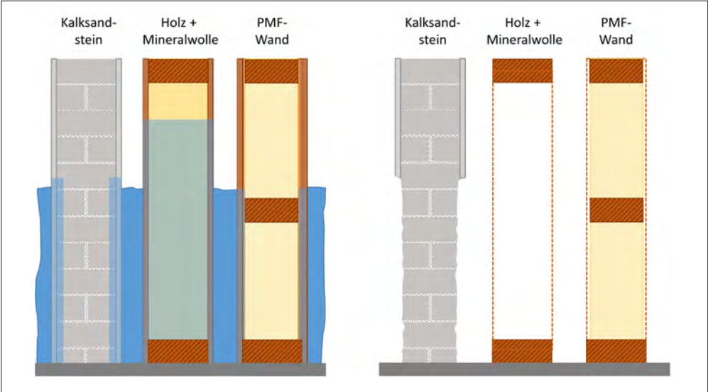
Bild 5: Bauweisen im Vergleich. Links während der Überschwemmung, rechts während der Reparatur. Bei der PMF-Wand wird bei der Reparatur lediglich die Verkleidung entfernt, Holzteile und Schaumkern werden gereinigt und die Holzteile getrocknet. Es muss weder die vollgesogene Isolierung ausgetauscht werden, noch müssen durchnässte Mauersteine behandelt werden.
